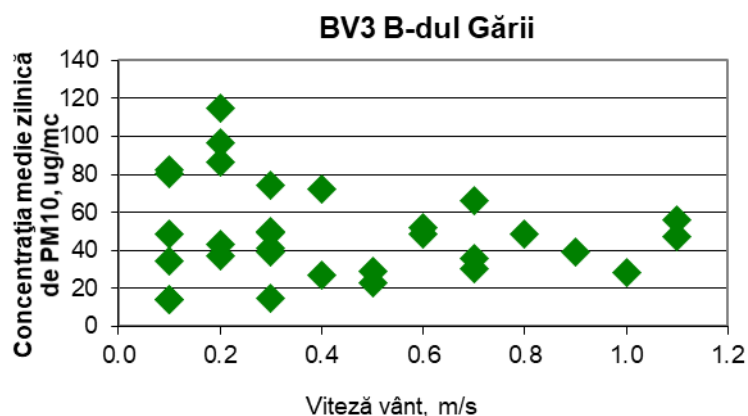
Figura 1.1.2.4.2. Evoluția mediilor zilnice de PM 10 în funcție de viteza vântului la stația BV3
