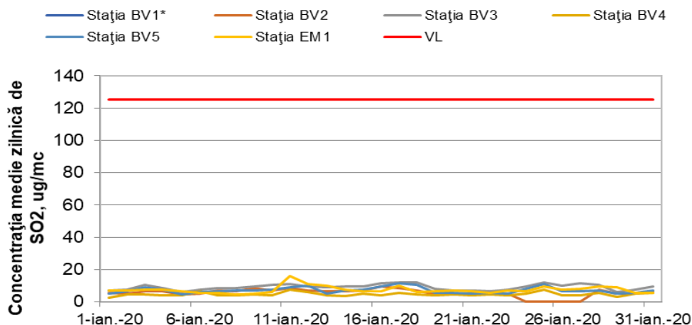
Figura 1.1.2.1.1. Evoluția mediilor zilnice de \text{SO}_2 în luna ianuarie
