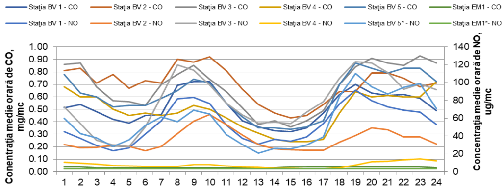
Figura 1.1.2.2.4. Ciclul zilnic al \text{NO} și \text{CO}
