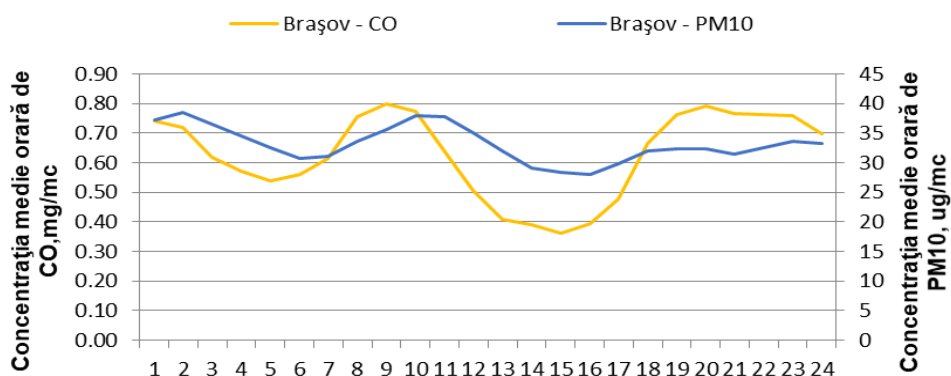
Figura 1.1.2.4.3: Ciclul zilnic al PM10 și CO în Brașov
