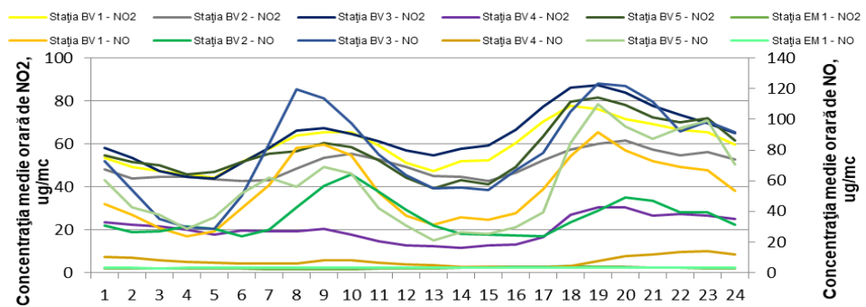
Figura 1.1.2.2.2. Ciclul zilnic al NO 2 și NO
