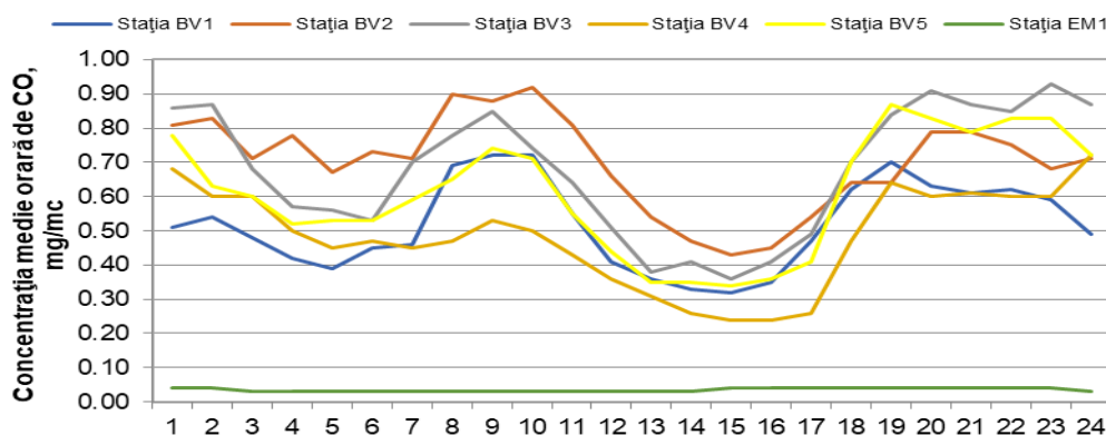
Figura 1.1.2.5.2. Ciclul zilnic al CO
