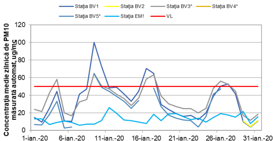
Figura 1.1.2.4.1. Evoluția mediilor zilnice de PM 10 în luna ianuarie
