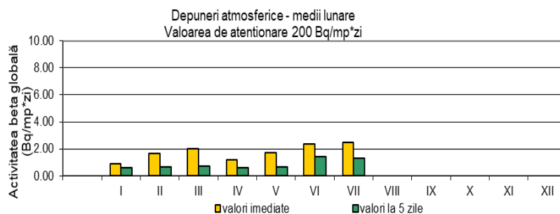
Figura 1.3.4: Activitatea beta globală pentru depuneri atmosferice
