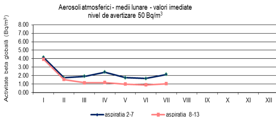
Figura 1.3.1: Activitatea beta globală pentru aerosoli atmosferici
