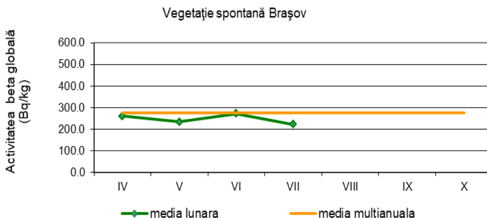
Figura 1.3.9: Activitatea beta globală a probelor de vegetație spontană recoltate din Brașov
