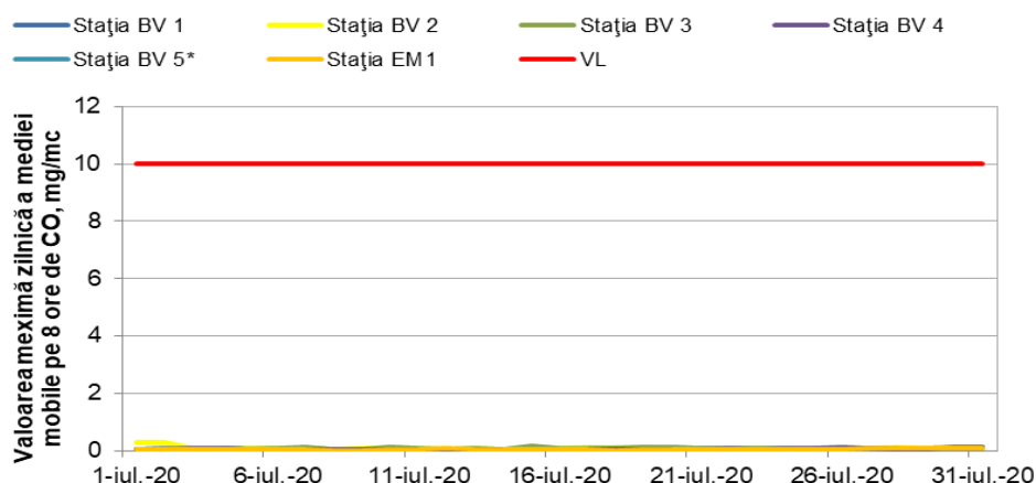
Figura 1.1.2.5.1. Evoluția maximelor zilnice ale mediei mobile de CO în luna iulie
