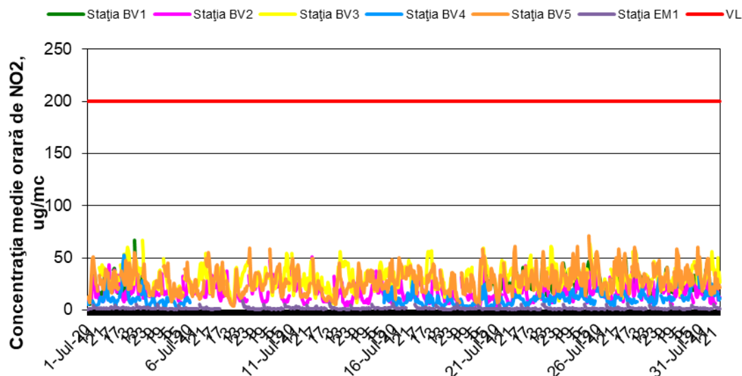
Figura 1.1.2.2.1. Evoluția mediilor orare de NO 2 în luna iulie
