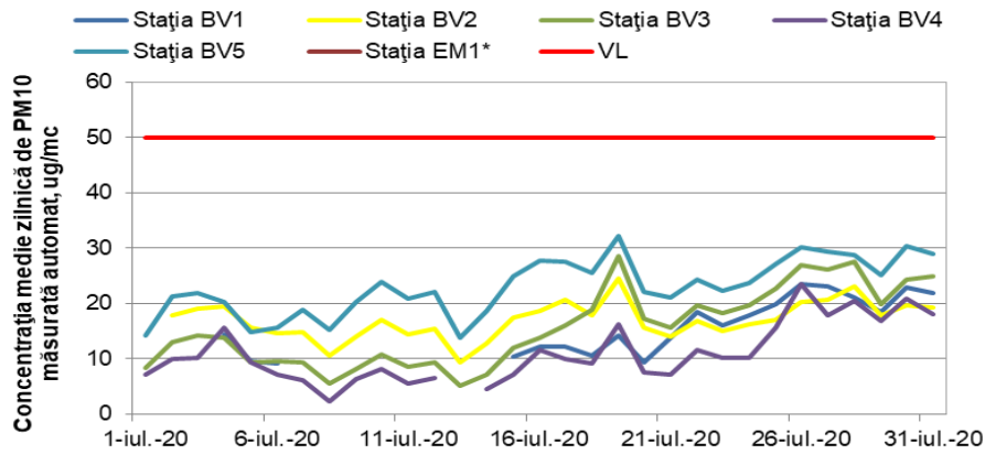
Figura 1.1.2.4.1. Evoluția mediilor zilnice de PM 10 în luna iulie
