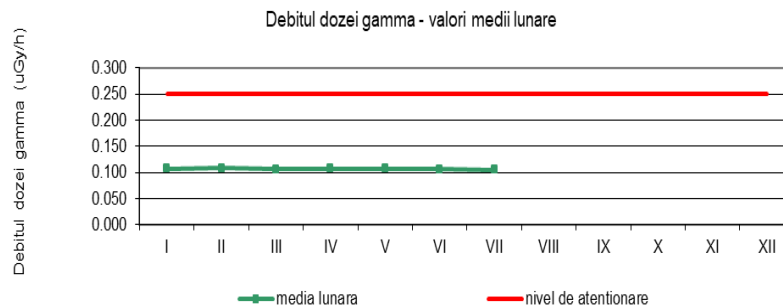
Figura 1.3.3: Debitul dozei gamma în aer
