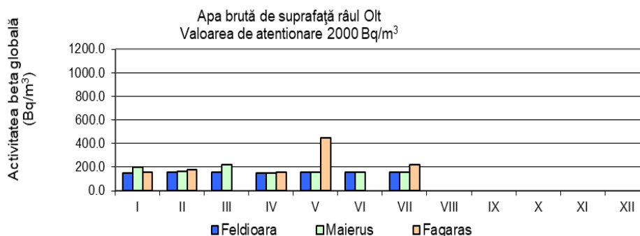
Figura 1.3.7: Activitatea beta globală la 5 zile pentru apa de suprafață Râul Olt
