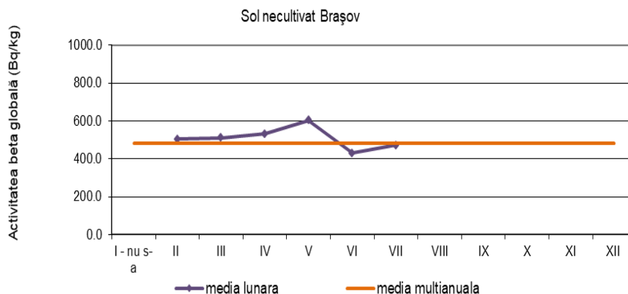
Figura 1.3.8: Activitatea beta globală a probelor de sol necultivat recoltate din Brașov
