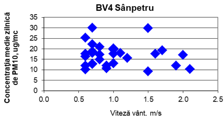
Figura 1.1.2.4.2. Evoluția mediilor zilnice de PM 10 în funcție de viteza vântului
