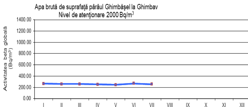
Figura 1.3.5: Activitatea beta globală imediată pentru apa de suprafață Pârâul Ghimbășel
