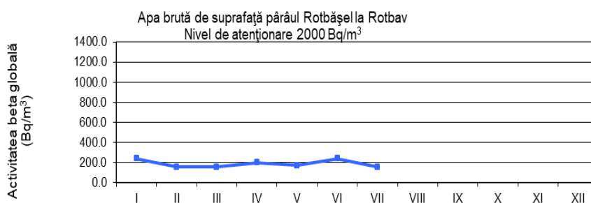
Figura 1.3.6: Activitatea beta globală la 5 zile pentru apa de suprafață-Pârâul Rotbășel
