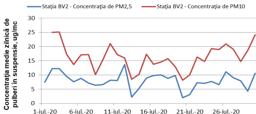
Figura 1.1.2.4.4 Evoluția mediilor zilnice de PM 2,5 și PM10 în luna iulie
