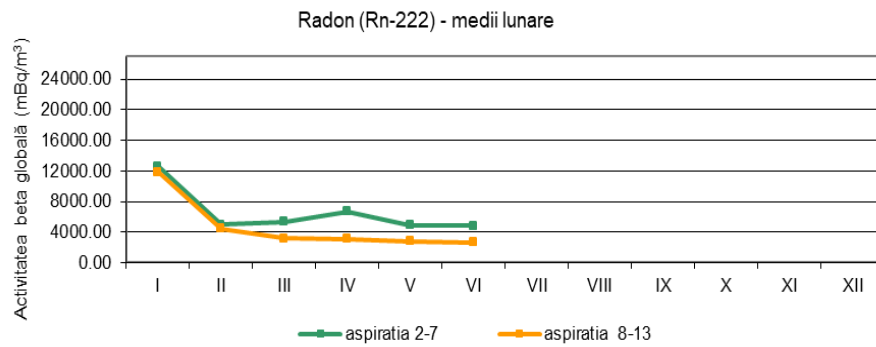
Figura 1.3.2: Activitatea calculată a Radonului
