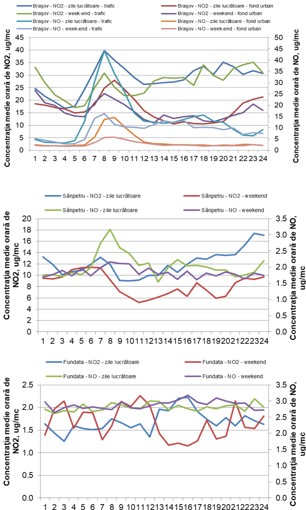
Figura 1.1.2.2.3. Ciclul zilnic al oxizilor de azot în timpul săptămânii
