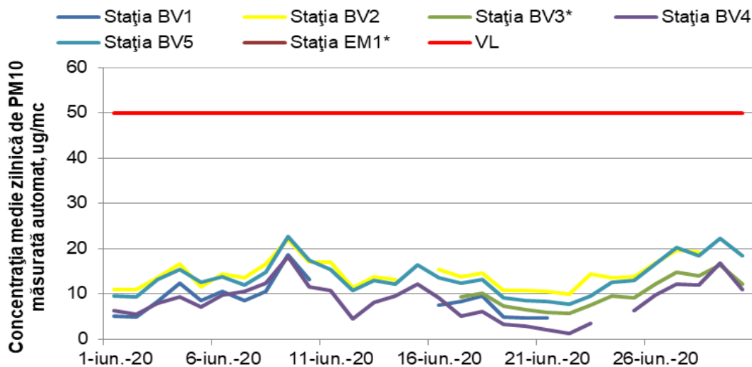
Figura 1.1.2.4.1. Evoluția mediilor zilnice de PM 10 în luna iunie
