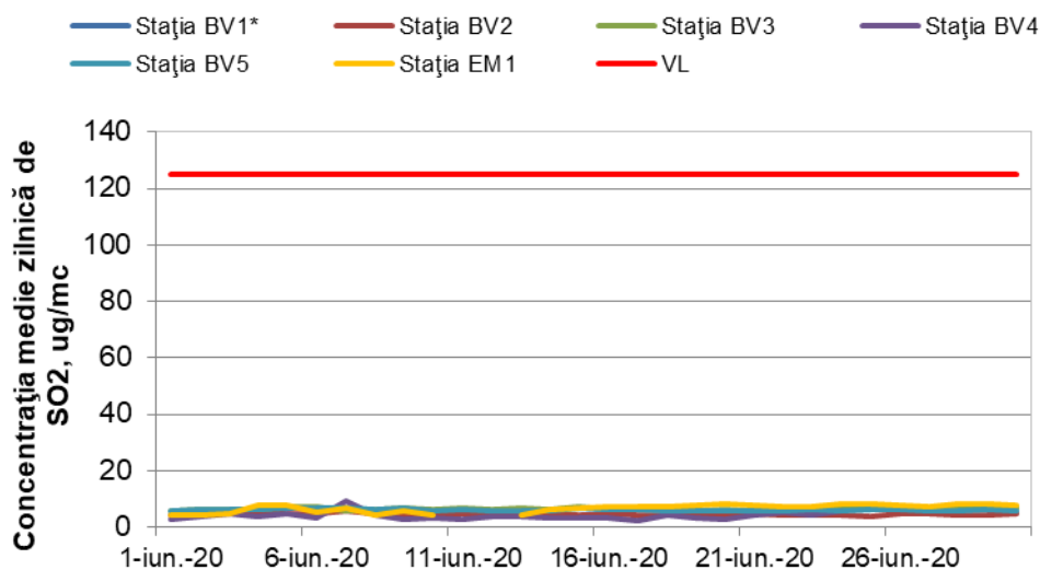
Figura 1.1.2.1.1. Evoluția mediilor zilnice de SO 2 în luna iunie
