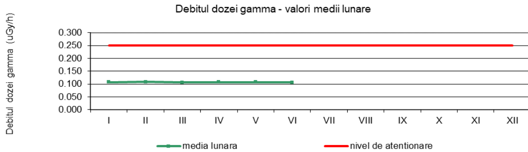
Fig. 1.3.3. Debitul dozei gamma în aer
