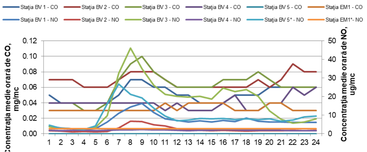
Figura 1.1.2.2.4. Ciclu zilnic al NO și CO
