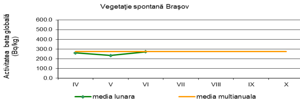
Fig. 1.3.9. Activitatea beta globală la 5 zile pentru solul necultivat
