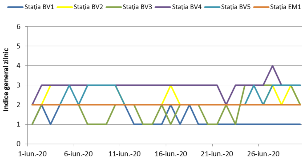
Figura 1.1.2.7.1. Indicele general zilnic de calitate a aerului
