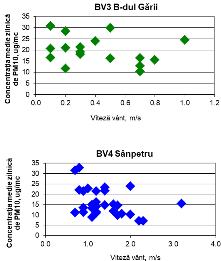
Figura 1.1.2.4.2. Evoluția mediilor zilnice de PM 10 în funcție de viteza vântului
