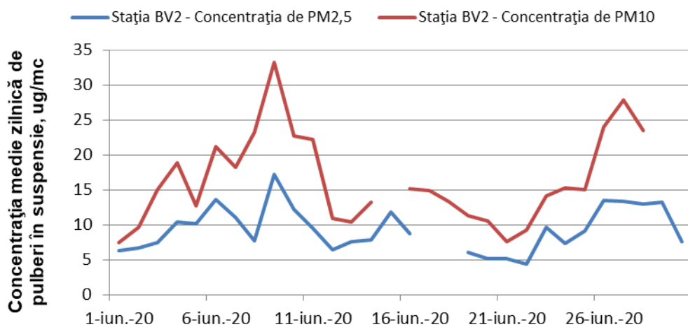
Figura 1.1.2.4.4 Evoluția mediilor zilnice de PM 2,5 și PM10 în luna iunie
