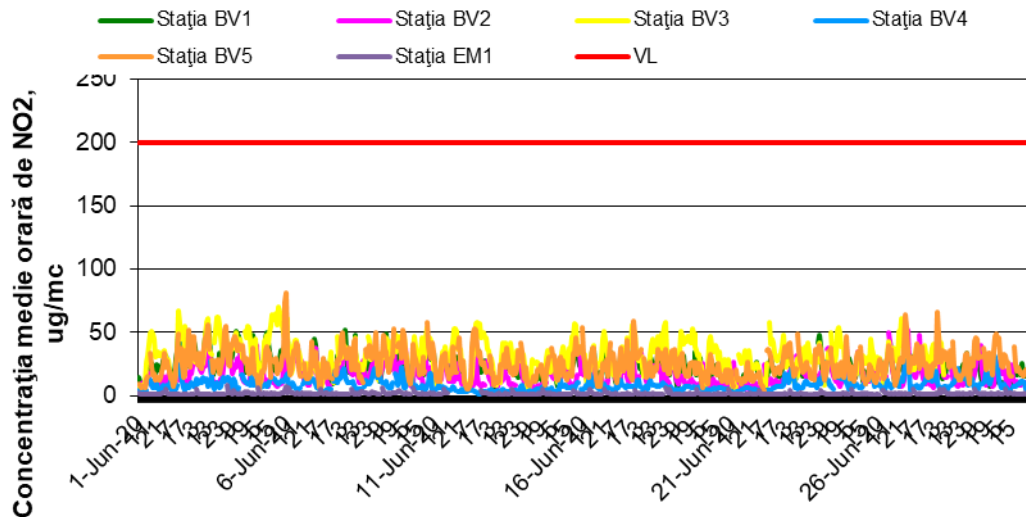
Figura 1.1.2.2.1. Evoluția mediilor orare de \text{NO}_2 în luna iunie
