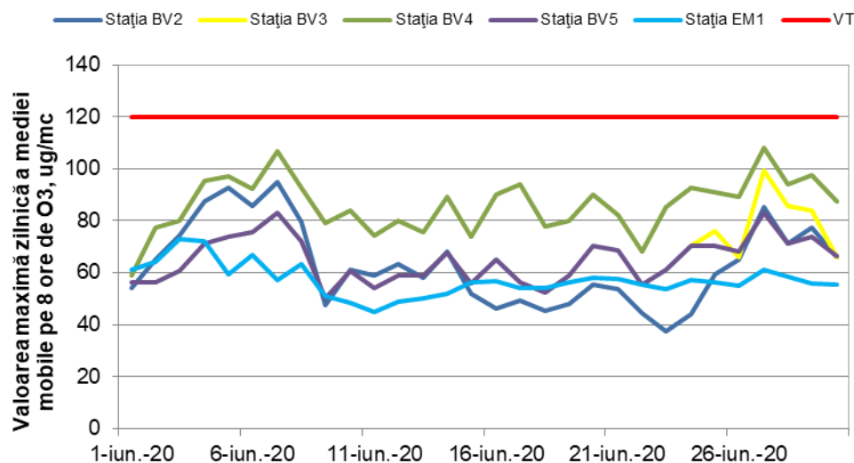
Figura 1.1.2.3.1. Evoluția maximelor zilnice ale mediilor mobile pe 8 ore de O 3 în luna iunie
