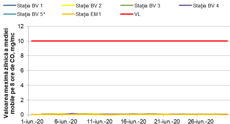
Figura 1.1.2.5.1. Evoluția maximelor zilnice ale mediei mobile de CO în luna iunie
