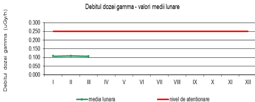
Fig. 1.3.3. Debitul dozei gamma în aer
