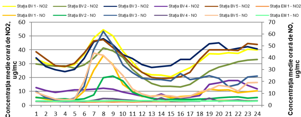
Figura 1.1.2.2.2. Ciclul zilnic al \text{NO}_2 și NO
