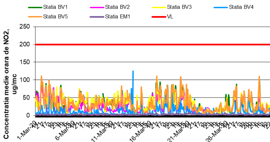
Figura 1.1.2.2.1. Evoluția mediilor orare de \text{NO}_2 în luna martie
