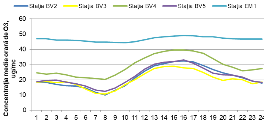
Figura 1.1.2.3.2. Ciclul zilnic al ozonului
