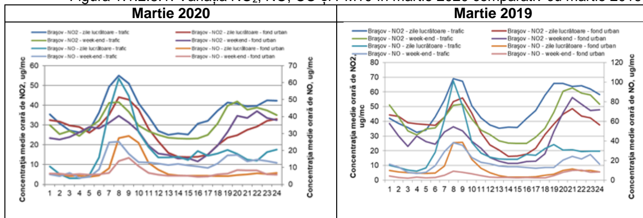
Figura 1.1.2.8.1. Variația NO 2 , NO, CO și PM10 în martie 2020 comparativ cu martie 2019
