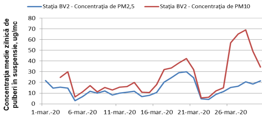
Figura 1.1.2.4.4 Evoluția mediilor zilnice de PM 2,5 și PM10 în luna martie
