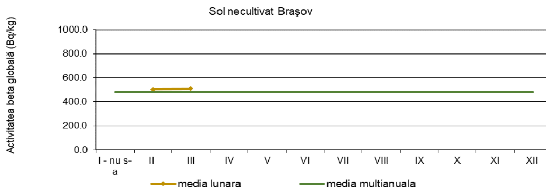
Fig. 1.3.8. Activitatea beta globală la 5 zile a solului necultivat
