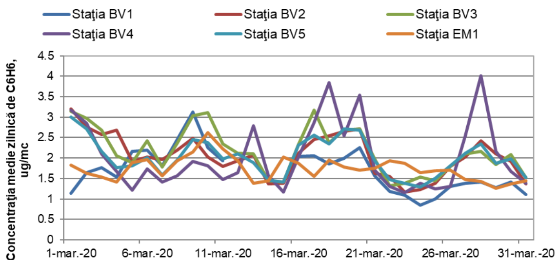
Figura 1.1.2.6.1: Evoluția mediilor zilnice de benzen în luna martie
