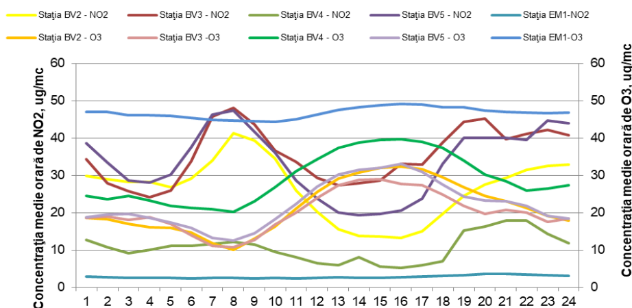
Figura 1.1.2.3.3. Ciclul zilnic al O_3 și NO_2
