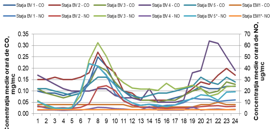
Figura 1.1.2.2.4. Ciclul zilnic al NO și CO
