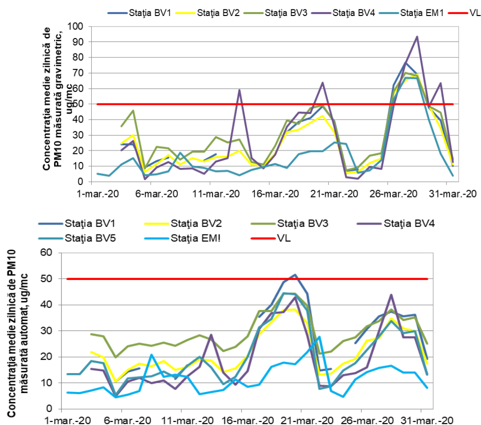
Figura 1.1.2.4.1. Evoluția mediilor zilnice de PM 10 în luna martie
