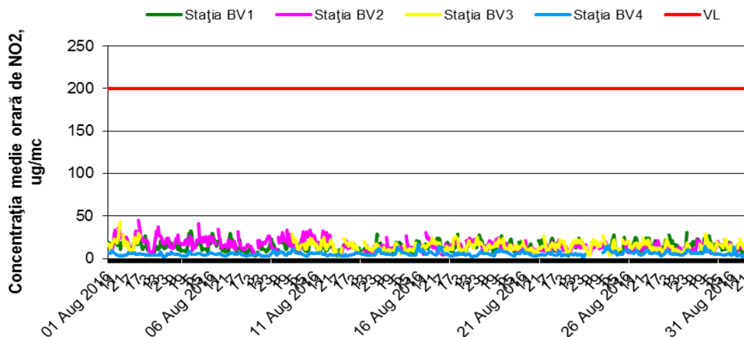
Figura 1.1.2.2.1. Evoluția mediilor orare de \text{NO}_2 în luna august
