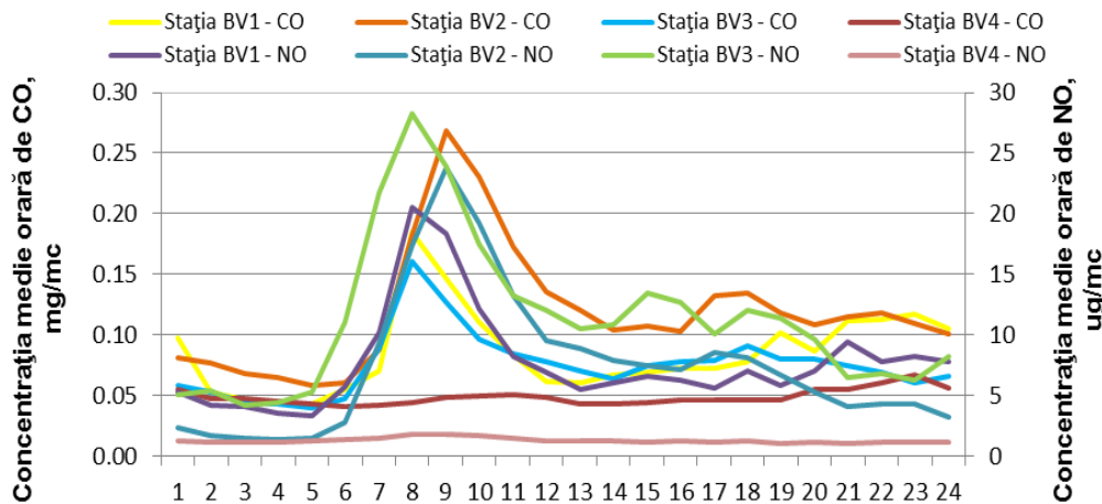
Figura 1.1.2.2.4. Ciclul zilnic al NO și CO
