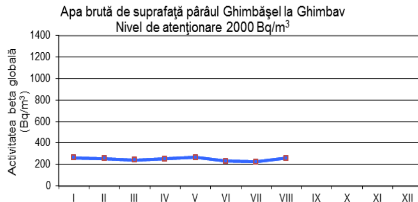
Fig. 1.4.5. Activitatea beta globală imediată pentru apa de suprafață Pârâul Ghimbășel
