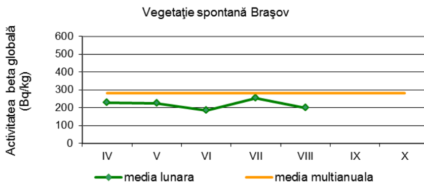
Fig. 1.4.9. Activitatea beta globală a vegetației spontane
