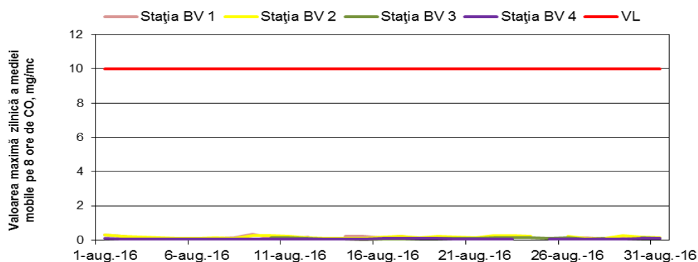
Figura 1.1.2.5.1. Evoluția maximelor zilnice ale mediei mobile de CO în luna august
