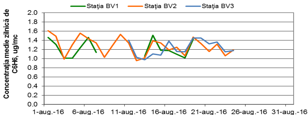
Figura 1.1.2.6.1: Evoluția mediilor zilnice de benzen în luna august
