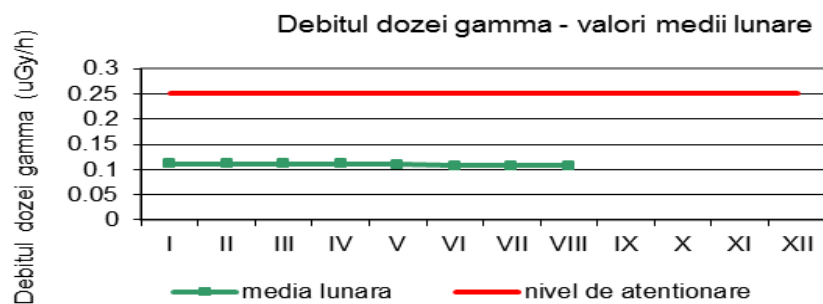
Fig. 1.4.3. Debitul dozei gamma în aer
