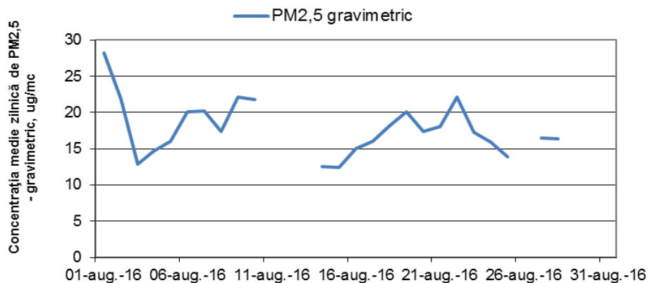
Figura 1.1.2.4.4 Evoluția mediilor zilnice de PM 2,5 în luna august
