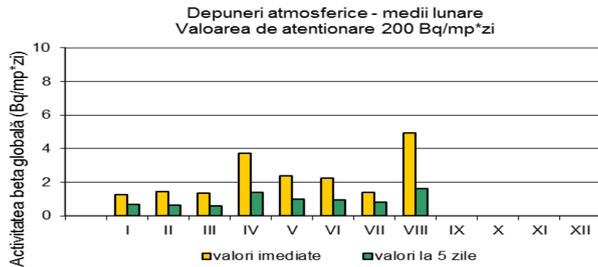
Fig. 1.4.4. Activitatea beta globală pentru depuneri atmosferice
