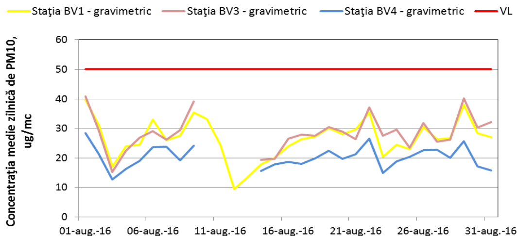
Figura 1.1.2.4.1. Evoluția mediilor zilnice de PM 10 în luna august
