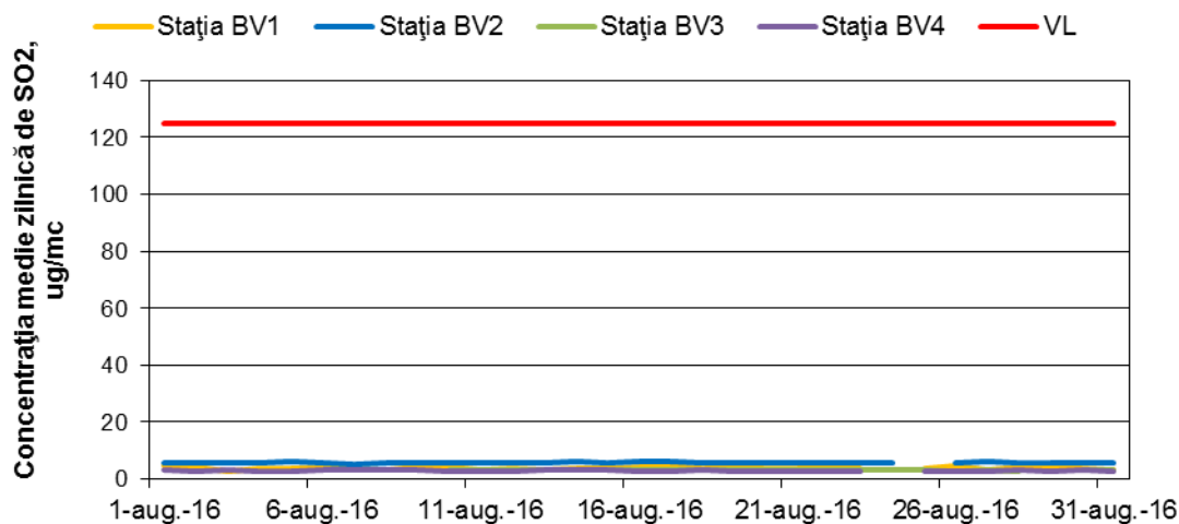
Figura 1.1.2.1.1. Evoluția mediilor zilnice de \text{SO}_2 în luna august
