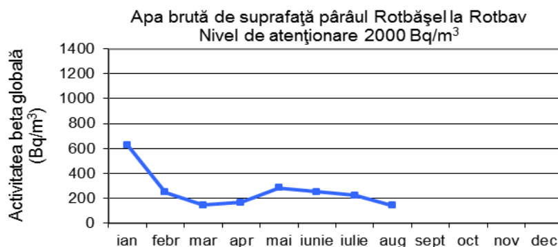
Fig. 1.4.6. Activitatea beta globală la 5 zile pentru apa de suprafață Pârâul Rotbășel
