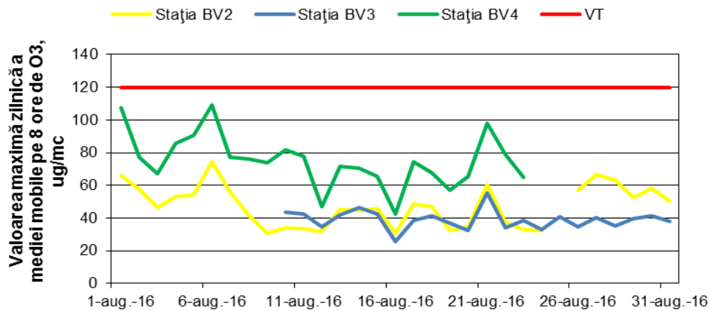
Figura 1.1.2.3.1. Evoluția maximelor zilnice ale mediilor mobile pe 8 ore de O 3 în luna august
