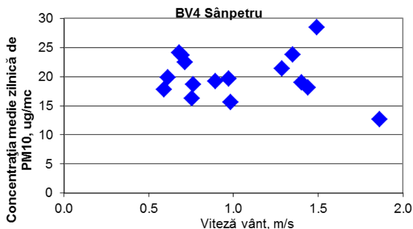
Figura 1.1.2.4.3. Evoluția mediilor zilnice de PM 10 în funcție de viteza vântului la stația BV4
