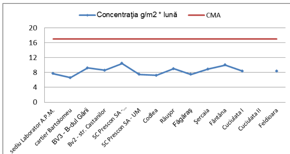
Figura 1.1.1.2. Cantitatea de pulberi sedimentabile în județul Brașov
