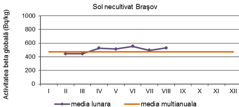
Fig. 1.4.8. Activitatea beta globală a solului necultivat
