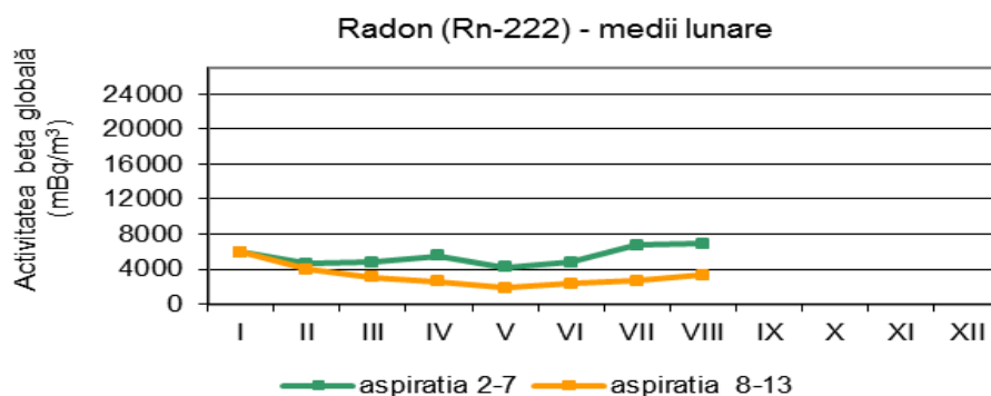
Fig. 1.4.2. Activitatea calculată a Radonului
