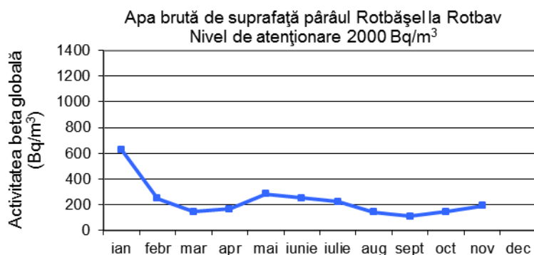
Fig. 1.4.6. Activitatea beta globală –la 5 zile-pentru apa de suprafață-Pârâu Rotbășel
