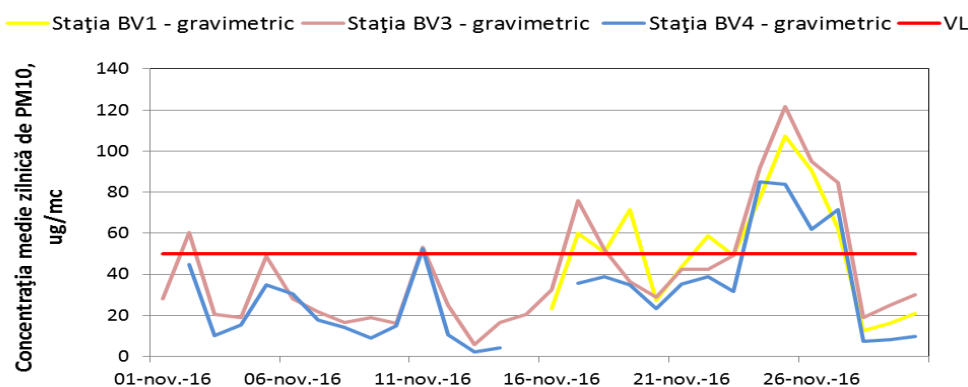
Figura 1.1.2.4.1. Evoluția mediilor zilnice de PM 10 în luna noiembrie
