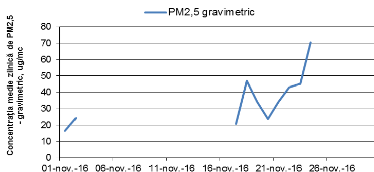
Figura 1.1.2.4.4 Evoluția mediilor zilnice de PM 2,5 în luna noiembrie
