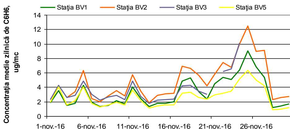
Figura 1.1.2.6.1: Evoluția mediilor zilnice de benzen în luna noiembrie
