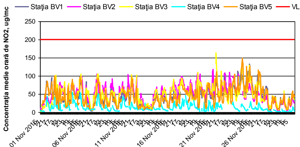
Figura 1.1.2.2.1. Evoluția mediilor orare de \text{NO}_2 în luna noiembrie
