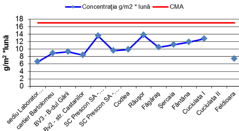
Figura 1.1.1.2. Cantitatea de pulberi sedimentabile în județul Brașov
