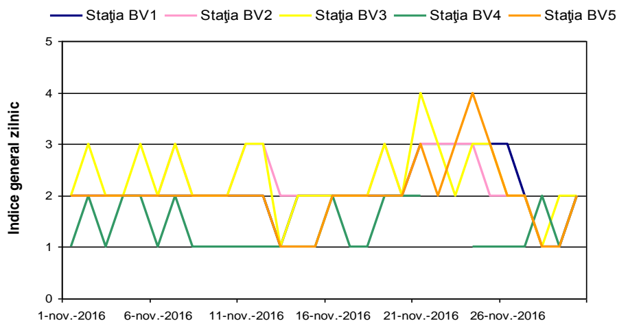
Figura 1.1.2.7.1. Indicele general zilnic de calitatea aerului
