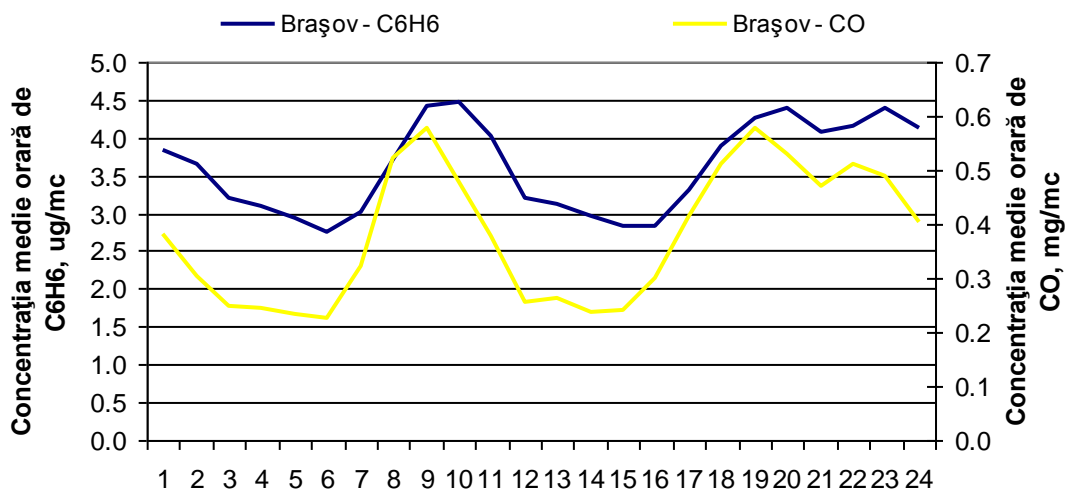
Figura 1.1.2.6.2: Ciclu zilnic al CO și benzenului în Brașov
