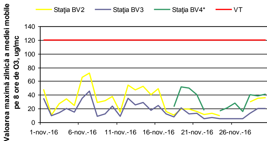
Figura 1.1.2.3.1. Evoluția maximelor zilnice ale mediilor mobile pe 8 ore de O 3 în luna noiembrie
