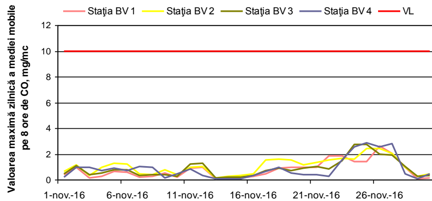
Figura 1.1.2.5.1. Evoluția maximelor zilnice ale mediei mobile de CO în luna noiembrie
