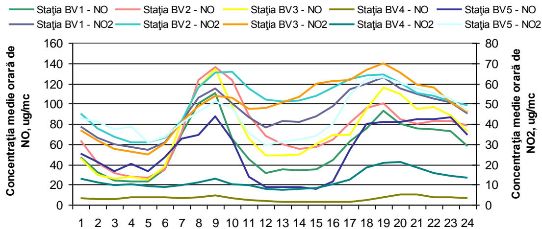
Figura 1.1.2.2.2. Ciclul zilnic al NO 2 și NO
