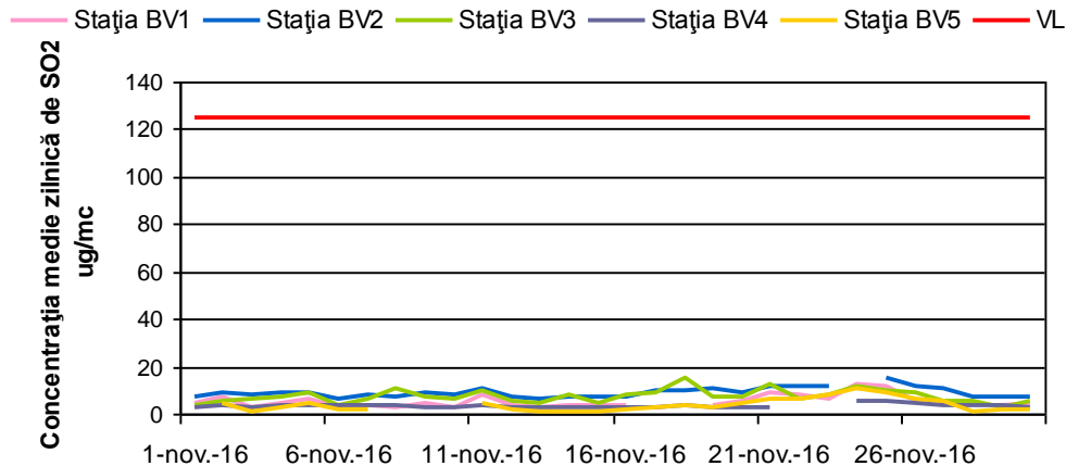
Figura 1.1.2.1.1. Evoluția mediilor zilnice de \text{SO}_2 în luna noiembrie
