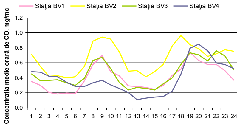
Figura 1.1.2.5.2. Ciclul zilnic al CO
