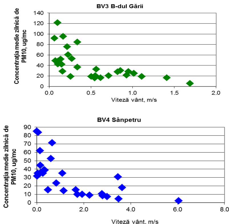
Figura 1.1.2.4.3. Evoluția mediilor zilnice de PM 10 în funcție de viteza vântului la stațiile BV3 și BV4
