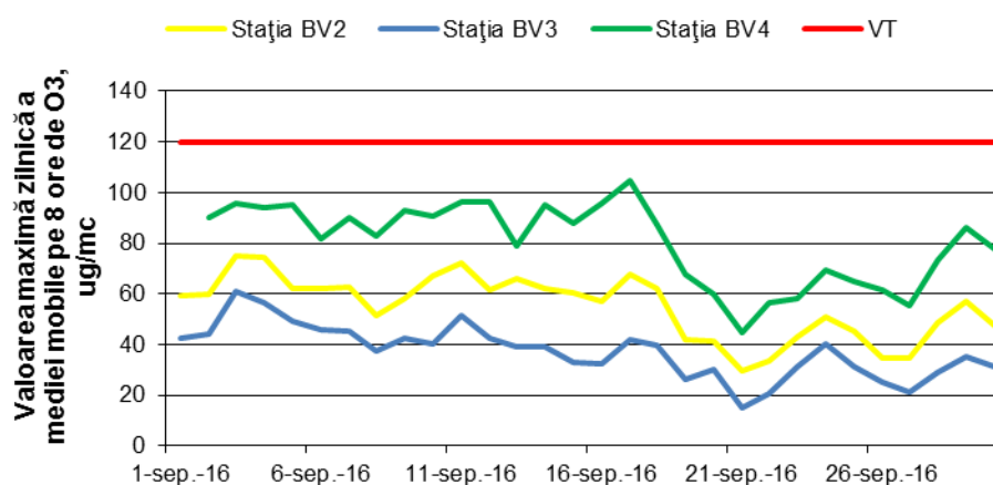
Figura 1.1.2.3.1. Evoluția maximelor zilnice ale mediilor mobile pe 8 ore de O 3 în luna septembrie
