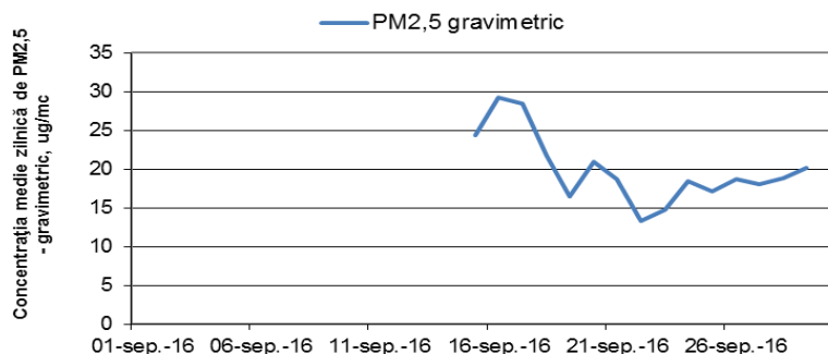
Figura 1.1.2.4.4 Evoluția mediilor zilnice de PM 2,5 în luna septembrie
