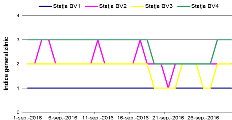
Figura 1.1.2.7.1. Indicele general zilnic de calitatea aerului
