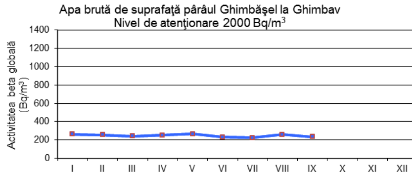
Fig. 1.4.5. Activitatea beta globală imediată pentru apa de suprafață Pârâu Ghimbășel
