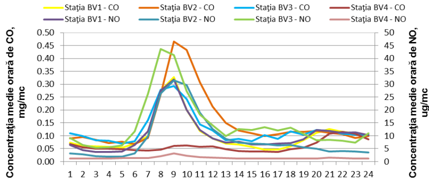
Figura 1.1.2.2.4. Ciclul zilnic al NO și CO
