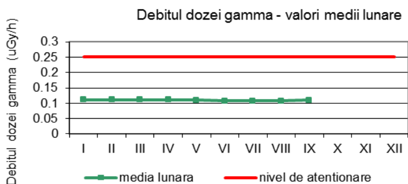
Fig. 1.4.3. Debitul dozei gamma în aer
