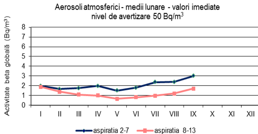
Fig. 1.4.1. Activitatea beta globală pentru aerosoli atmosferici
