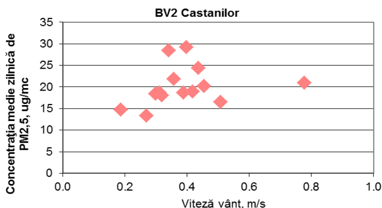
Figura 1.1.2.4.5. Evoluția mediilor zilnice de PM2,5 în funcție de viteza vântului la BV2
