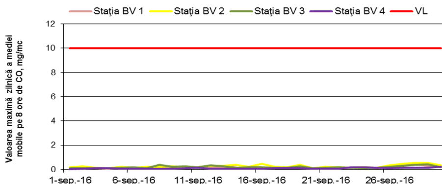
Figura 1.1.2.5.1. Evoluția maximelor zilnice ale mediei mobile de CO în luna septembrie
