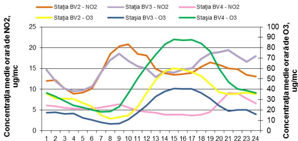
Figura 1.1.2.3.3. Ciclul zilnic al \text{O}_3 și \text{NO}_2
