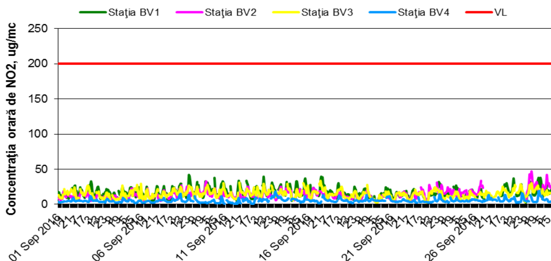
Figura 1.1.2.2.1. Evoluția mediilor orare de \text{NO}_2 în luna septembrie
