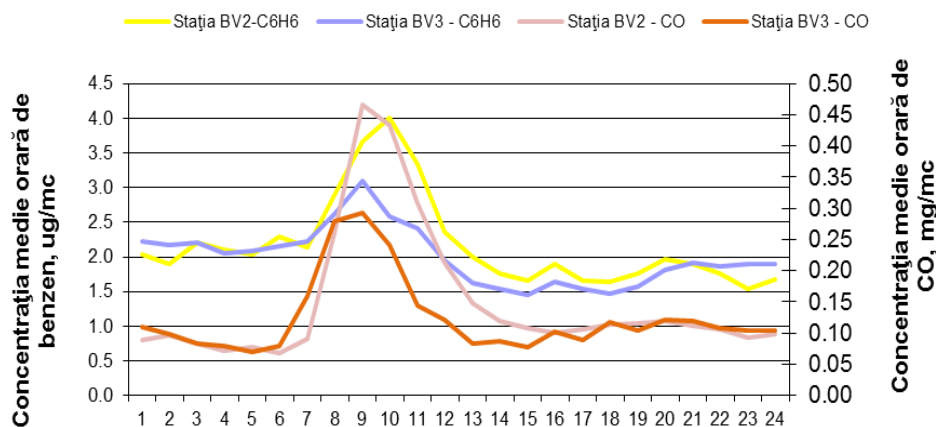
Figura 1.1.2.6.2: Ciclul zilnic al CO și benzenului
