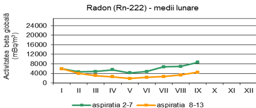
Fig. 1.4.2. Activitatea calculată a Radonului
