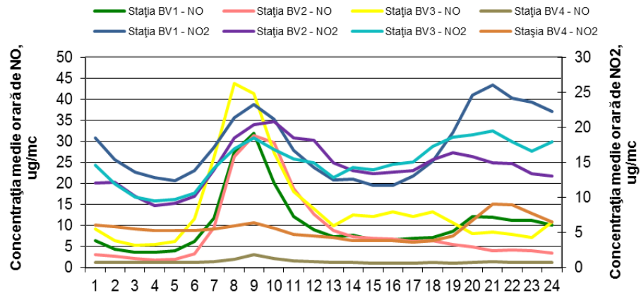
Figura 1.1.2.2.2. Ciclul zilnic al NO 2 și NO
