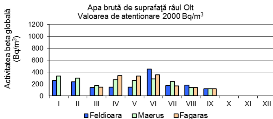
Fig. 1.4.7. Activitatea beta globală –la 5 zile-pentru apa de suprafață Râul OLT
