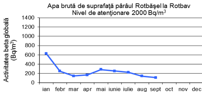
Fig. 1.4.6. Activitatea beta globală –la 5 zile-pentru apa de suprafață-Pârâu Rotbășel
