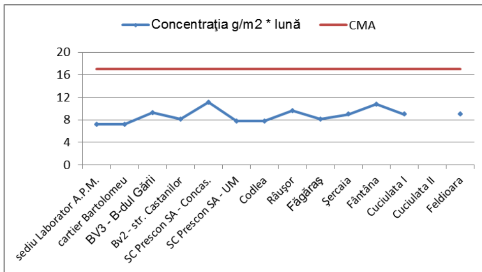
Figura 1.1.1.2. Cantitatea de pulberi sedimentabile în județul Brașov
