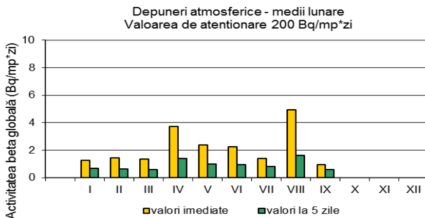
Fig. 1.4.4. Activitatea beta globală pentru depuneri atmosferice
