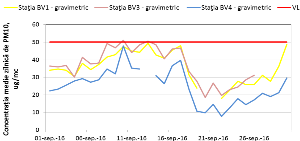
Figura 1.1.2.4.1. Evoluția mediilor zilnice de PM 10 în luna septembrie
