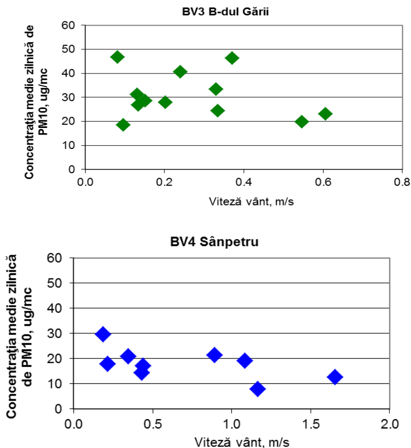
Figura 1.1.2.4.3. Evoluția mediilor zilnice de PM 10 în funcție de viteza vântului la stația BV4
