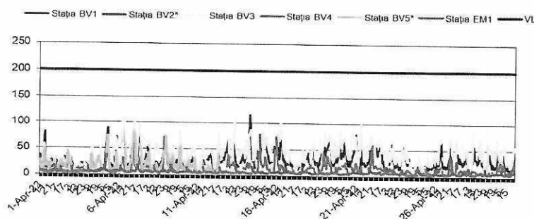
Figura 1.1.2.2.1. Evoluția mediilor orare de NO 2 în luna aprilie
