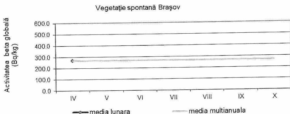
Fig. 1.2.9. Activitatea beta globală la 5 zile pentru vegetația spontană
