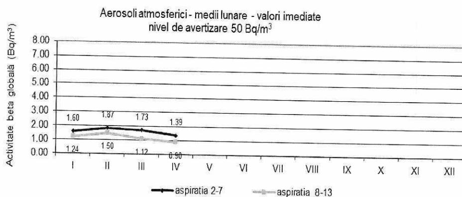
Fig. 1.2.1. Activitatea beta globală pentru aerosoli atmosferici
