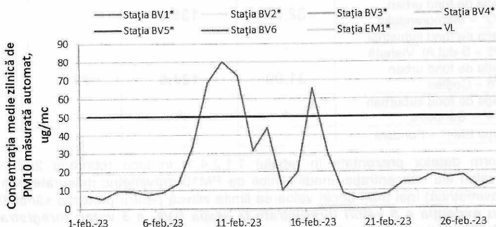
Figura 1.1.2.4.3. Evoluția mediilor zilnice de PM 10, metoda automată, în luna februarie
