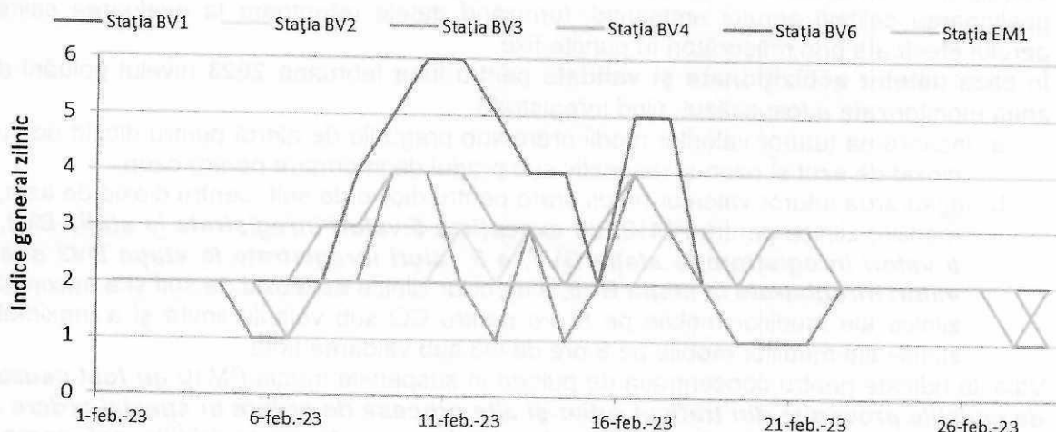
Figura 1.1.2.7.1: Evoluția indicelui general de calitate a aerului din rețeaua locală de monitorizare a calității aerului
