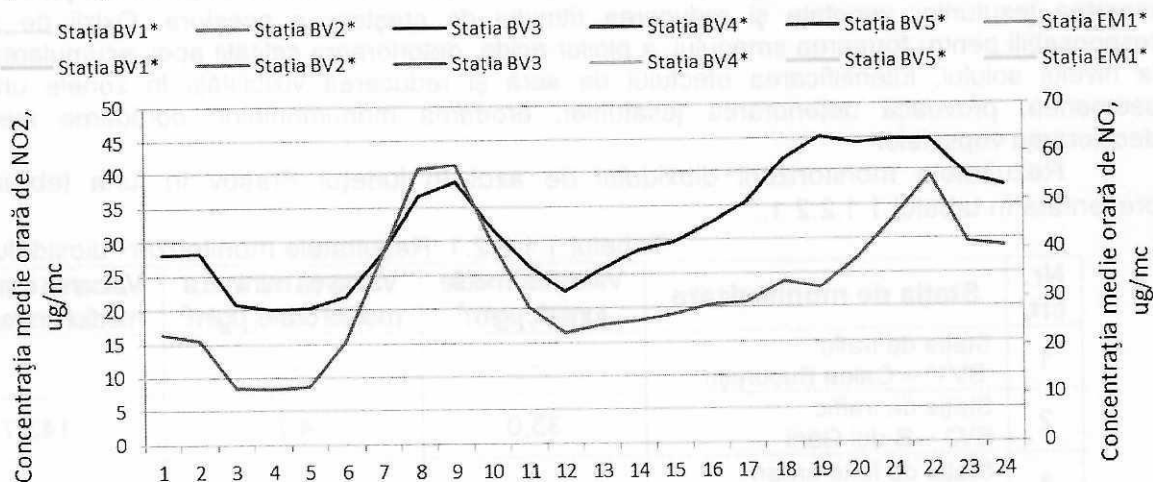
Figura 1.1.2.2.2. Ciclul zilnic al \text{NO}_2 și \text{NO}
