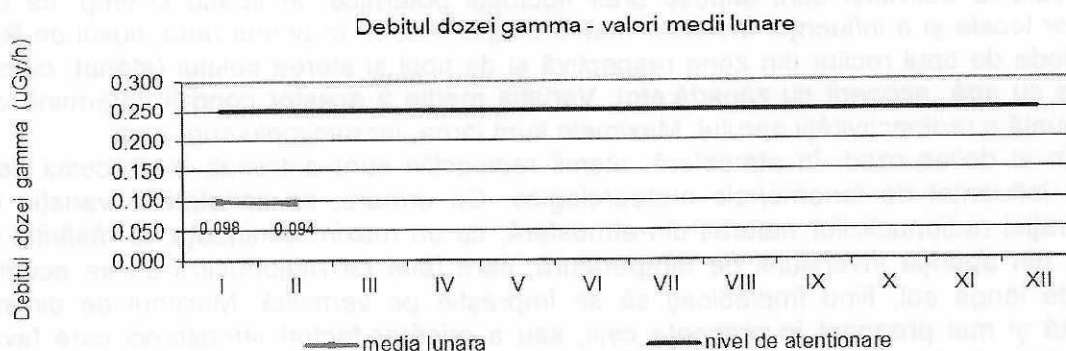
Fig. 1.2.3. Activitatea debitului gamma
