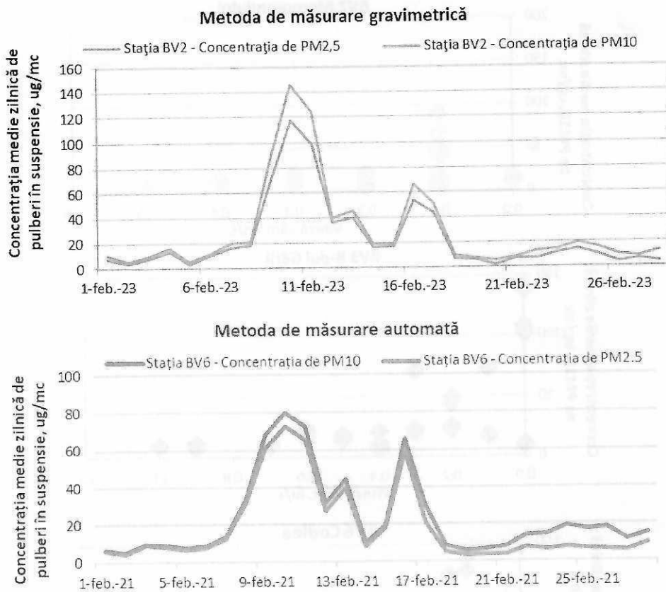
Figura 1.1.2.4.4 Evoluția mediilor zilnice de PM 2,5 și PM10 în luna februarie
