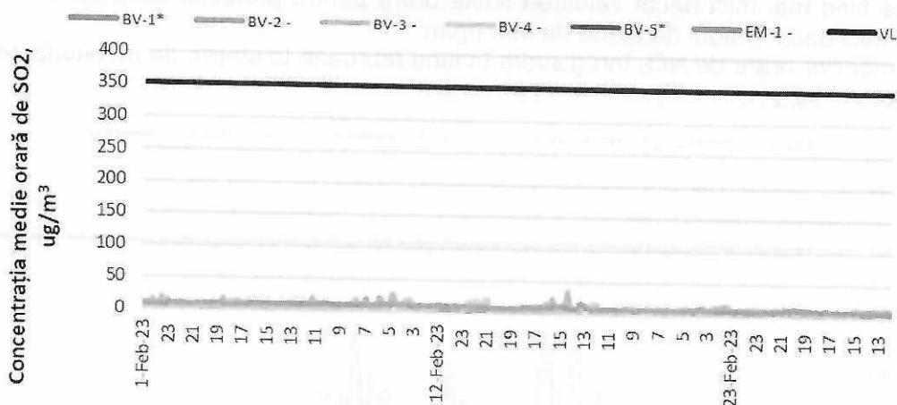
Figura 1.1.2.1.2. Evoluția mediilor orare de SO 2 în luna februarie
