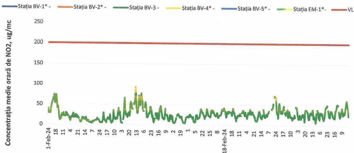
Figura 1. Evoluția concentrației medii orare de \text{NO}_2 în luna februarie 2024
