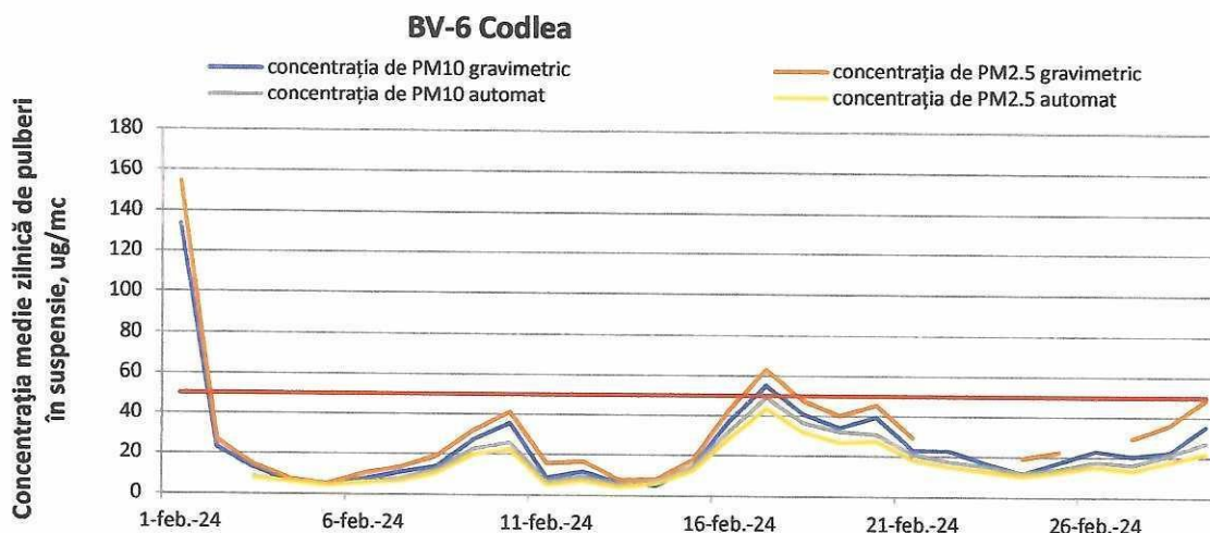
Figura 10. Evoluția concentrațiilor mediilor zilnice de PM10 și PM2,5 (gravimetric) și PM10 și PM2,5 (automat) la stația BV6, în luna februarie 2024
