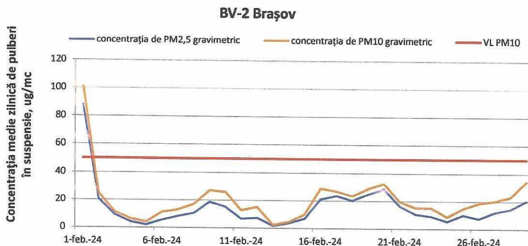
Figura 9. Evoluția concentrațiilor mediilor zilnice de PM10 și PM2,5 (gravimetric) la stația BV2, în luna februarie 2024
