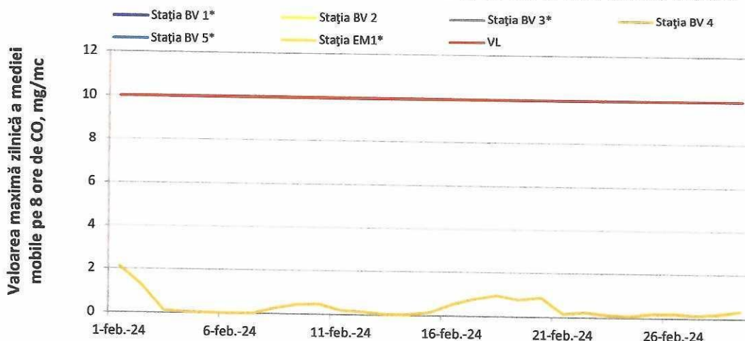
Figura 2. Evoluția maximelor zilnice ale mediei mobile de CO în luna februarie 2024
