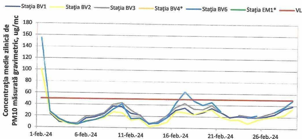
Figura 5. Evoluția concentrațiilor mediilor zilnice de PM 10 (gravimetric) în luna februarie 2024
