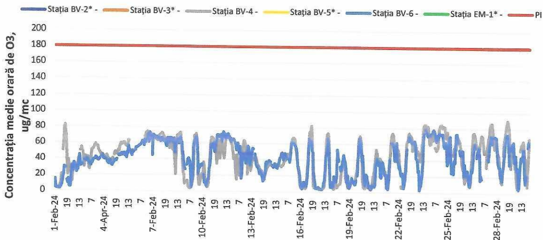
Figura 4. Evoluția concentrațiilor medii orare de O 3 în luna februarie 2024
