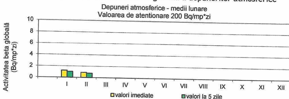
Figura 17. Activitatea beta globală a depunerilor atmosferice
