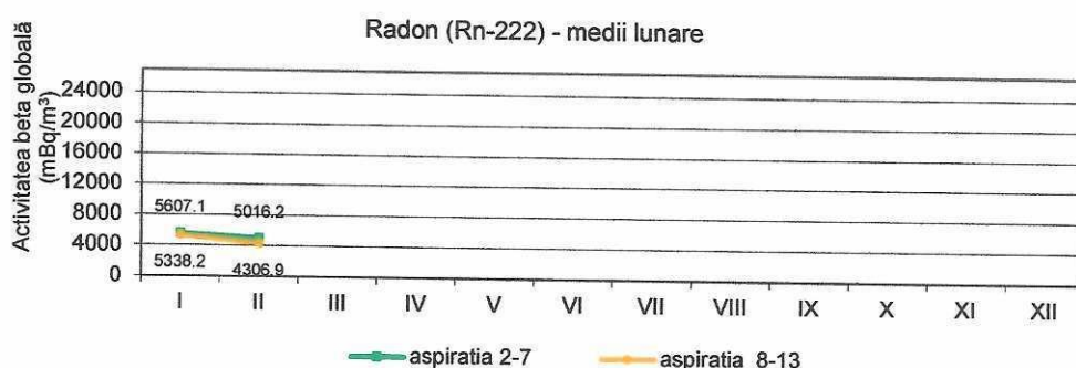
Figura 15. Activitatea calculată a Radonului
