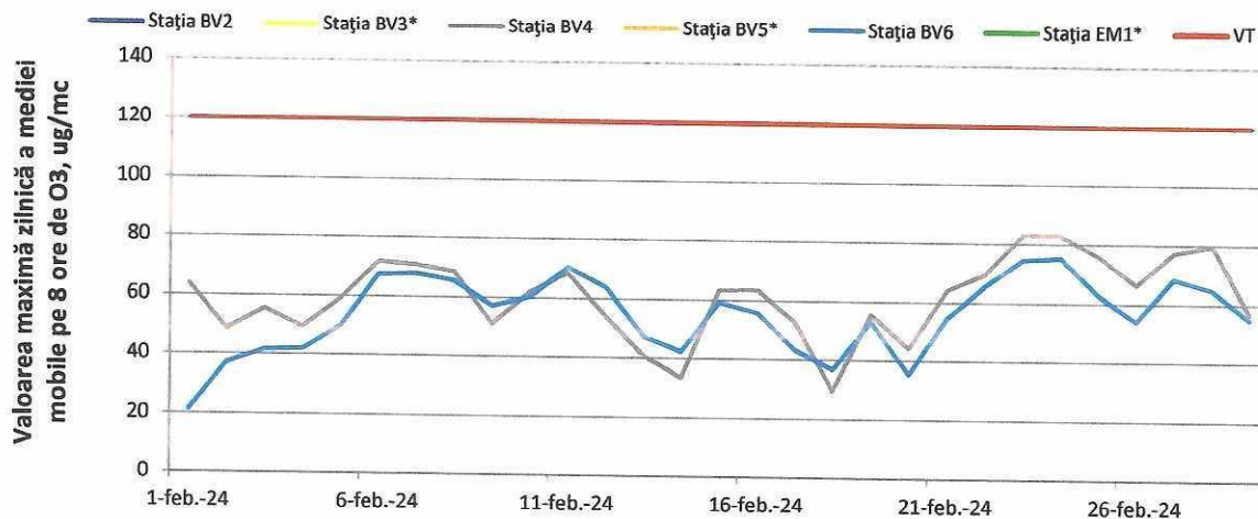
Figura 3. Evoluția concentrațiilor maxime zilnice ale mediilor mobile pe 8 ore de O 3 în luna februarie 2024
