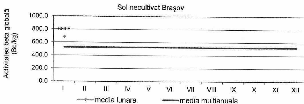
Fig. 21. Activitatea beta globală la 5 zile pentru solul necultivat
