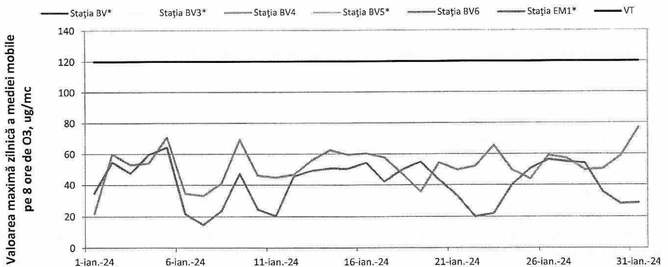
Figura 3. Evoluția concentrațiilor maximelor zilnice ale mediilor mobile pe 8 ore de O 3 în luna ianuarie 2024
