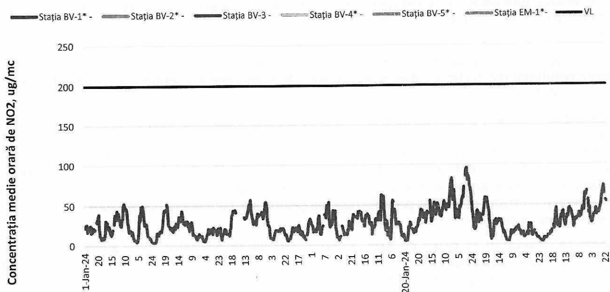
Figura 1. Concentrații medii orare de NO 2 în luna ianuarie 2024
