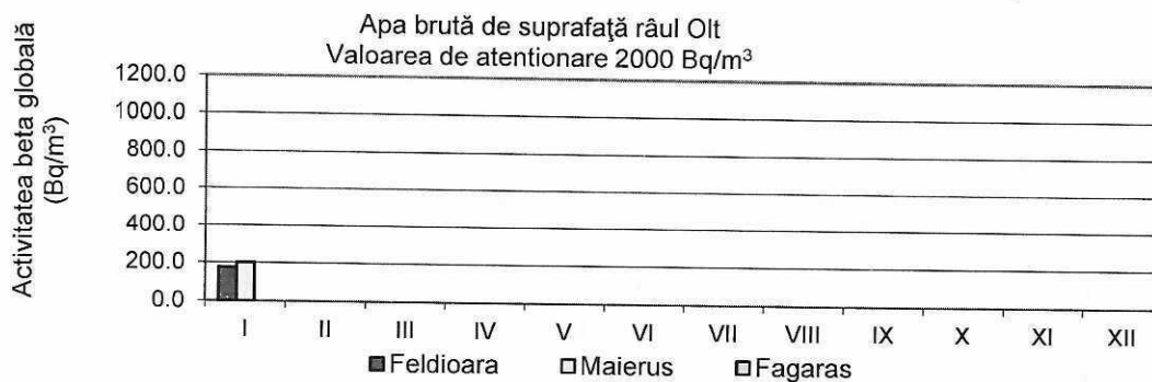
Fig. 20. Activitatea beta globală la 5 zile pentru apa de suprafață Râul Olt
