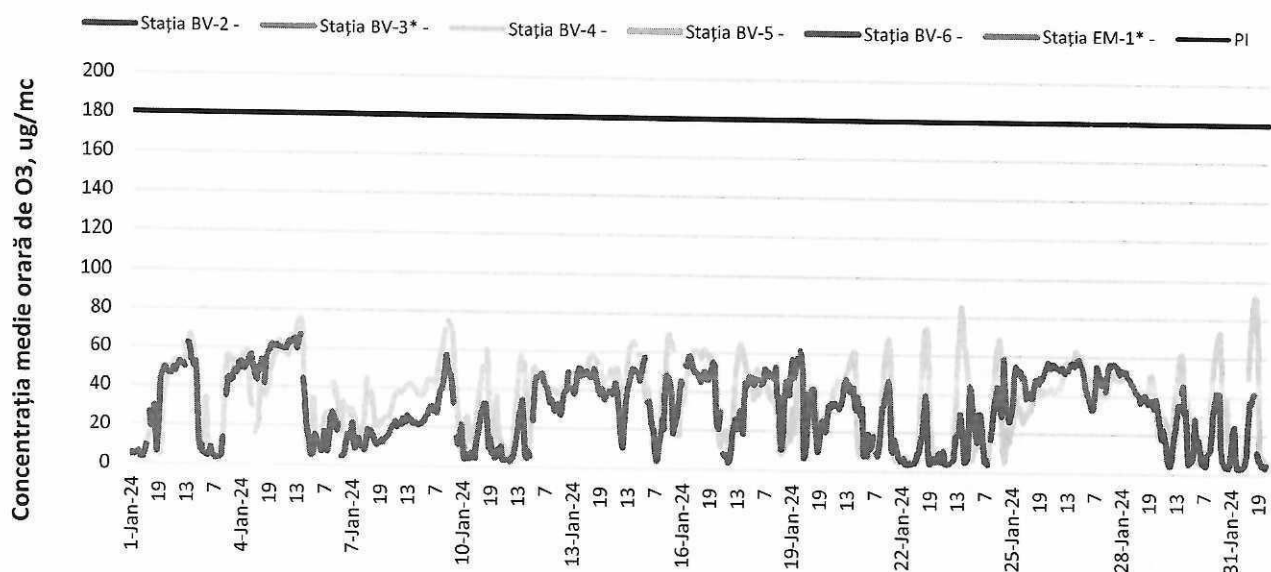
Figura 4. Evoluția concentrațiilor medii orare de O 3 în luna ianuarie 2024
