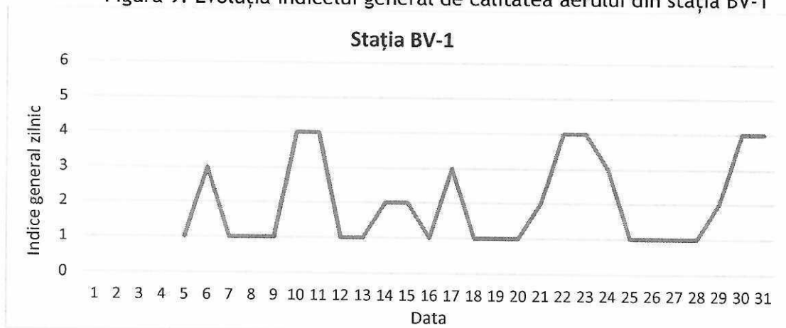
Figura 9. Evoluția indicelui general de calitate a aerului din stația BV-1
