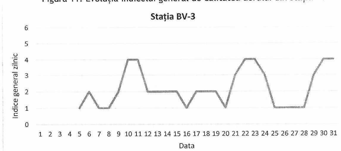
Figura 11. Evoluția indicelui general de calitate a aerului din stația BV-3
