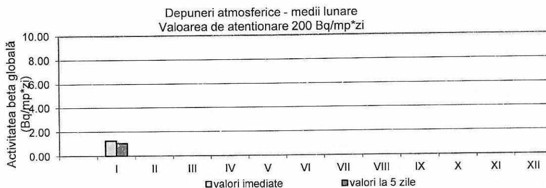
Figura 17. Activitatea beta globală pentru depuneri atmosferice
