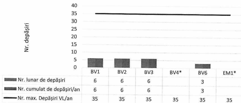
Figura 6. Numărul lunar și cumulat de depășiri ale valorii limită zilnice la PM10
