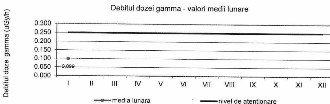
Figura 16. Debitul dozei gamma
