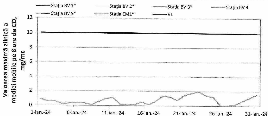
Figura 2. Evoluția maximelor zilnice ale mediei mobile de CO în luna ianuarie 2024
