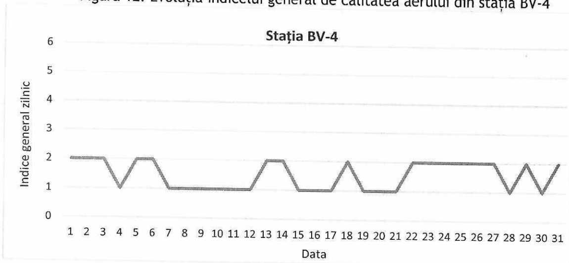
Figura 12. Evoluția indicelui general de calitate a aerului din stația BV-4
