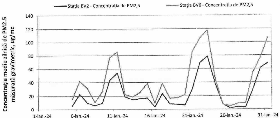
Figura 8. Evoluția mediilor zilnice de PM 2,5 (gravimetric) în luna ianuarie 2024
