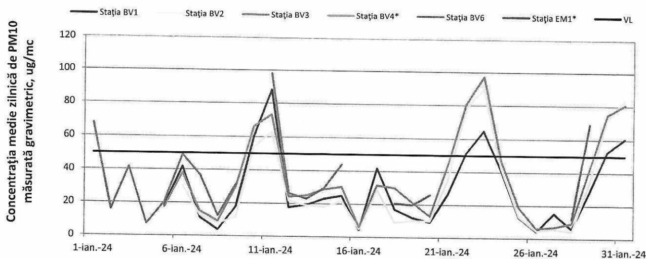
Figura 5. Evoluția mediilor zilnice de PM 10 (gravimetric) în luna ianuarie 2024
