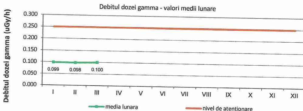
Fig. 16. Debitul dozei gamma în aer
