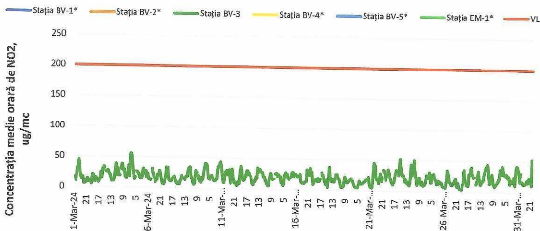
Figura 1. Concentrații medii orare de NO 2 în luna martie 2024
