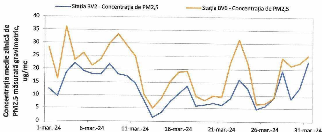
Figura 8. Evoluția mediilor zilnice de PM 2,5 (gravimetric) în luna martie 2024
