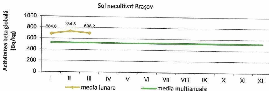
Fig. 21. Activitatea beta globală la 5 zile pentru solul necultivat
