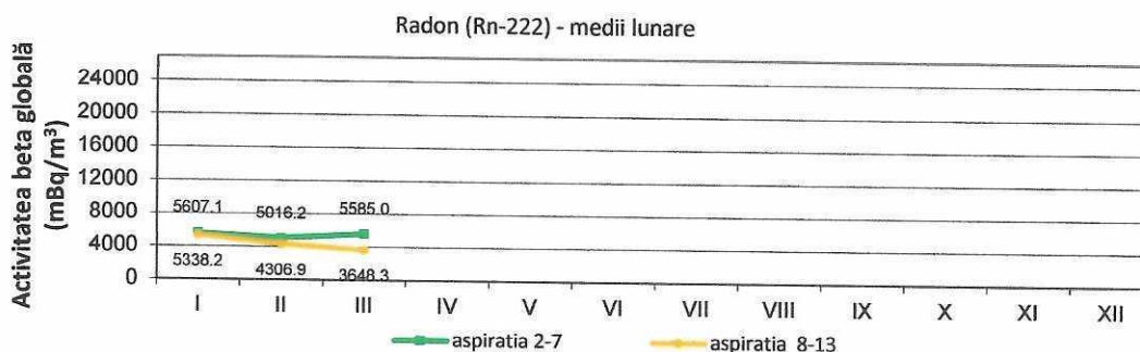
Fig. 15. Activitatea calculată a Radonului
