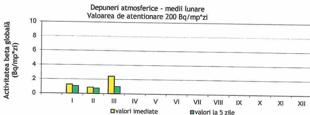
Fig. 17. Activitatea beta globală pentru depuneri atmosferice
