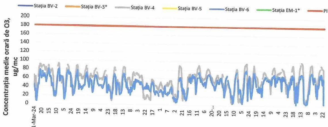
Figura 4. Evoluția concentrațiilor medii orare de O 3 în luna martie 2024
