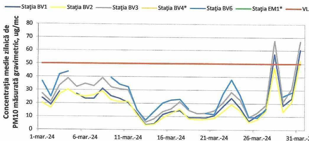
Figura 5. Evoluția mediilor zilnice de PM 10 (gravimetric) în luna martie 2024
