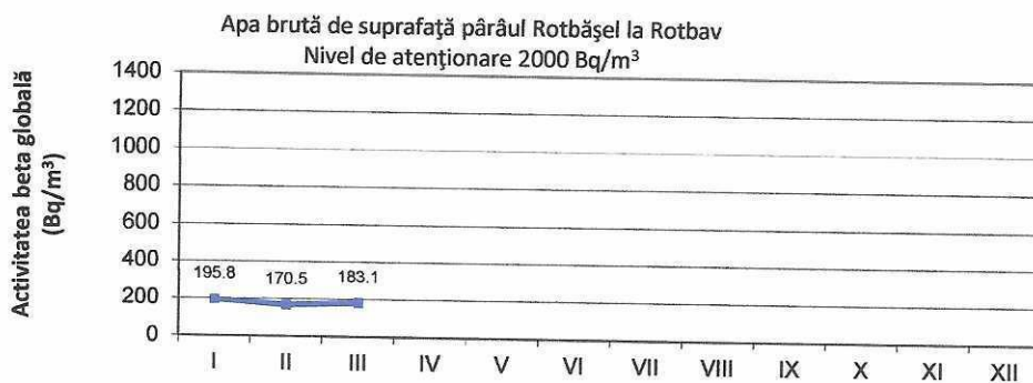
Fig. 19. Activitatea beta globală la 5 zile pentru apa de suprafață-Pârâul Rotbășel
