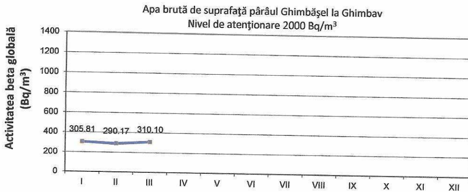
Fig. 18. Activitatea beta globală imediată pentru apa de suprafață Pârâul Ghimbășel
