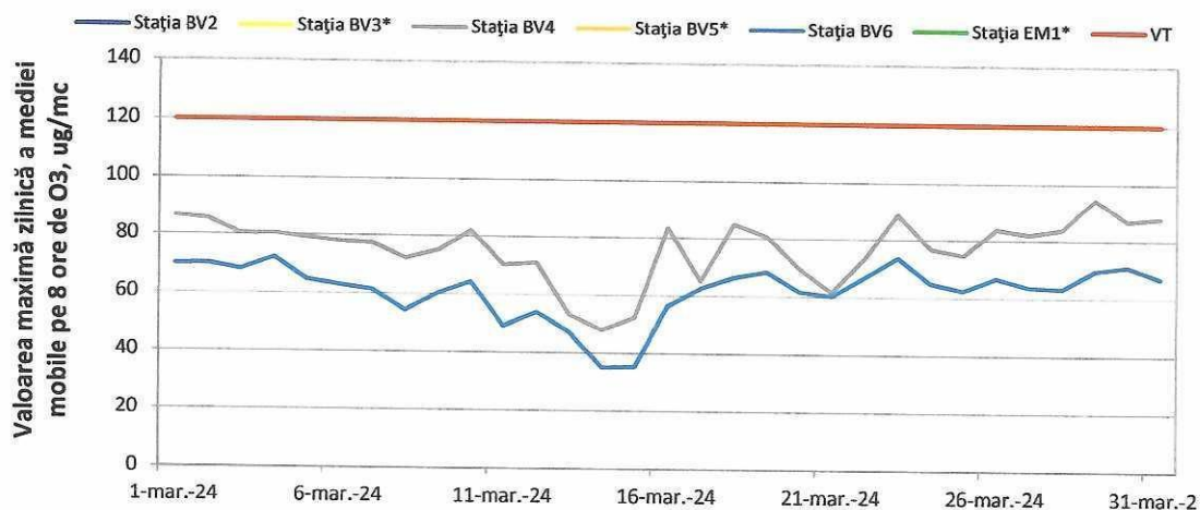
Figura 3. Evoluția concentrațiilor maximelor zilnice ale mediilor mobile pe 8 ore de O 3 în luna martie 2024
