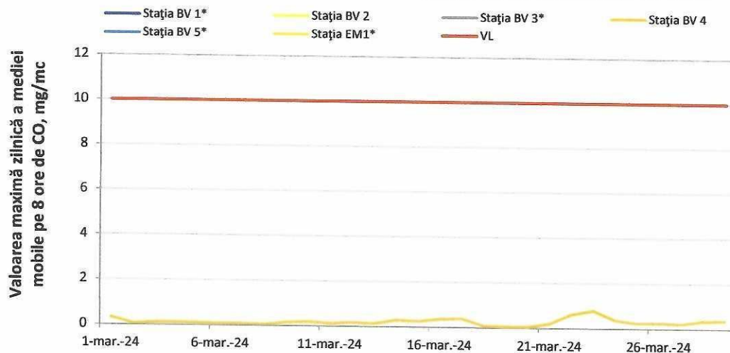
Figura 2. Evoluția maximelor zilnice ale mediei mobile de CO în luna martie 2024
