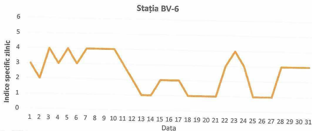
Figura 13. Evoluția indicelui general de calitate a aerului din stația BV-6
