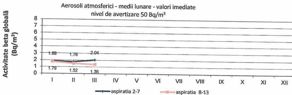
Fig. 14. Activitatea beta globală pentru aerosoli atmosferici
