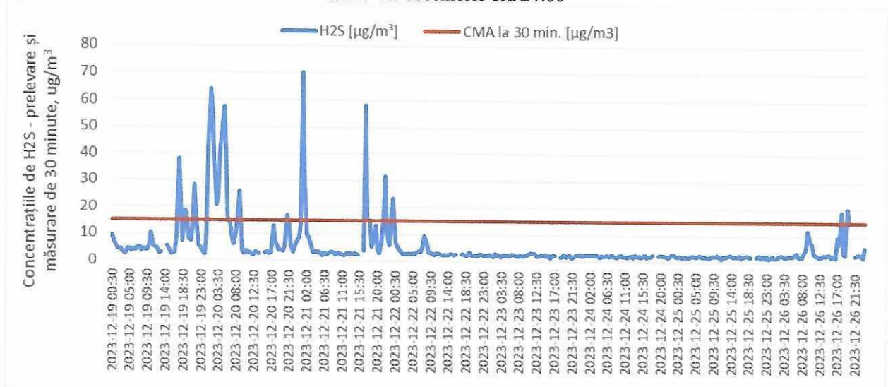
Figura 2. Evoluția concentrațiilor de H 2 S - medii la 30 minute, înregistrate în perioada 19 decembrie, ora 00:00–26 decembrie ora 24:00
