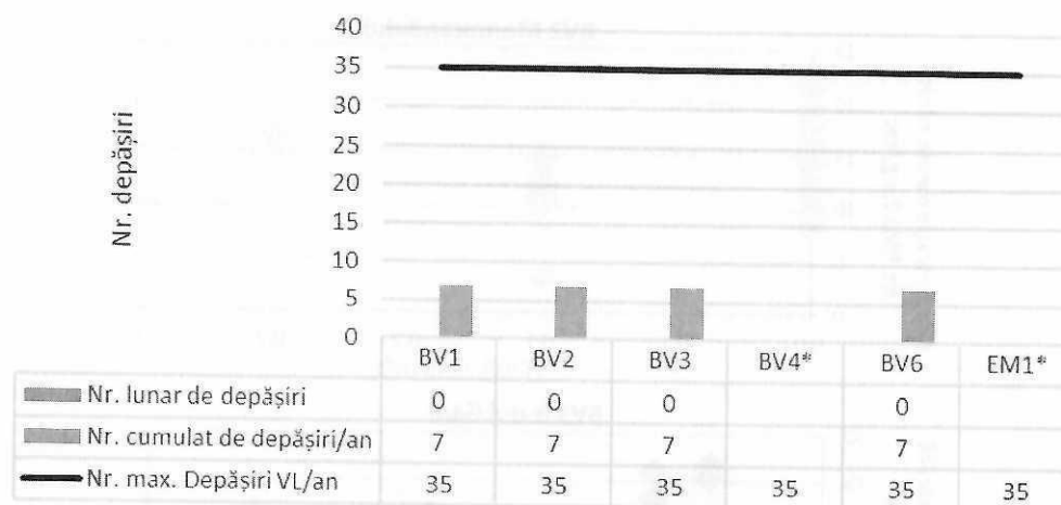
Figura 1.1.2.4.2 Numărul lunar și cumulativ de depășiri ale valorii limită zilnice la PM10
