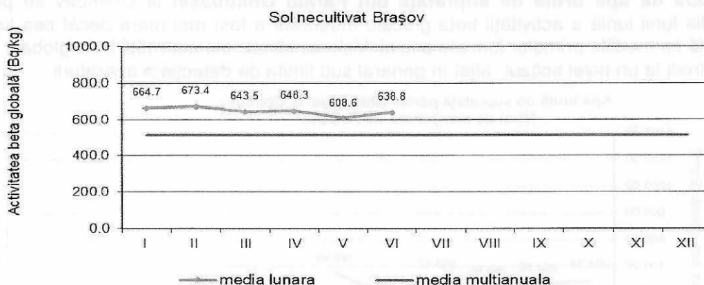
Fig. 1.2.8. Activitatea beta globală pentru sol necultivat
