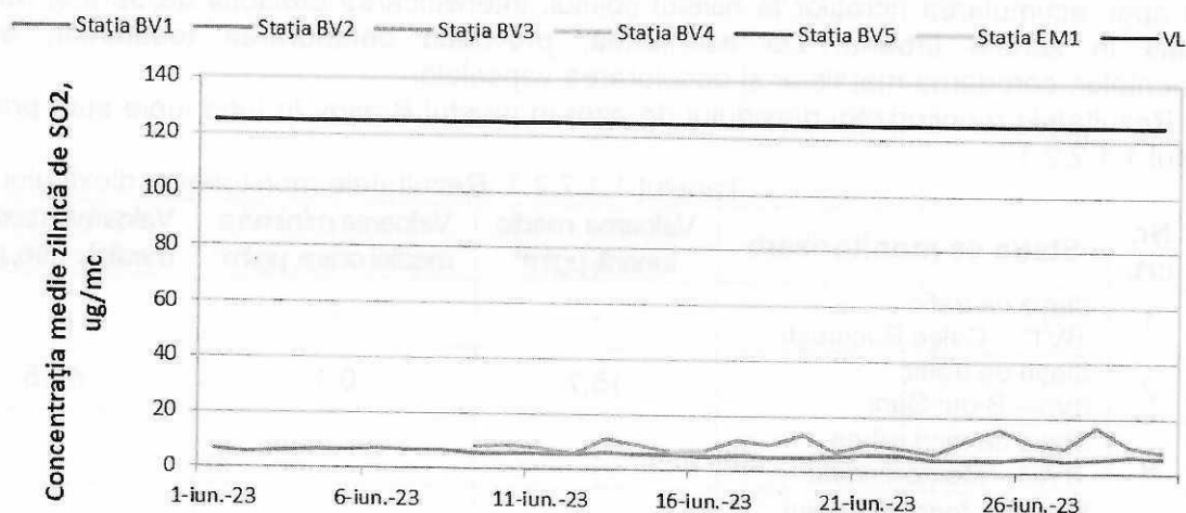
Figura 1.1.2.1.1. Evoluția mediilor zilnice de \text{SO}_2 în luna iunie
