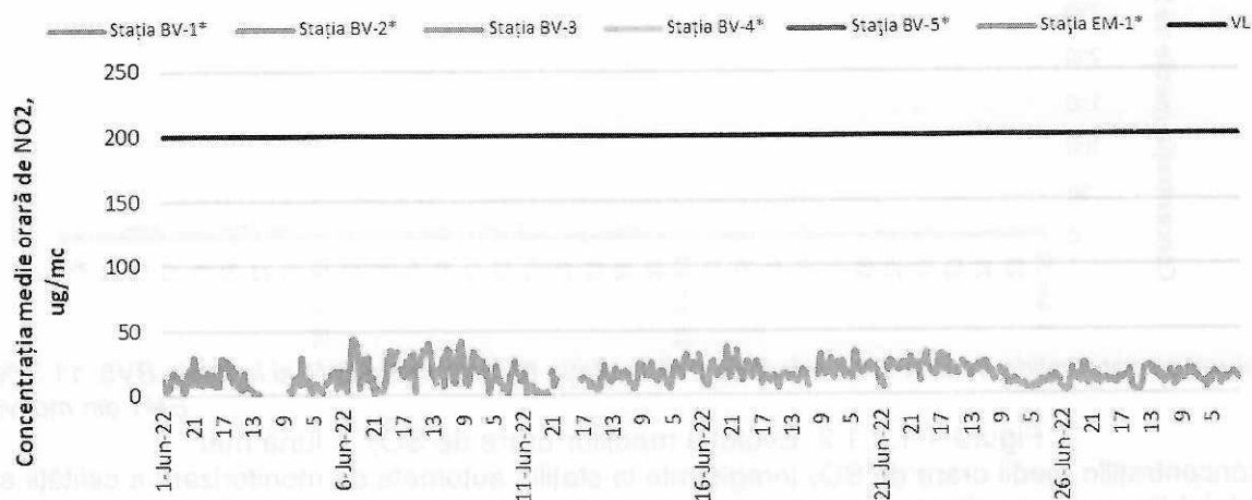
Figura 1.1.2.2.1. Evoluția mediilor orare de \text{NO}_2 în luna iunie
