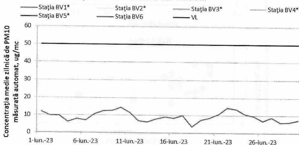
Figura 1.1.2.4.3. Evoluția mediilor zilnice de PM 10, metoda automată, în luna iunie
