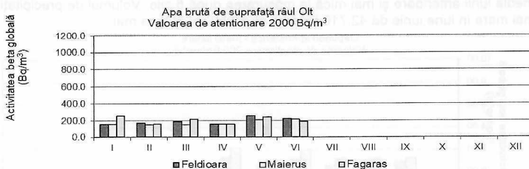
Fig. 1.2.7. Activitatea beta globală la 5 zile pentru apa de suprafață Râul Olt
