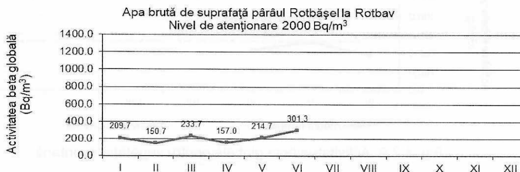
Fig. 1.2.6. Activitatea beta globală la 5 zile pentru apa de suprafață-Pârâul Rotbășel
