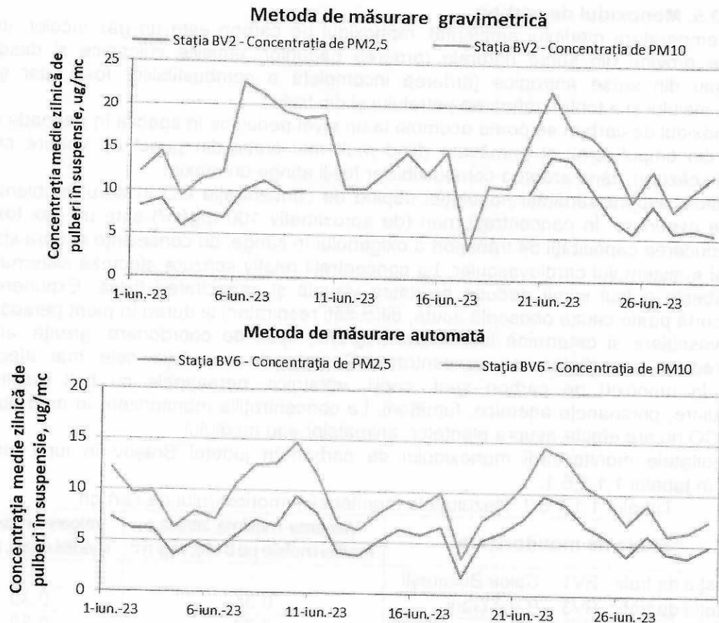
Figura 1.1.2.4.4 Evoluția mediilor zilnice de PM 2,5 și PM10 în luna iunie
