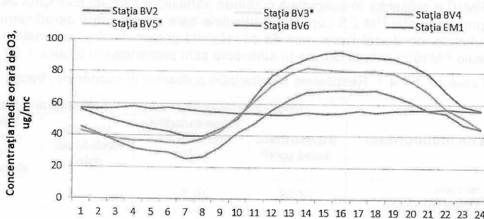
Figura 1.1.2.3.3. Ciclul zilnic al ozonului
