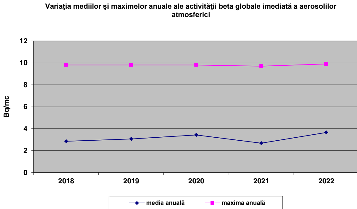
Figura IX.1.1.3 Variația mediilor și maximelor anuale ale activității beta globale imediată a aerosolilor atmosferici
