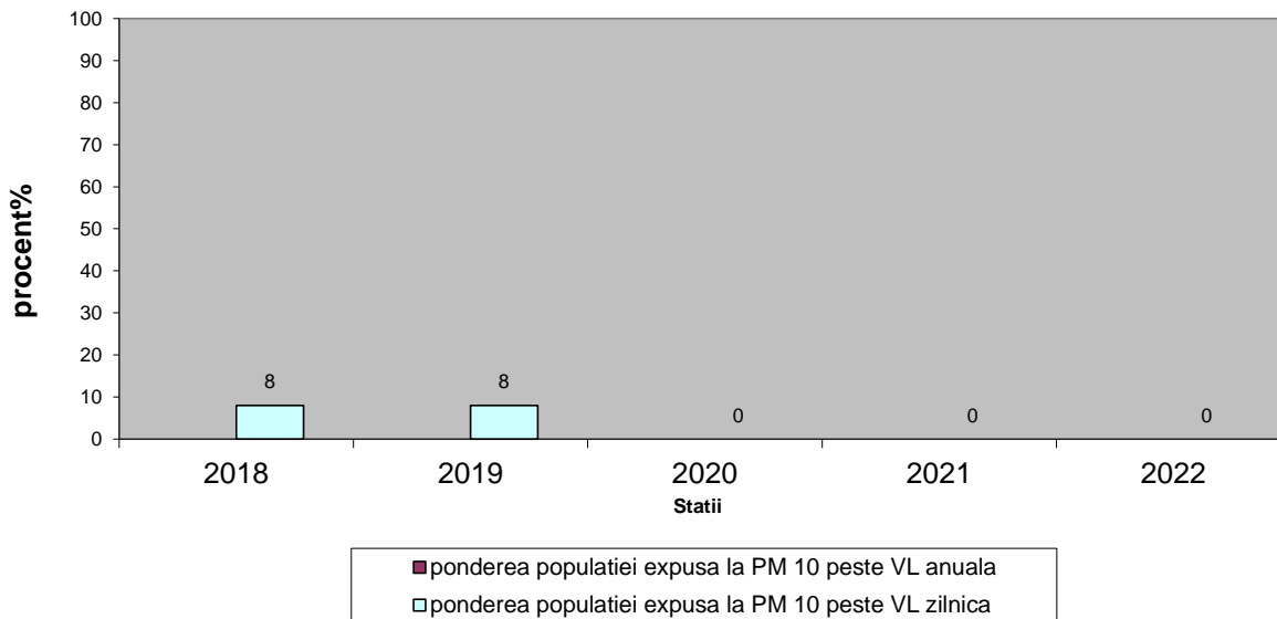
Ponderea populației expusa la concentrații de PM10
