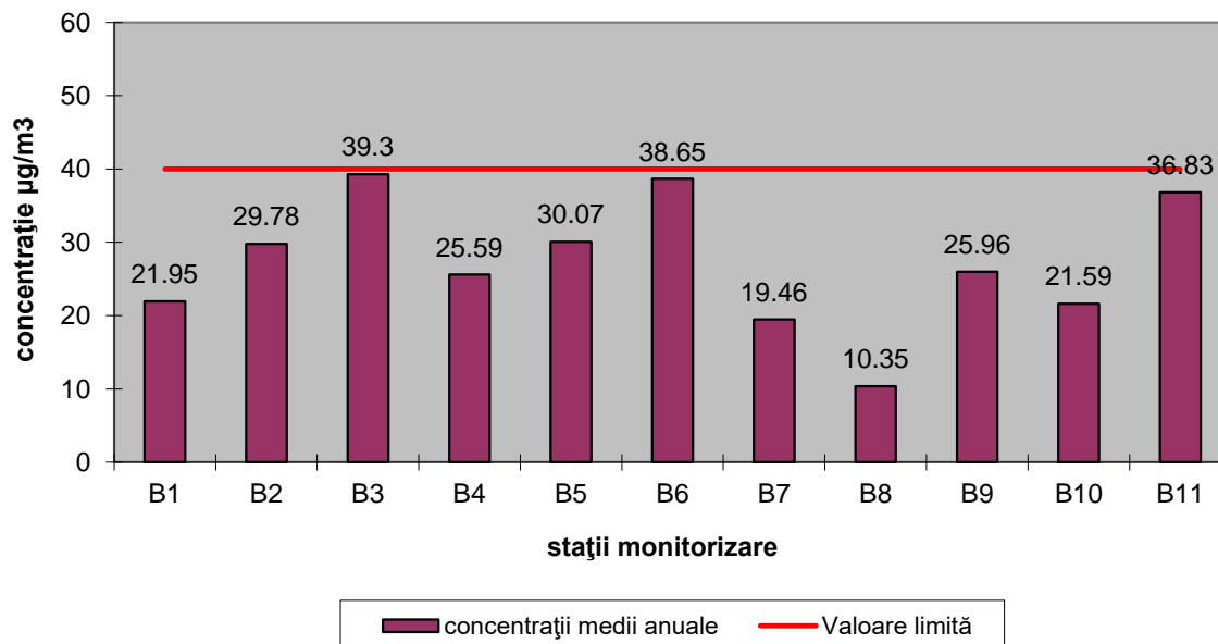
NO2 Concentrații medii anuale 2022 înregistrate la stațiile de monitorizare
