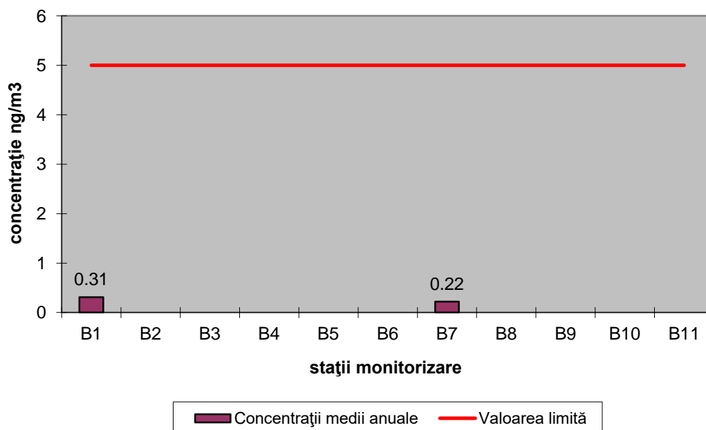
Cd - Concentrații medii anuale 2022 înregistrate la stațiile de monitorizare
