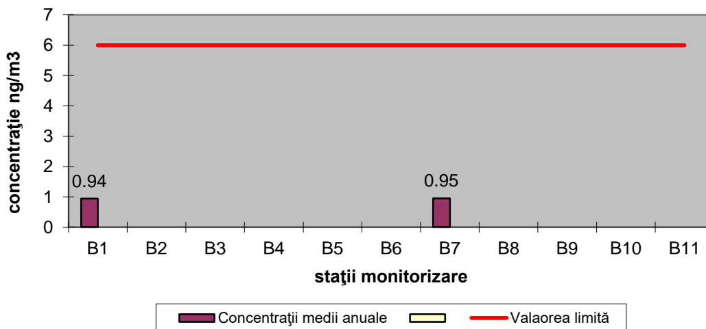
As - Concentrații medii anuale 2022 înregistrate la stațiile de monitorizare
