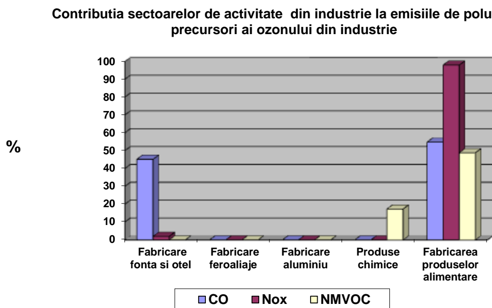
grafic 1.2.2.4 Contributia sectoarelor de activitate din industrie la emisiile de poluanti precursori ai ozonului din industrie, in anul 2021
