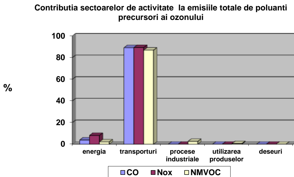
grafic 1.2.2.3 Contributia sectoarelor de activitate la emisiile de poluanti precursori ai ozonului in anul 2021
