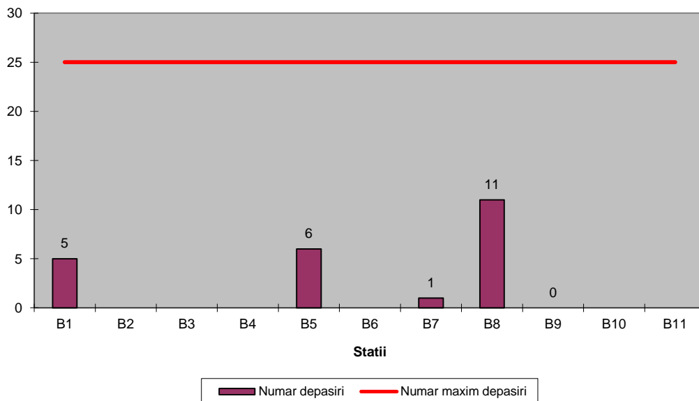
O3- Număr zile cu depășiri ale valorii țintă în anul 2022
