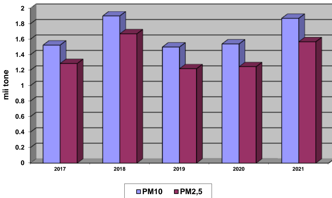
Evoluția emisiilor de particule primare în suspensie
