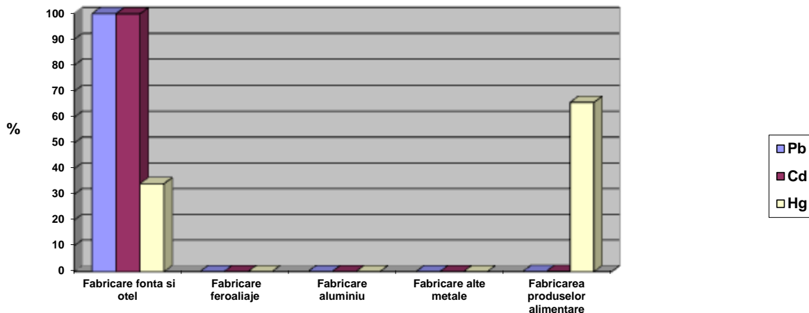
Contributia sectoarelor de activitate din industrie la emisiile de metale grele din industrie
