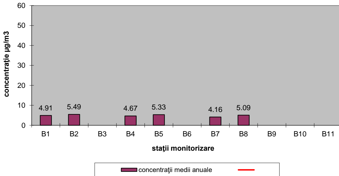
SO2 Concentrații medii anuale 2022 înregistrate la stațiile de monitorizare
