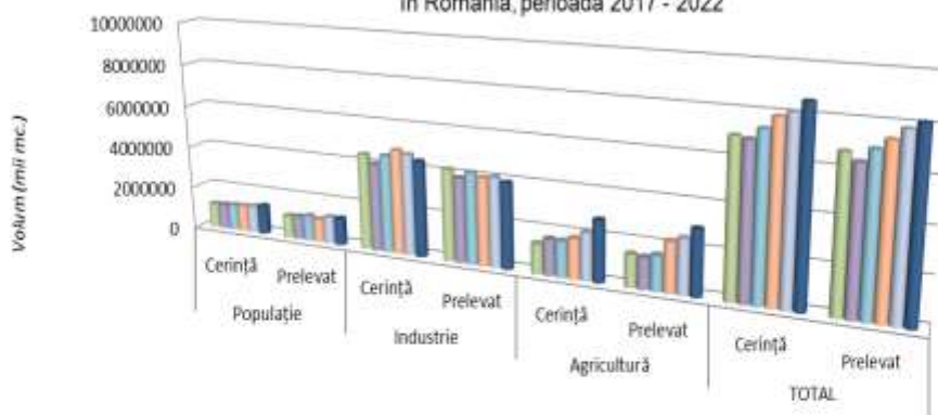
Figura 2/Tabelul II.1.1.2 Evoluția cerinței de apă comparativ cu prelevarea volumelor de apă în România, perioada 2017 - 2022
