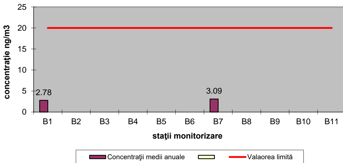
Ni - Concentrații medii anuale 2022 înregistrate la stațiile de monitorizare
