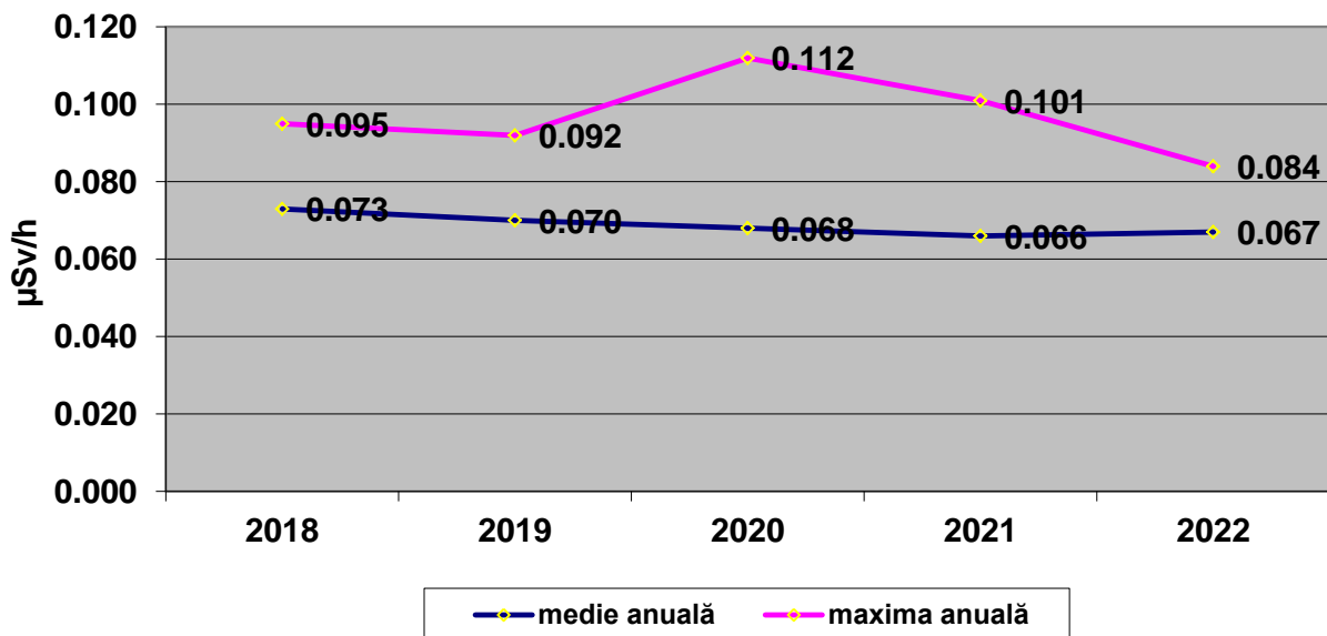
Variația mediilor și maximelor anuale ale debitului dozei gama
