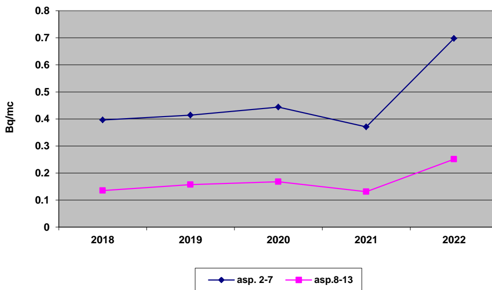
Variația activității specifice medie anuală a toronului din atmosferă în funcție de variația diurnă
