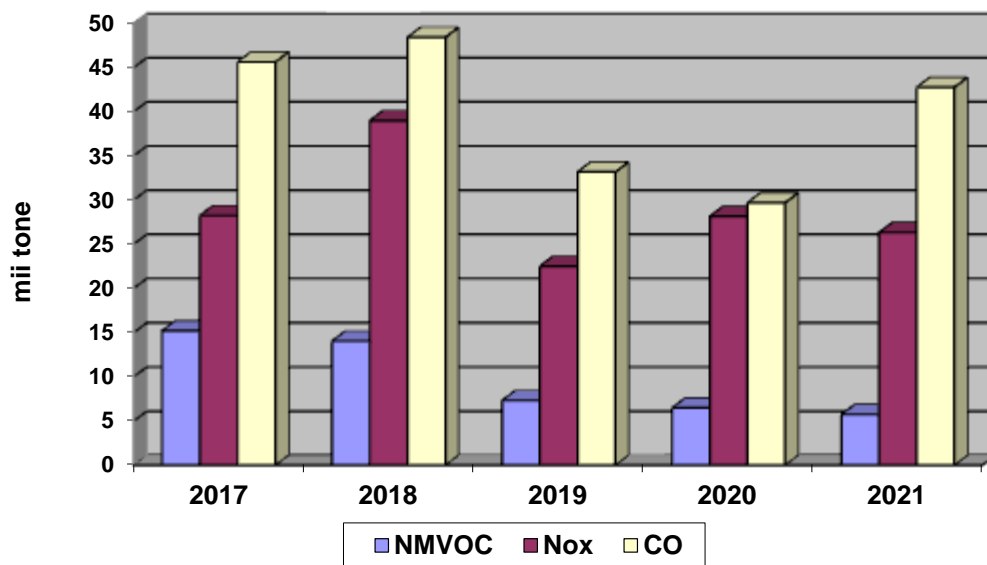
Evoluția emisiilor de poluanți precursori ai ozonului
