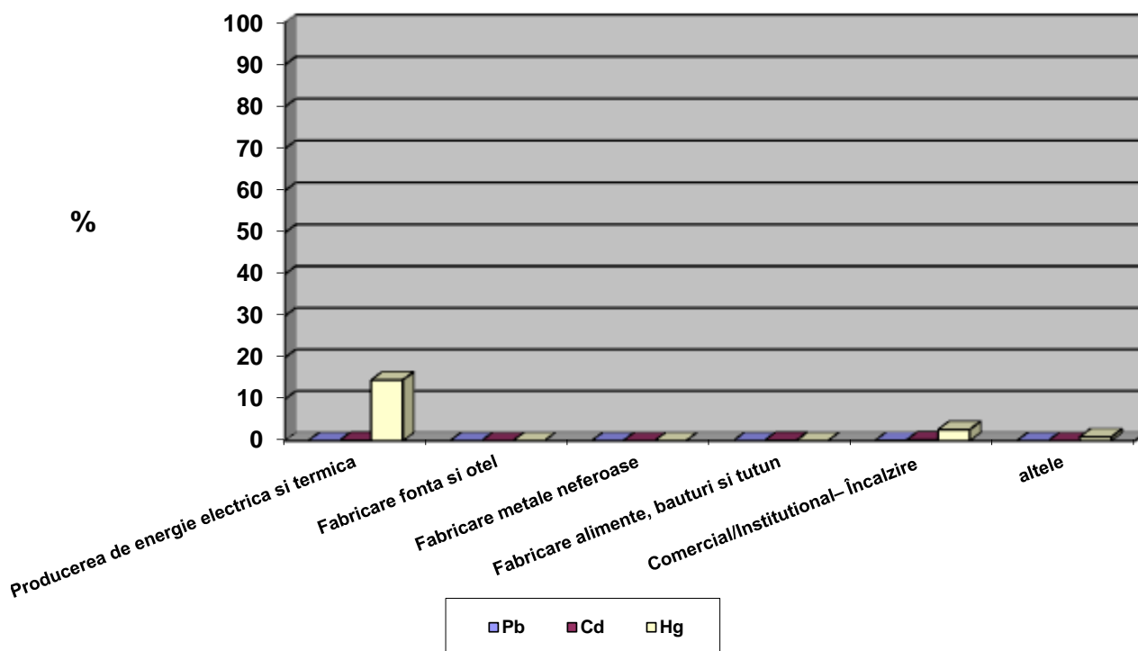
Contribuția sectoarelor de activitate din energie, la emisiile totale de metale grele, in anul 2021
