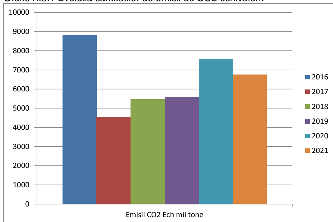
Grafic X.3.1 Evoluția cantitatilor de emisii de CO2 echivalent
