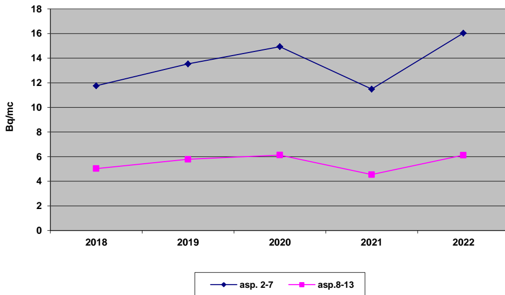
Figura IX.1.1.5 Variația activității specifice medie anuală a toronului din atmosferă în funcție de variația diurnă
