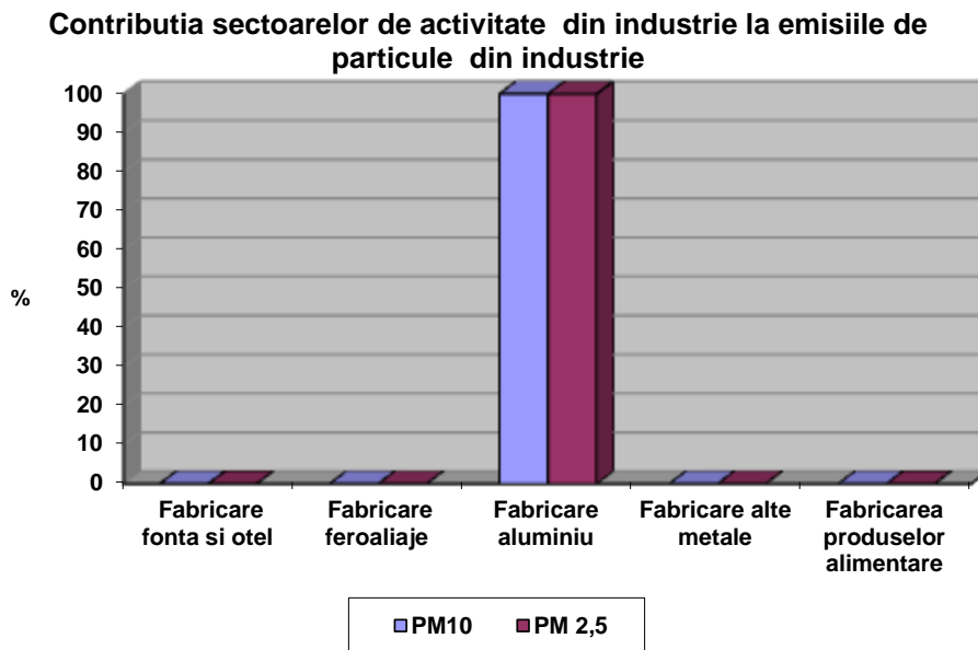
grafic 1.2.2.6 Contributia sectoarelor de activitate din industrie la emisiile particule provenite din industrie in anul 2021
