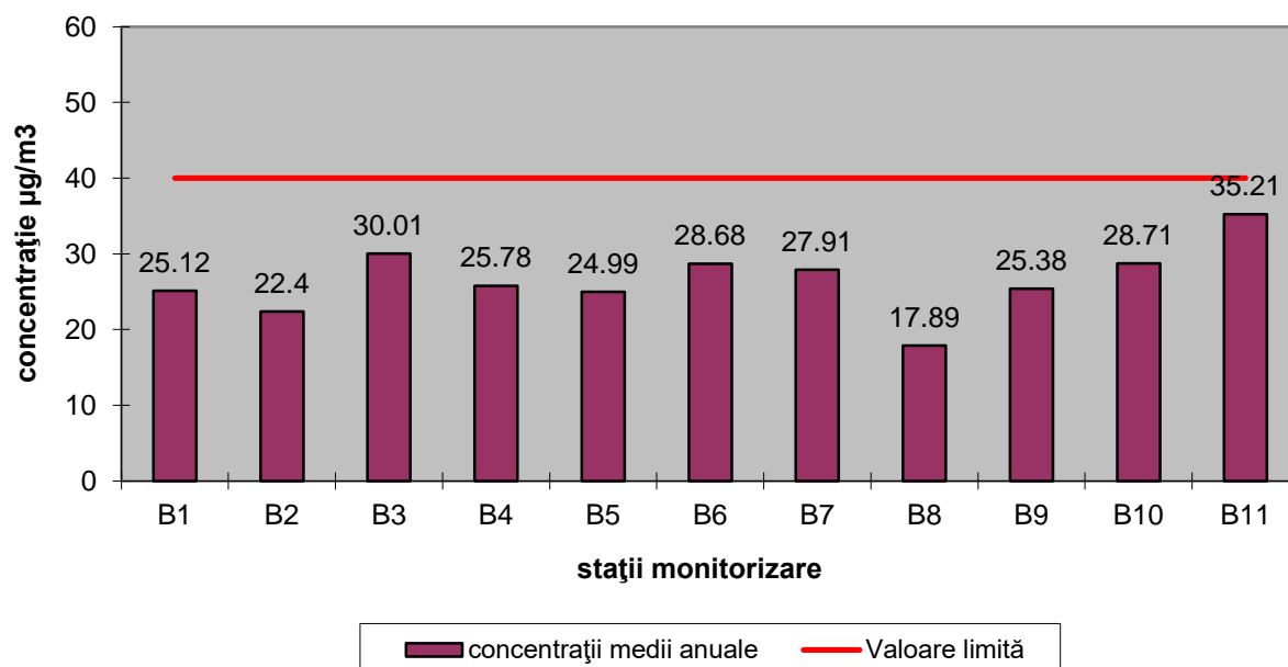
PM10 Concentrații medii anuale 2022 înregistrate la stațiile de monitorizare
