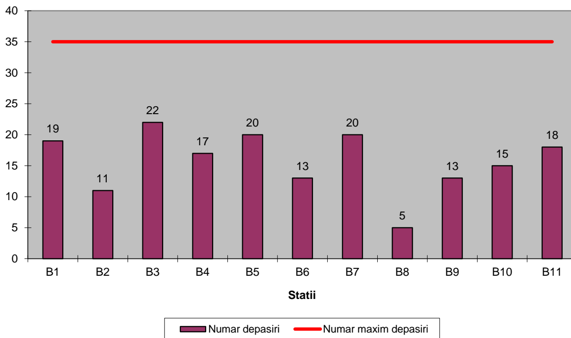
PM10- Număr de depășiri în anul 2022
