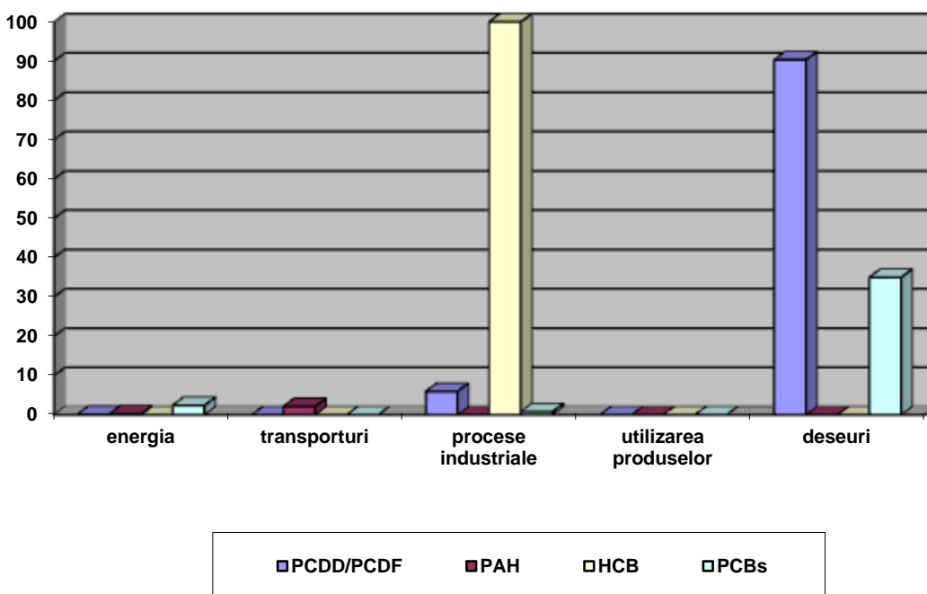
Contribuția sectoarelor de activitate, la emisiile totale de poluanți organici persistenți
