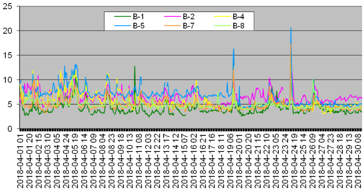
SO2 aprilie 2018 Valori orare Valoare [ \mu\text{g}/\text{m}^3 ]
