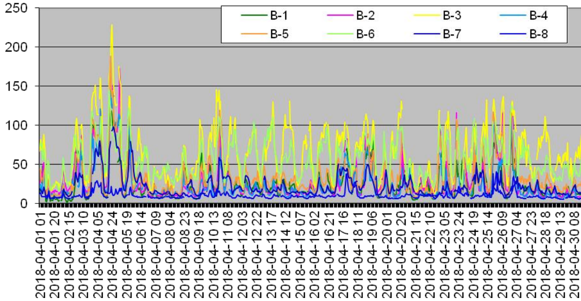
NO2 aprilie 2018 Valori orare Valoare [ \mu\text{g}/\text{m}^3 ]
