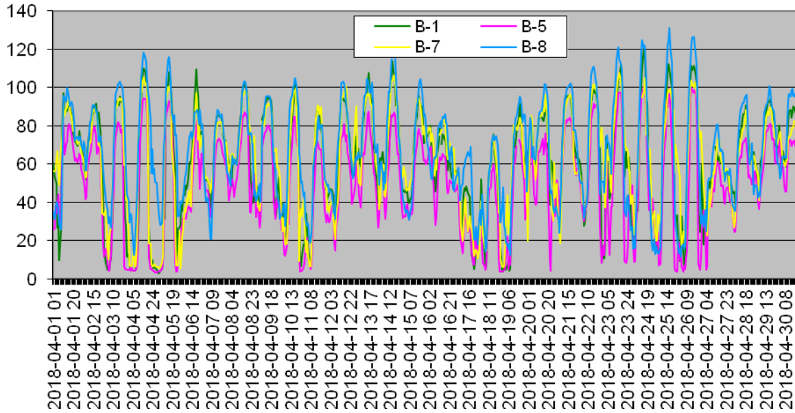
O3 aprilie 2018 Valori orare Valoare [ \mu\text{g}/\text{m}^3 ]
