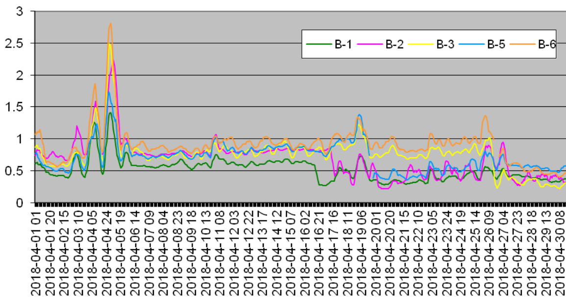
CO aprilie 2018 Media mobila orara Valoare [mg/m 3 ]
