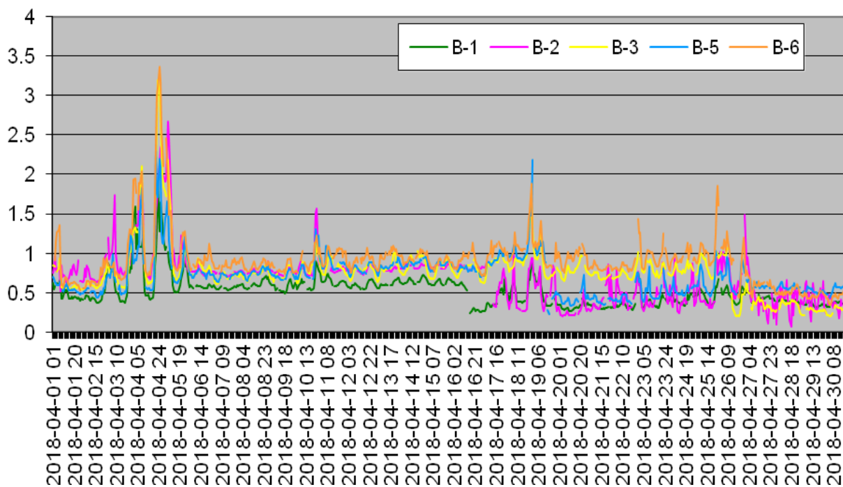
CO aprilie 2018 Valori orare Valoare [mg/m 3 ]
