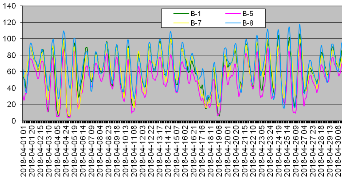
O3 aprilie 2018 Media mobila orara Valoare [ \mu\text{g}/\text{m}^3 ]
