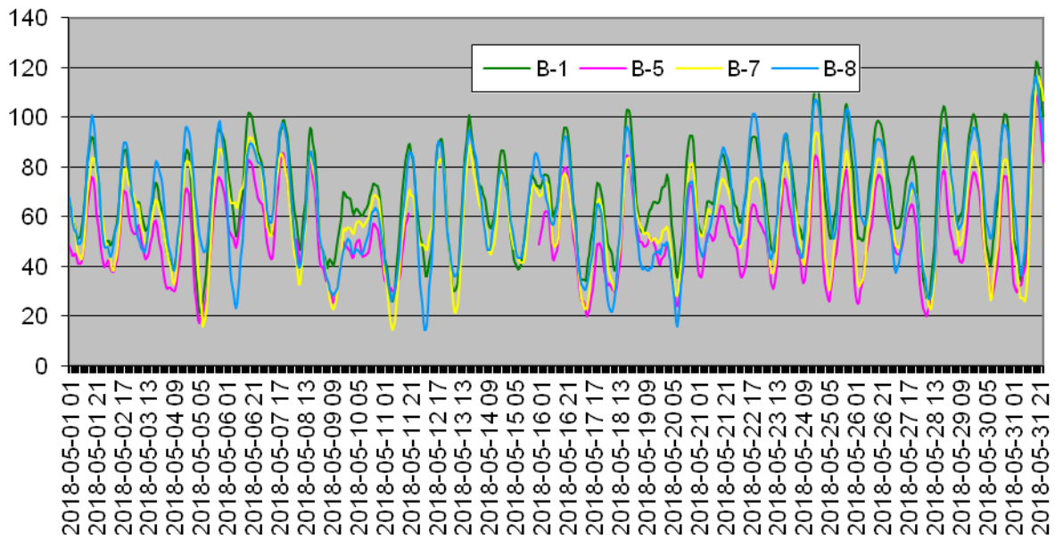
O3 mai 2018 Media mobila orara Valoare [ \mu\text{g}/\text{m}^3 ]
