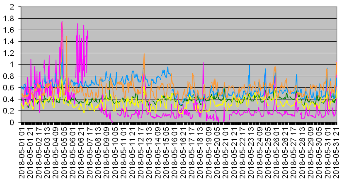
CO mai 2018 Valori orare Valoare [mg/m 3 ]
