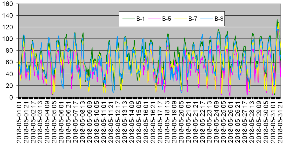
O3 mai 2018 Valori orare Valoare [ \mu\text{g}/\text{m}^3 ]
