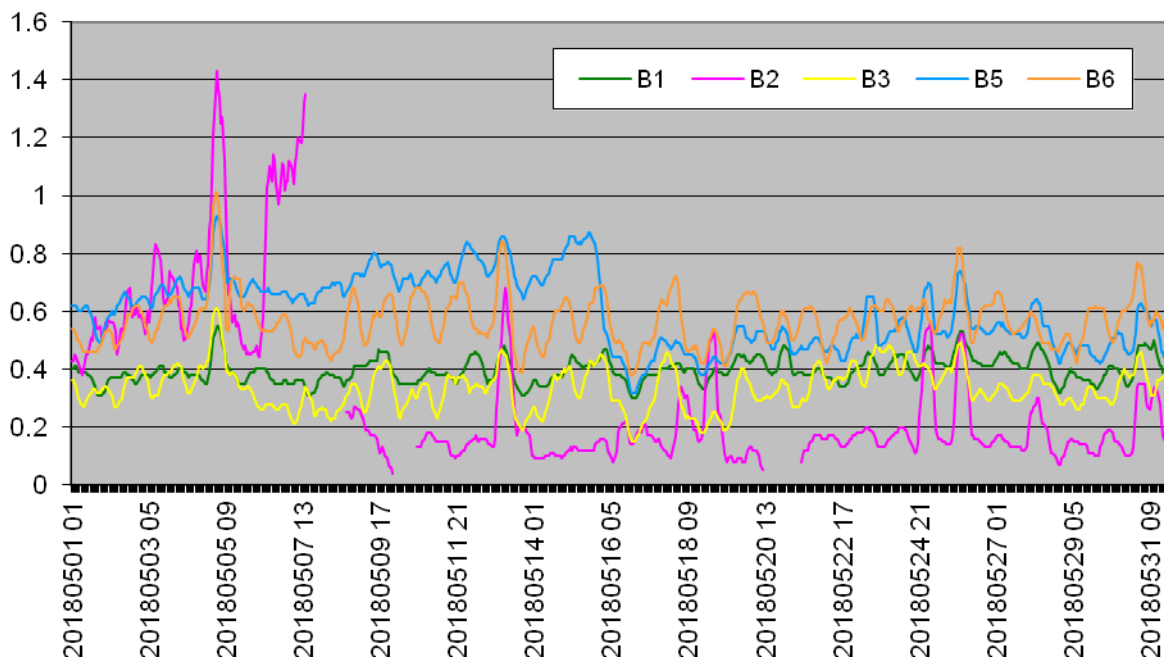
CO mai 2018 Media mobila orara Valoare [mg/m 3 ]
