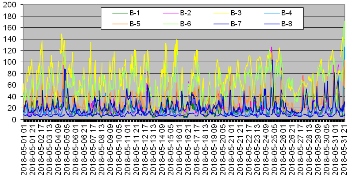
NO2 mai 2018 Valori orare Valoare [ \mu\text{g}/\text{m}^3 ]
