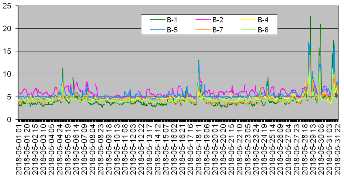
SO2 mai 2018 Valori orare Valoare [ \mu\text{g}/\text{m}^3 ]
