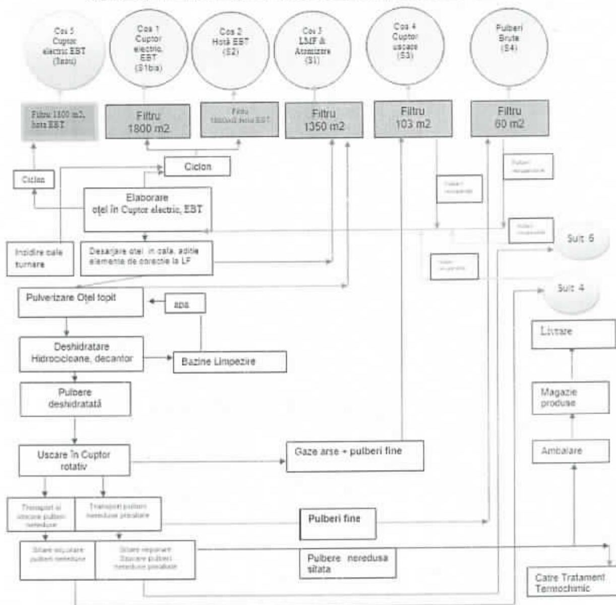
Anexa 2 - Schema flux tehnologic si sursele de emisie la fabricarea pulberilor feroase brute
