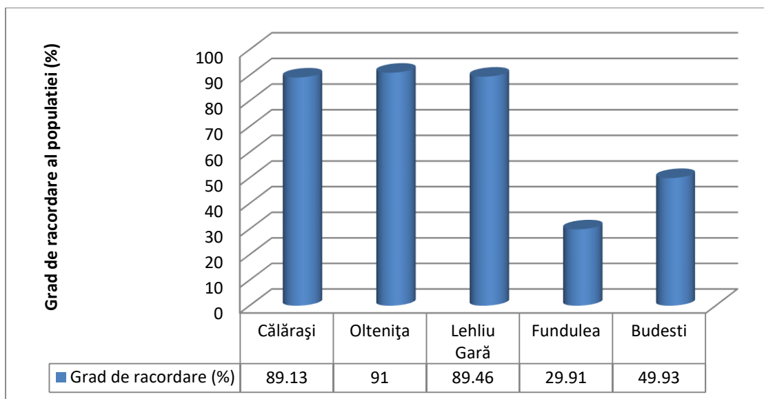
Figura 2.2.2.2.1. Gradul de racordare al populației urbane la sistemele de canalizare și epurare în anul 2017 în județul Călărași (Sursa : S.C. Ecoaqua S.A. Călărași)
