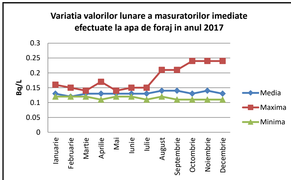
Figura nr. IX.1.2.2 .Media lunară a activității beta specifice – măsurători imediate pentru apa de foraj în municipiul Călărași, în anul 2017
