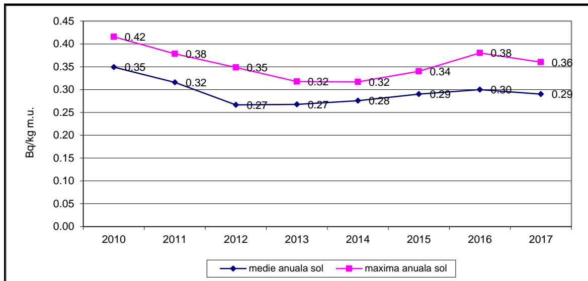
Figura nr. IX.1.3.1. Variația mediilor și maximelor anuale ale activității beta globale a solului în Călărași, în perioada 2010 – 2017
