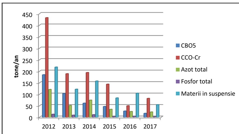
Fig. 2.2.2.2.5. Încărcarea cu poluanți a efluenților evacuați de la aglomerările urbane
