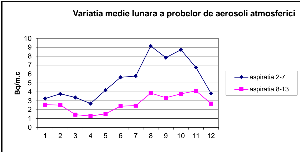
Figura nr. IX.1.1.2. Variațiile mediei lunare pe intervale de aspirație (aspirația 2-7 și aspirația 8-13) ale a activității beta globală (măsurare imediată) a aerosolilor atmosferici în anul 2017
