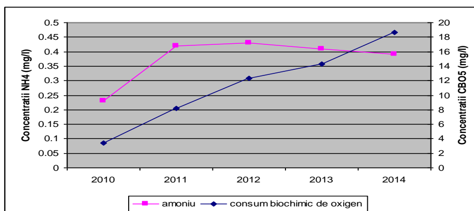
Figura 2.2.1.1.7. Evoluția indicatorilor CBO5 și NH4+ în Dunăre, din județul Călărași, în perioada 2010-2014 (Sursa : prelucrare date de la Administrația Bazinală de Apă Buzău – Ialomița)
