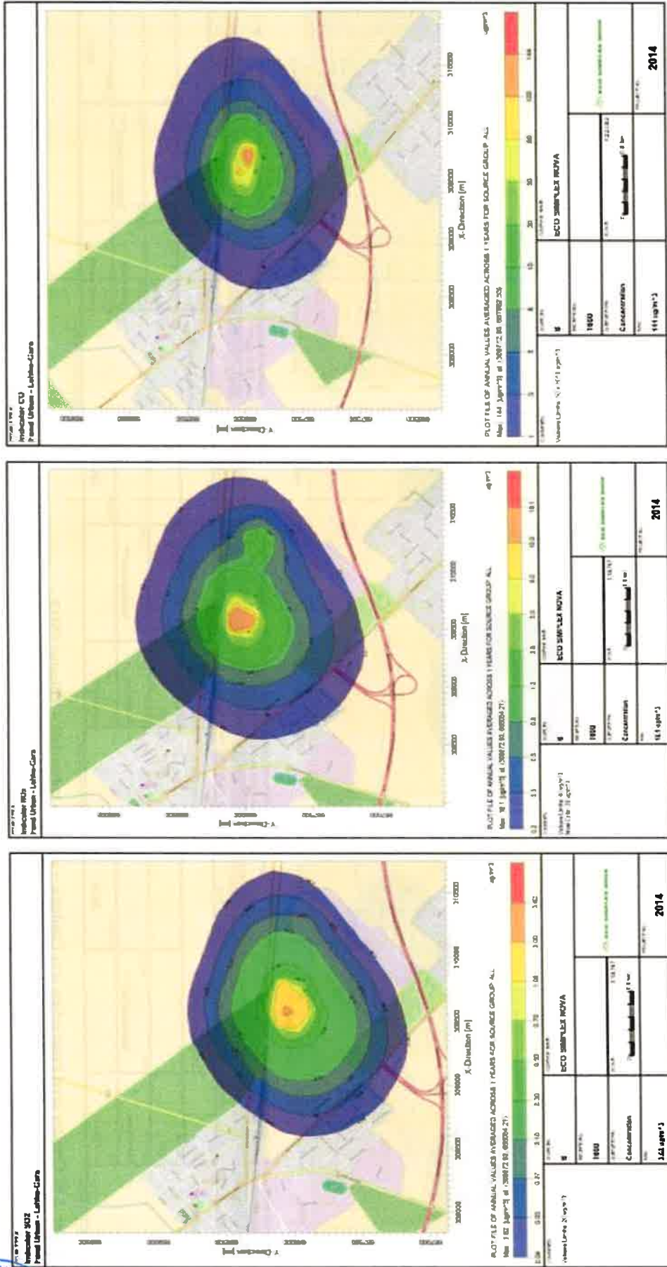
Figura nr. 3-85 Creșterea nivel Fond urban orașLehliu-Gară – activitate industrială - indicator SO2 Figura nr. 3-86 Creșterea nivel Fond urban oraș Lehliu-Gară –activitate industrială – indicator NOx Figura nr. 3-87 Creșterea nivel Fond urban oraș Lehliu-Gară -activitate industrială – indicator CO
