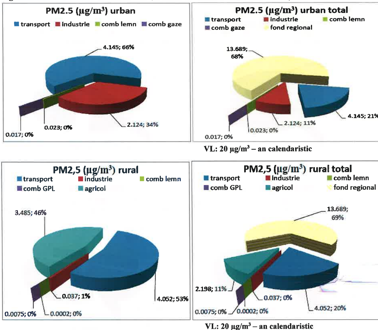
Figura nr. 4-5 Niveluri maxime PM2,5 în Scenariul de bază- Contribuție sectoare economice
