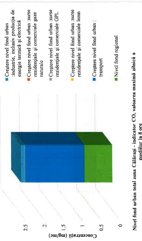
Figura nr. 3-97 Nivel fond urban total – indicator CO
