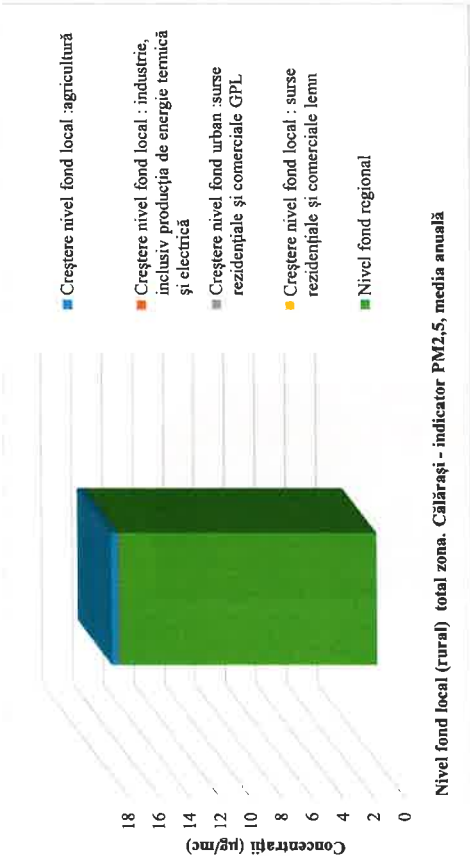
Figura nr. 3-138 Nivel Fond local ( rural) total – indicator PM2,5
