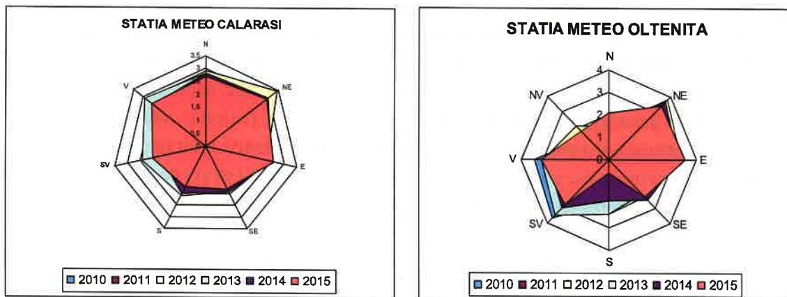
Figura nr. 2-26 Evoluția anuală a vitezei vânturilor la stațiile meteo Călărași și Oltenița
