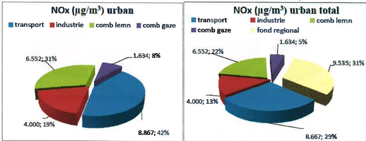
Figura nr. 4-7 Niveluri maxime NO x /NO 2 în Scenariul de bază- Contribuție sectoare economice
