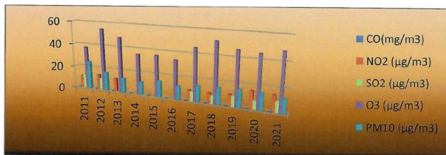
Figura 1.2 Evoluția valorilor măsurate de stația CS-2 Oțelu Roșu în 2011-2021 (medii anuale)
