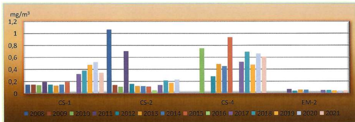
Figura 2.7 Evoluția valorilor măsurate concentrații de CO (medii anuale), în județul Caraș-Severin, mg/m 3
