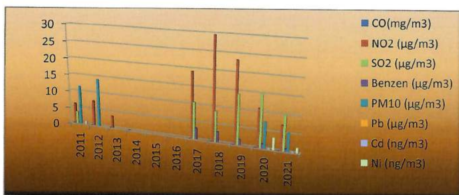
Figura 1.6 Evoluția valorilor măsurate de stația EM-2 Semenici în 2011-2021 (medii anuale)
