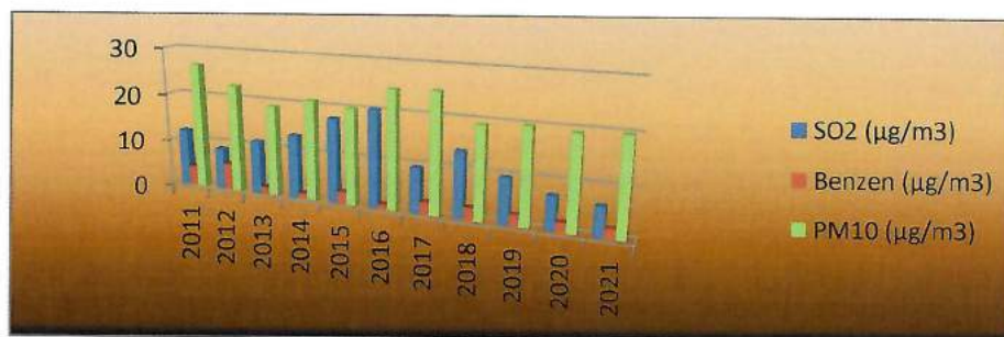
Figura 1.3 Evoluția valorilor măsurate de stația CS-3 Moldova Nouă în 2011-2021 (medii anuale)
