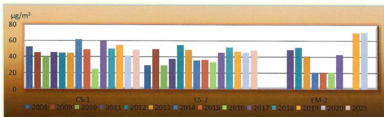
Figura 2.14 Evoluția valorilor măsurate concentrații de \text{O}_3 (medii anuale), în județul Caraș-Severin, \mu\text{g}/\text{m}^3
