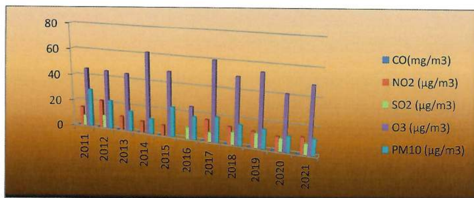
Figura 1.1 Evoluția valorilor măsurate de stația CS-1 Reșița în 2011-2021 (medii anuale)
