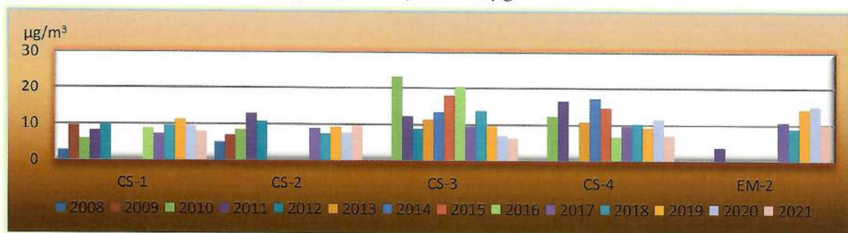
Figura 2.2 Evoluția valorilor măsurate concentrații de \text{SO}_2 (medii anuale), în județul Caraș-Severin, \mu\text{g}/\text{m}^3
