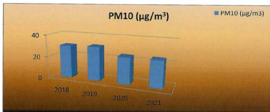
Figura 1.5 Evoluția valorilor măsurate de stația CS-5 Moldova Nouă 2018- 2021 (medii anuale)
