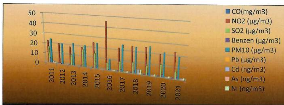
Figura 1.4 Evoluția valorilor măsurate de stația CS-4 Buchin în 2011-2021 (medii anuale)
