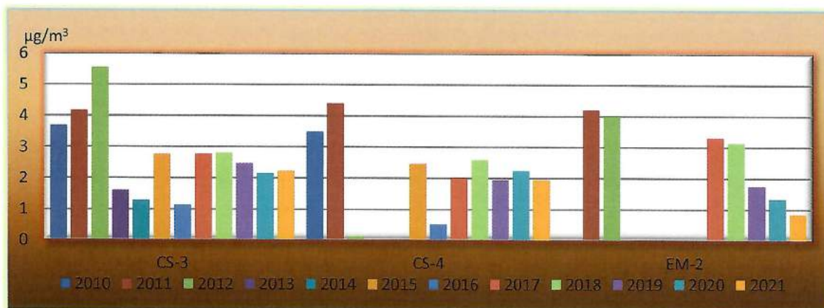
Figura 2.10 Evoluția valorilor măsurate concentrații de benzen (medii anuale), în județul Caraș-Severin, \mu\text{g}/\text{m}^3
