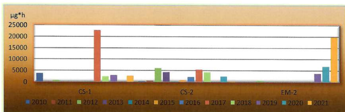
Figura 2.17 Evoluția valorilor ale parametrului AOT40 pentru protecția culturilor agricole, \mu\text{g}\cdot\text{h}
