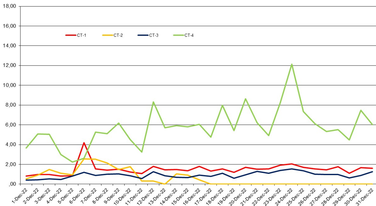
Benzen (ug/m3), perioada: 01 - 31 Decembrie 2022 - Date validate
