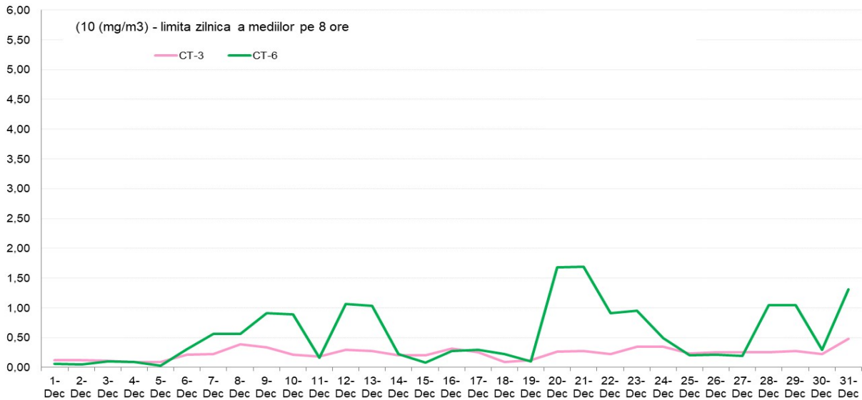
CO (mg/m 3 ) - maximul zilnic medie mobila perioada: 01 - 31 Decembrie 2022 - date validate
