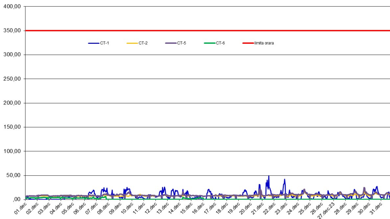
SO 2 (ug/m3), perioada: 01 - 31 Decembrie 2022 - Date validate
