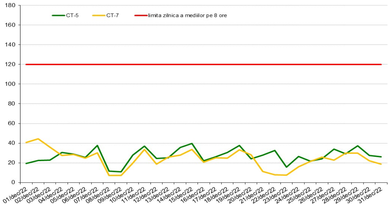
O 3 (mg/m 3 ) - maximul zilnic medie mobila perioada: 01 - 31 Decembrie 2022 - date validate
