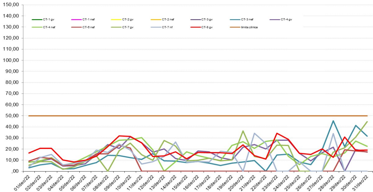
PM10 nef si PM10 gv (ug/m3), perioada: 01 - 31 Decembrie 2022 - Date validate
