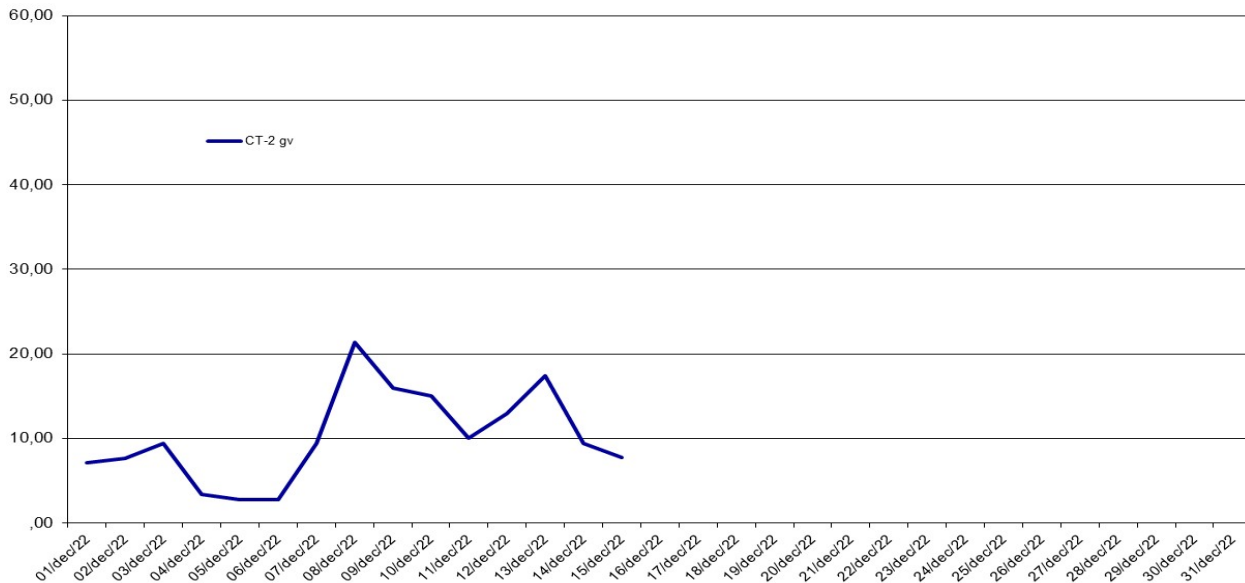
PM2.5 gv (ug/m3), perioada: 01 - 31 Decembrie 2022 - Date validate
