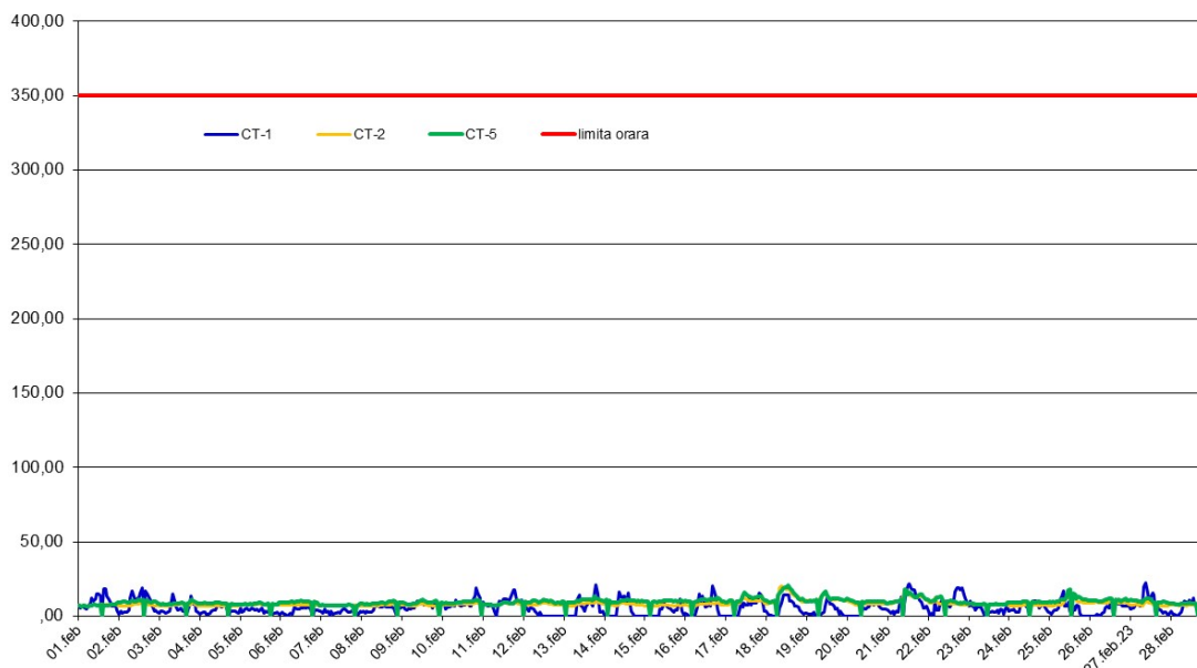
SO2 (ug/m3), perioada: 01 - 28 Februarie 2023 - Date validate
