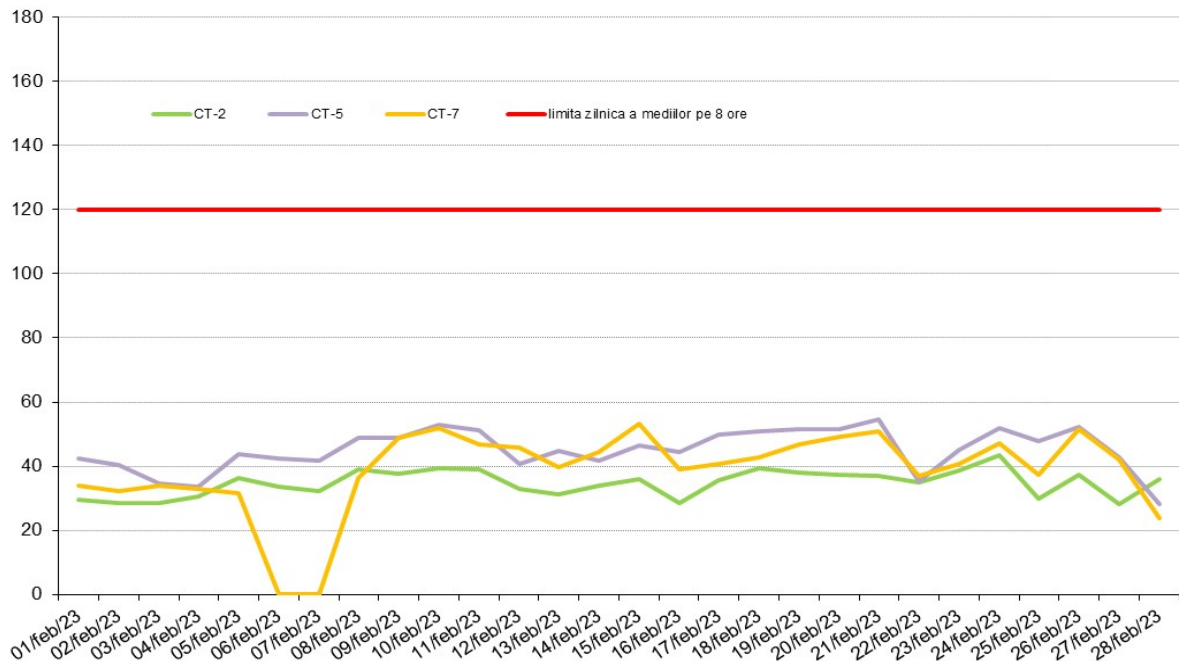
O 3 (mg/m 3 ) - maximul zilnic medie mobila perioada: 01 - 28 Februarie 2023 - date validate
