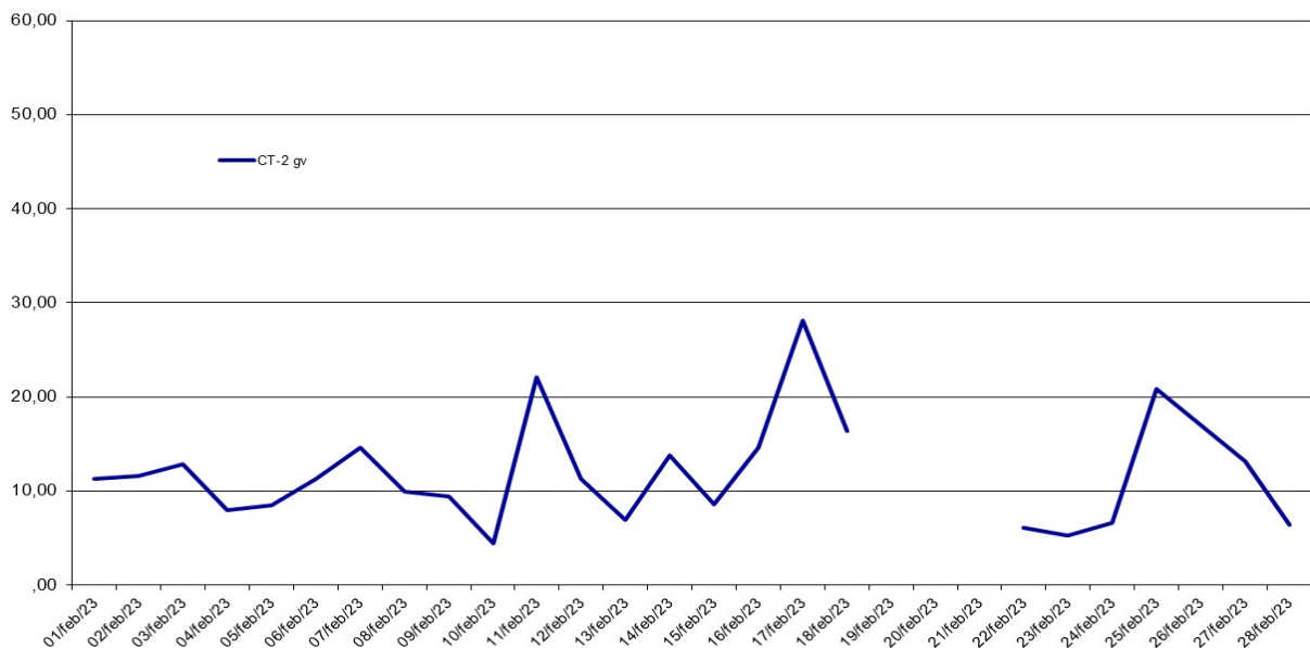
PM2.5 gv ( \mu\text{g}/\text{m}^3 ), perioada: 01 - 28 Februarie 2023 - Date validate
