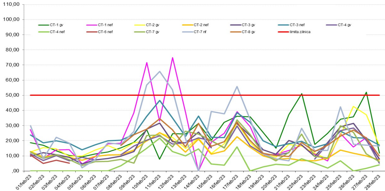
PM10 nef și PM10 gv ( \mu\text{g}/\text{m}^3 ), perioada: 01 - 28 Februarie 2023 - Date validate
