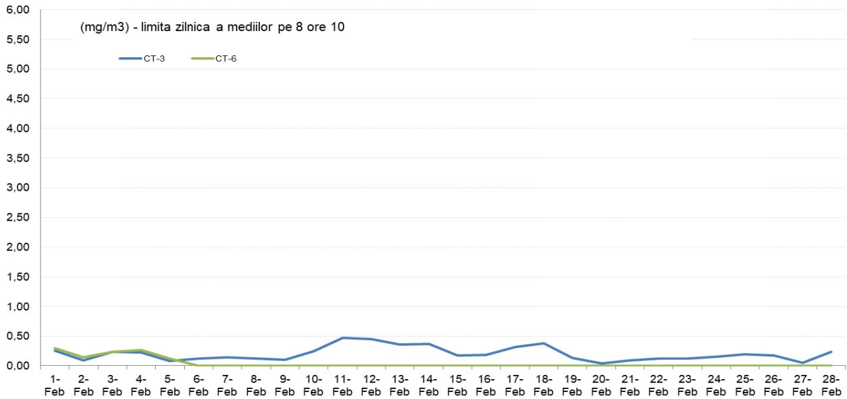
CO (mg/m 3 ) - maximul zilnic medie mobila perioada: 01 - 28 Februarie 2023 - date validate
