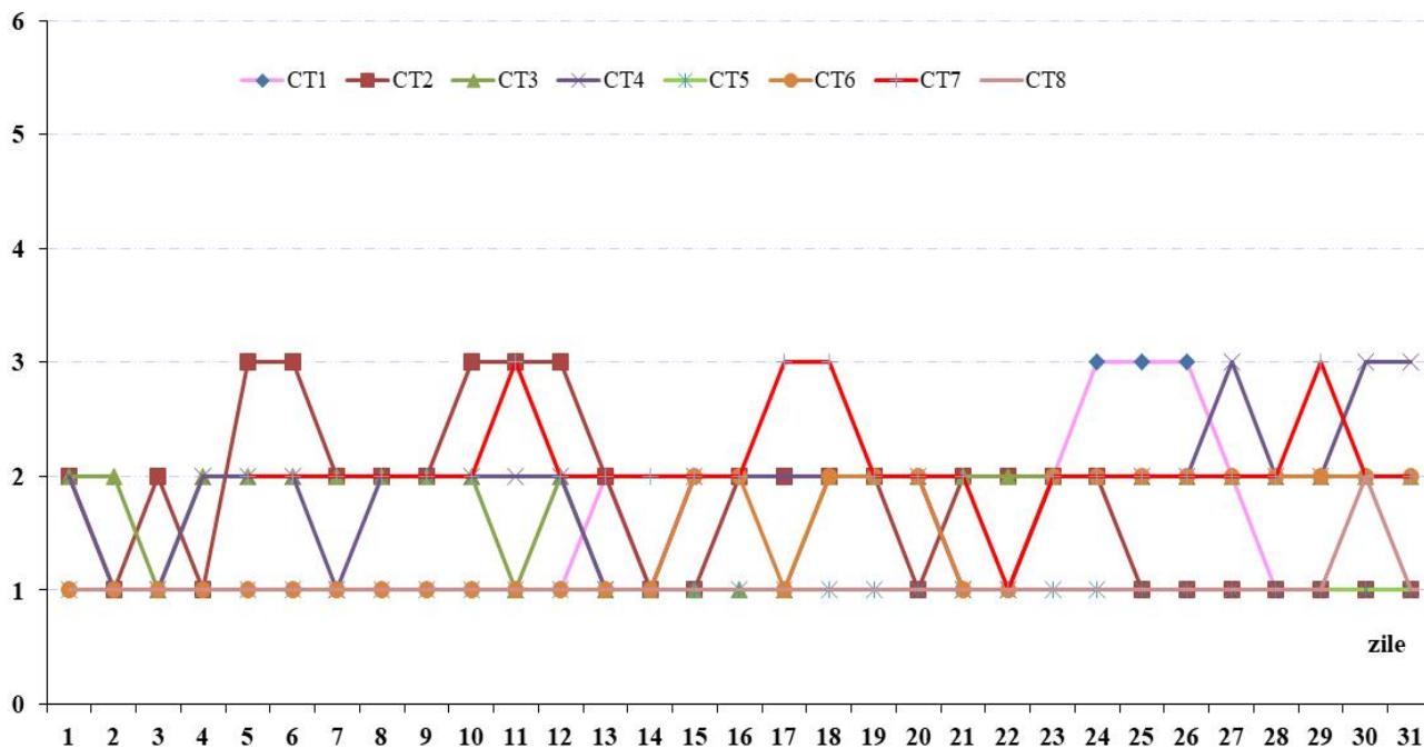
Indici generali - octombrie 2022
