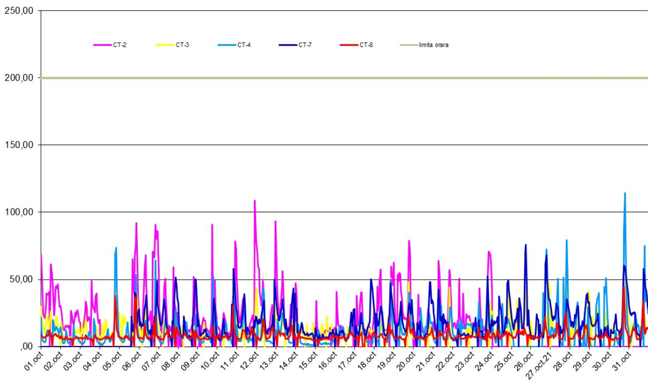
NO2 (ug/m3), perioada: 01 - 31 Octombrie 2022 - Date validate
