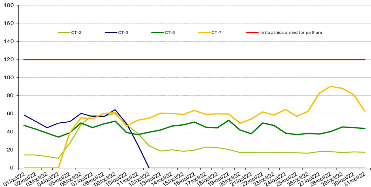
O 3 (mg/m 3 ) - maximul zilnic medie mobila perioada: 01 - 31 Octombrie 2022 - date validate
