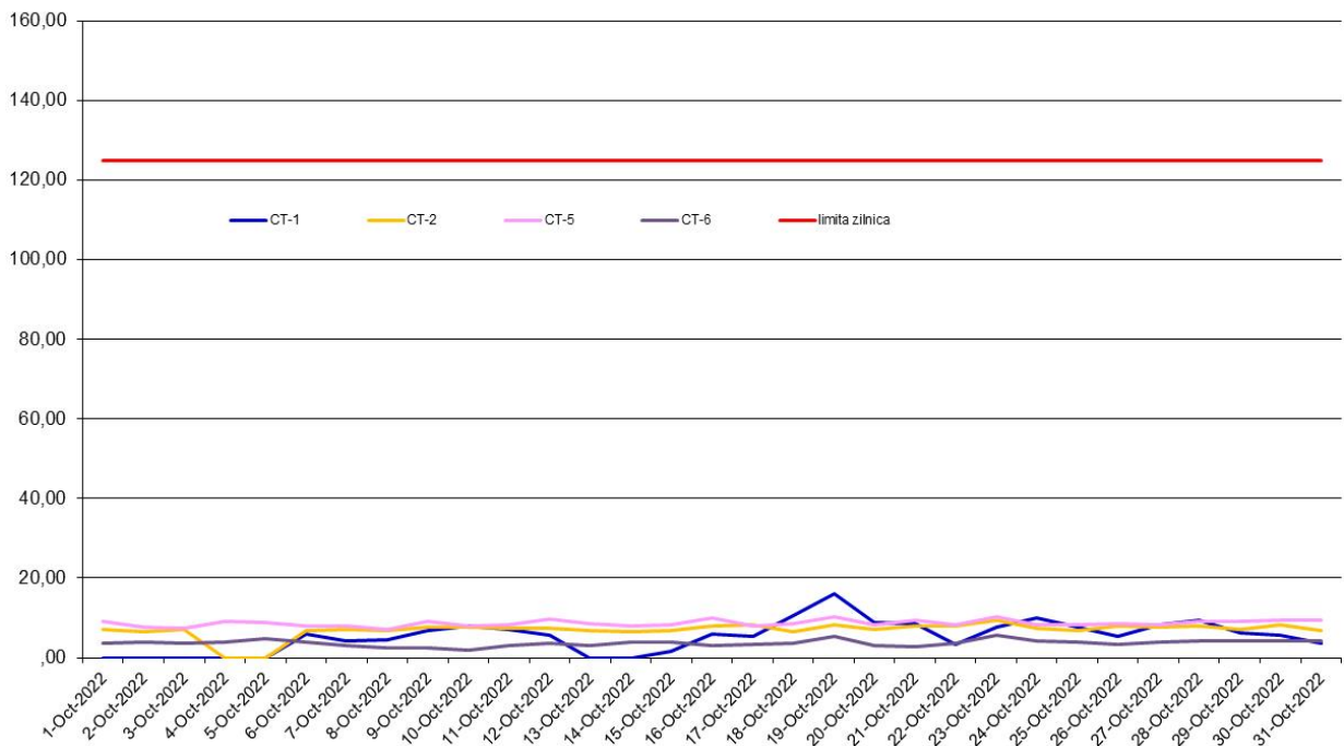
SO2 (ug/m3), perioada: 01 - 31 Octombrie 2022 - Date validate
