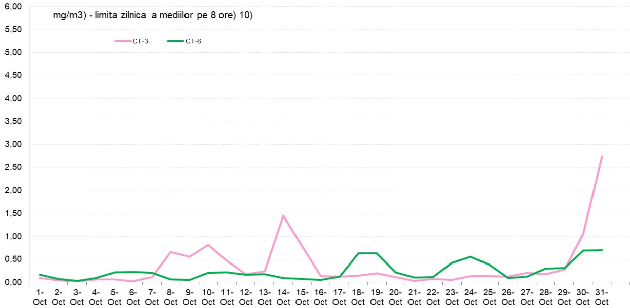
CO (mg/m 3 ) - maximul zilnic medie mobila perioada: 01 - 31 Octombrie 2022 - date validate
