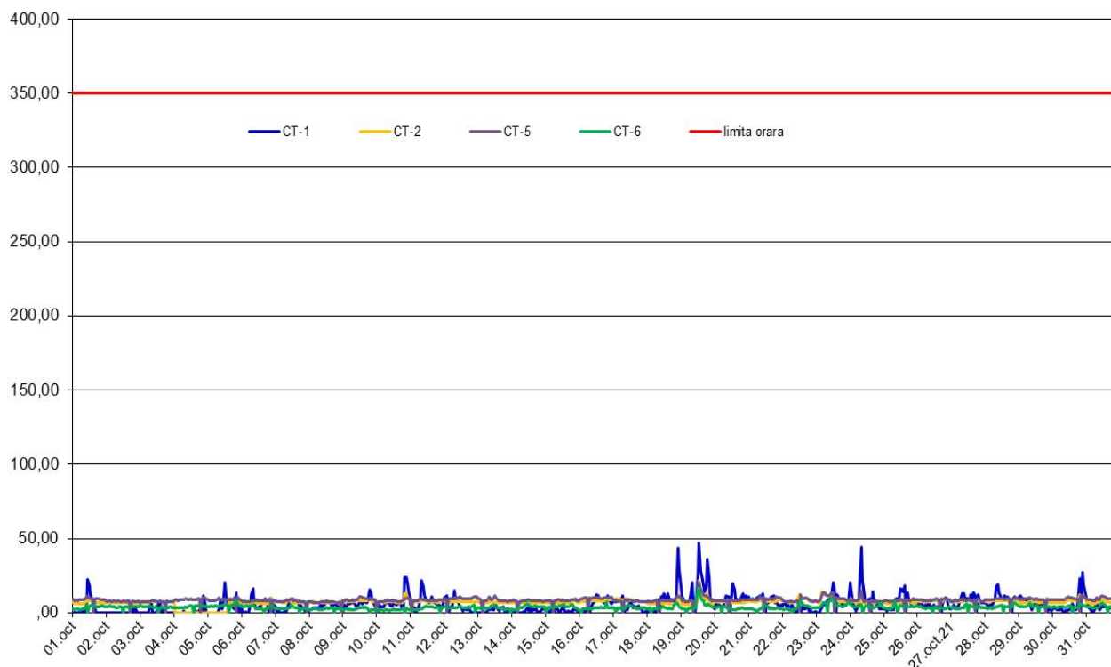
SO 2 (ug/m3), perioada: 01 - 31 Octombrie 2022 - Date validate
