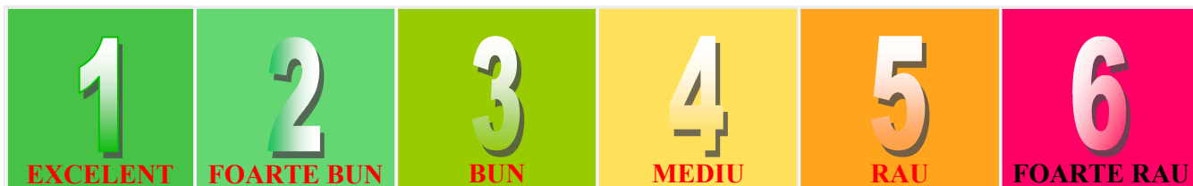
Indici generali - octombrie 2022
