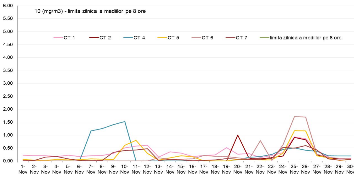
CO (mg/m 3 ) - maximul zilnic medie mobila perioada: 01 Noiembrie - 30 Noiembrie 2018 - date validate
