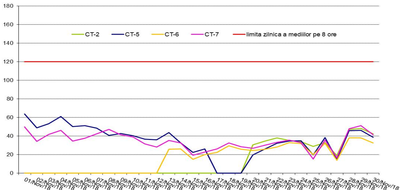
O 3 (mg/m 3 ) - maximul zilnic medie mobila perioada: 01 Noiembrie - 30 Noiembrie 2018 - date validate
