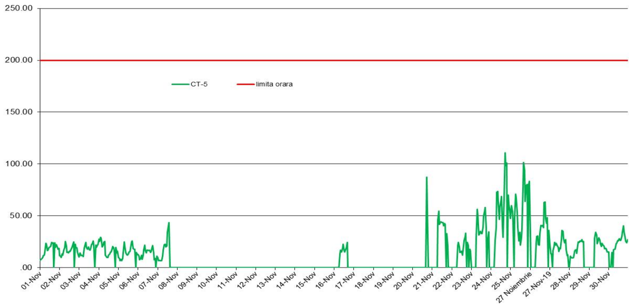
NO2 (ug/m3), perioada: 01 Noiembrie 2018-30 Noiembrie 2018 - Date validate
