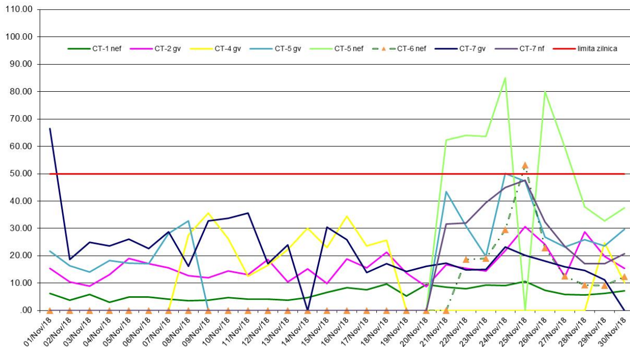
PM10 nef si PM10 gv (ug/m3), perioada: 01 -30 Noiembrie 2018 - Date validate
