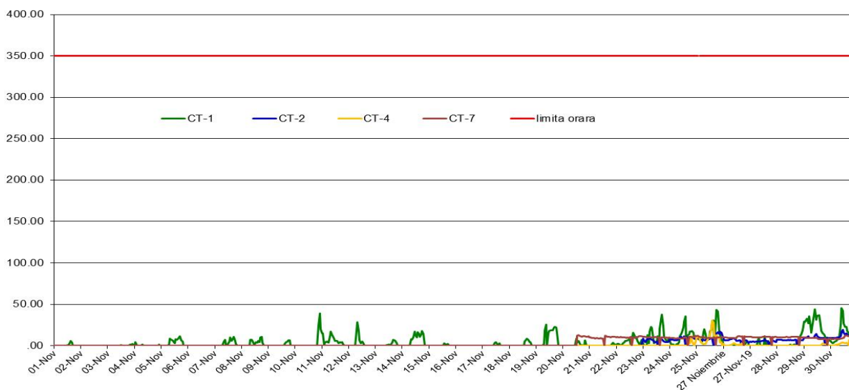
SO 2 (ug/m3), perioada: 01 Noiembrie 2018-30 Noiembrie 2018 - Date validate
