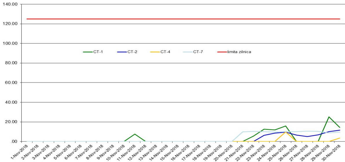
SO2 (ug/m3), perioada: 01 - 30 Noiembrie 2018 - Date validate
