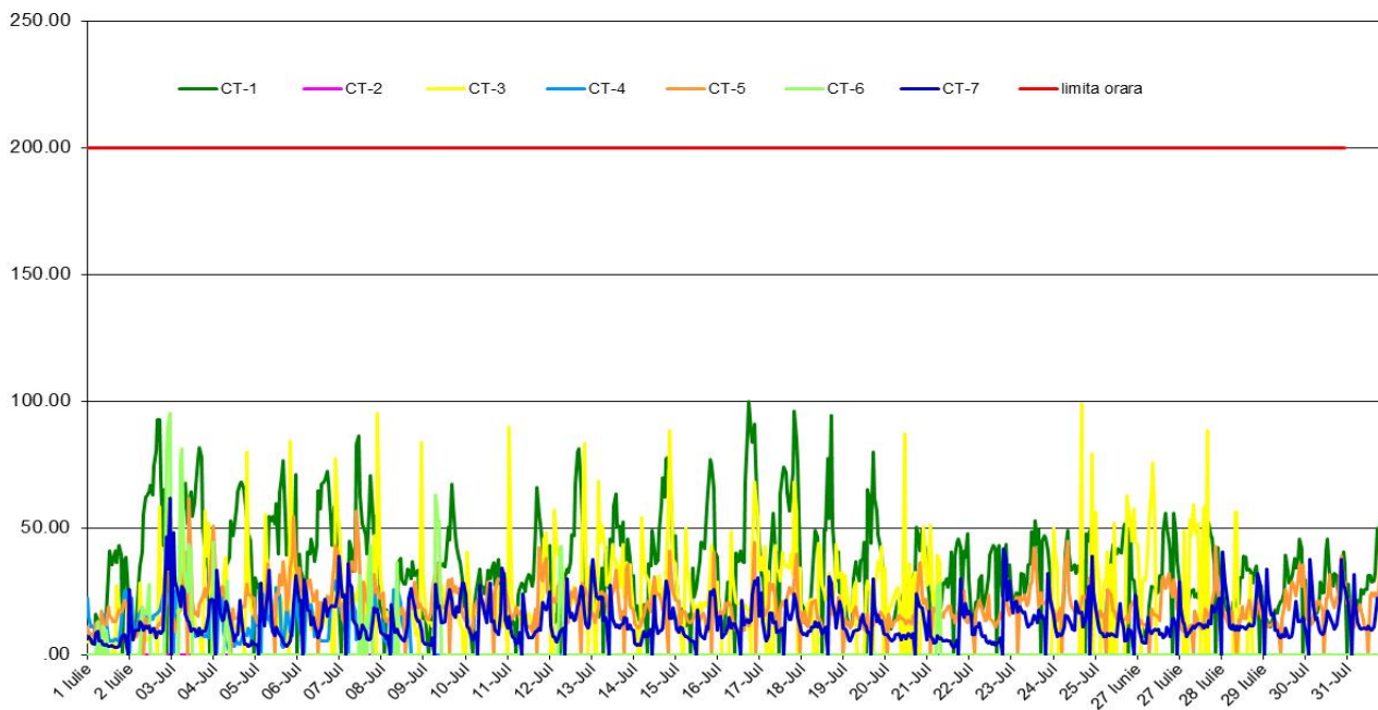
NO2 (ug/m3), perioada: 01 Iulie 2018-31 Iulie 2018 - Date validate
