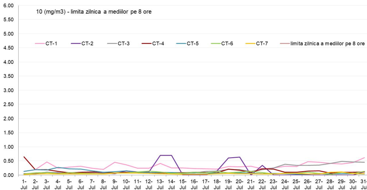
CO (mg/m3) - maximul zilnic medie mobila perioada: 01 Iulie - 31 Iulie 2018 - date validate
