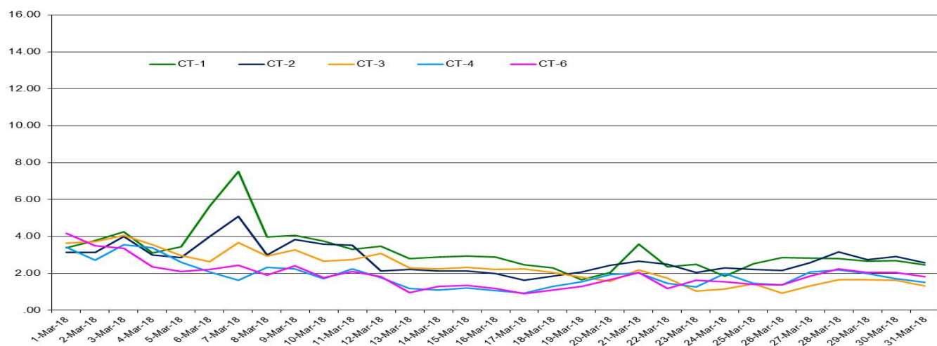
Benzen (ug/m3), perioada: 01 - 31 Martie 2018 - Date validate
