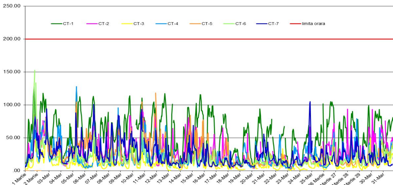
NO 2 ( \mu\text{g}/\text{m}^3 ), perioada: 01 Martie 2018-31 Martie 2018 - Date validate
