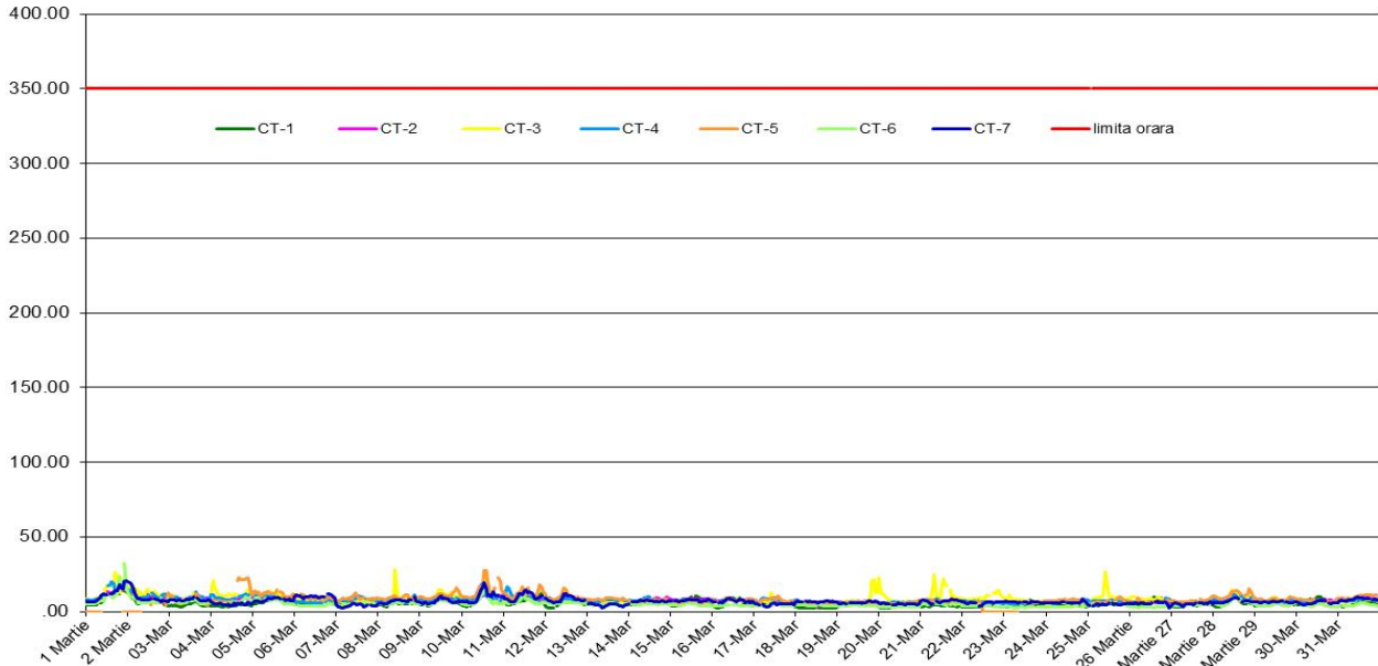
SO 2 (ug/m3), perioada: 01 Martie 2018-31 Martie 2018 - Date validate
