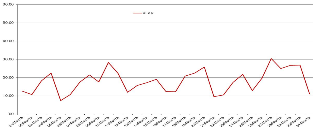
PM2.5 gv (ug/m3), perioada: 01 -31 Martie 2018 - Date validate
