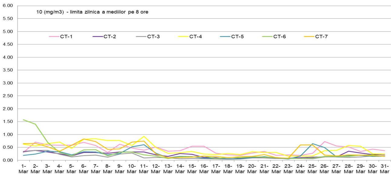
CO ( \text{mg}/\text{m}^3 ) - maximul zilnic medie mobila perioada: 01 Martie - 31 Martie 2018 - date validate
