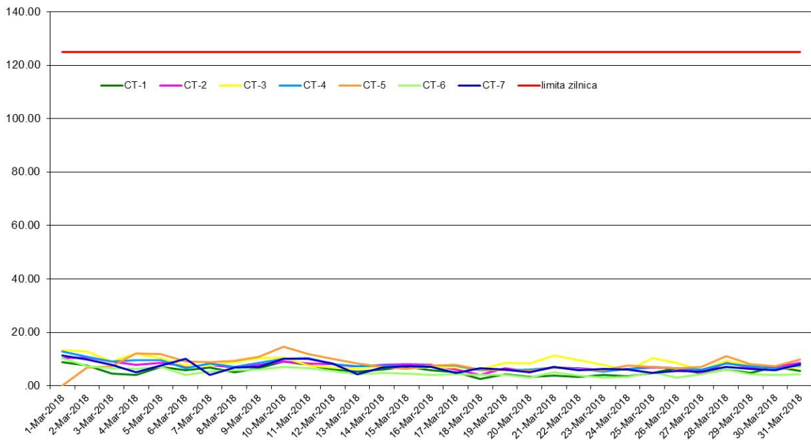
SO 2 (ug/m3), perioada: 01 Martie 2018-31 Martie 2018 - Date validate
