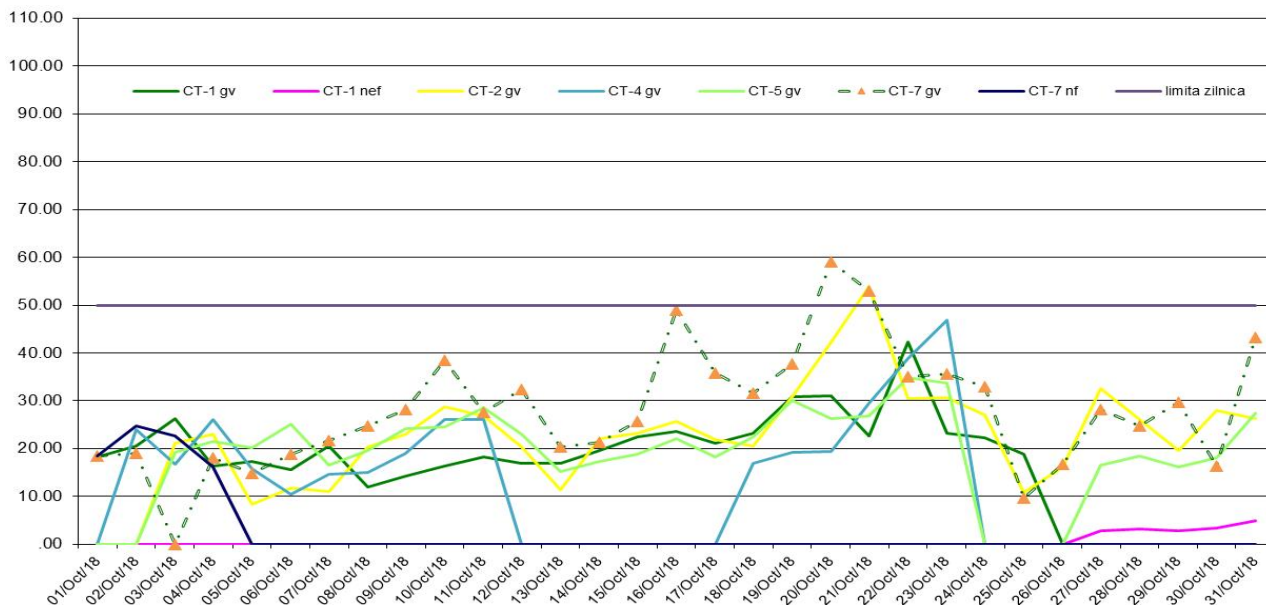
PM10 nef și PM10 gv ( \mu\text{g}/\text{m}^3 ), perioada: 01 -31 Octombrie 2018 - Date validate
