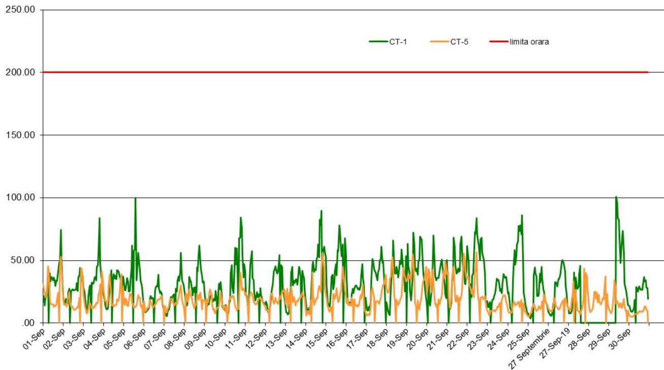
NO2 (ug/m3), perioada: 01 Septembrie 2018-30 Septembrie 2018 - Date validate
