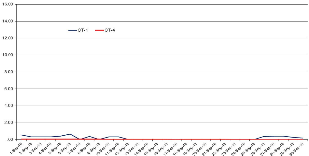
Benzen (ug/m3), perioada: 01 - 30 Septembrie 2018 - Date validate
