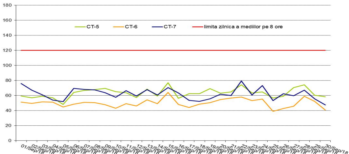
O 3 (mg/m 3 ) - maximul zilnic medie mobila perioada: 01 Septembrie - 30 Septembrie 2018 - date validate
