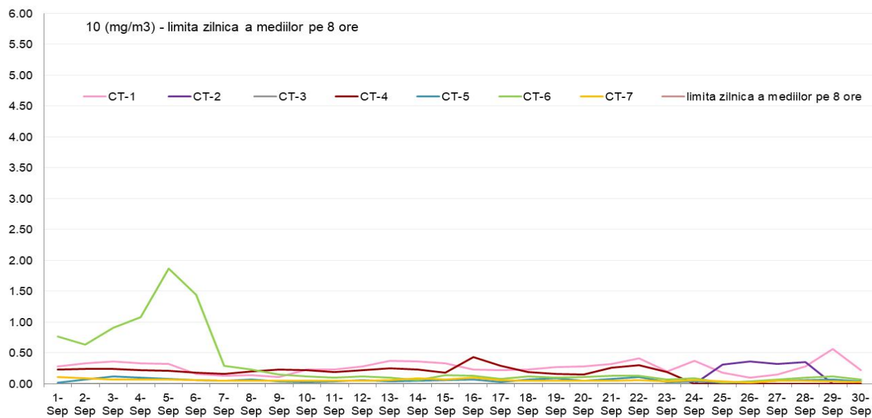
CO (mg/m3) - maximul zilnic medie mobila perioada: 01 Septembrie - 30 Septembrie 2018 - date validate
