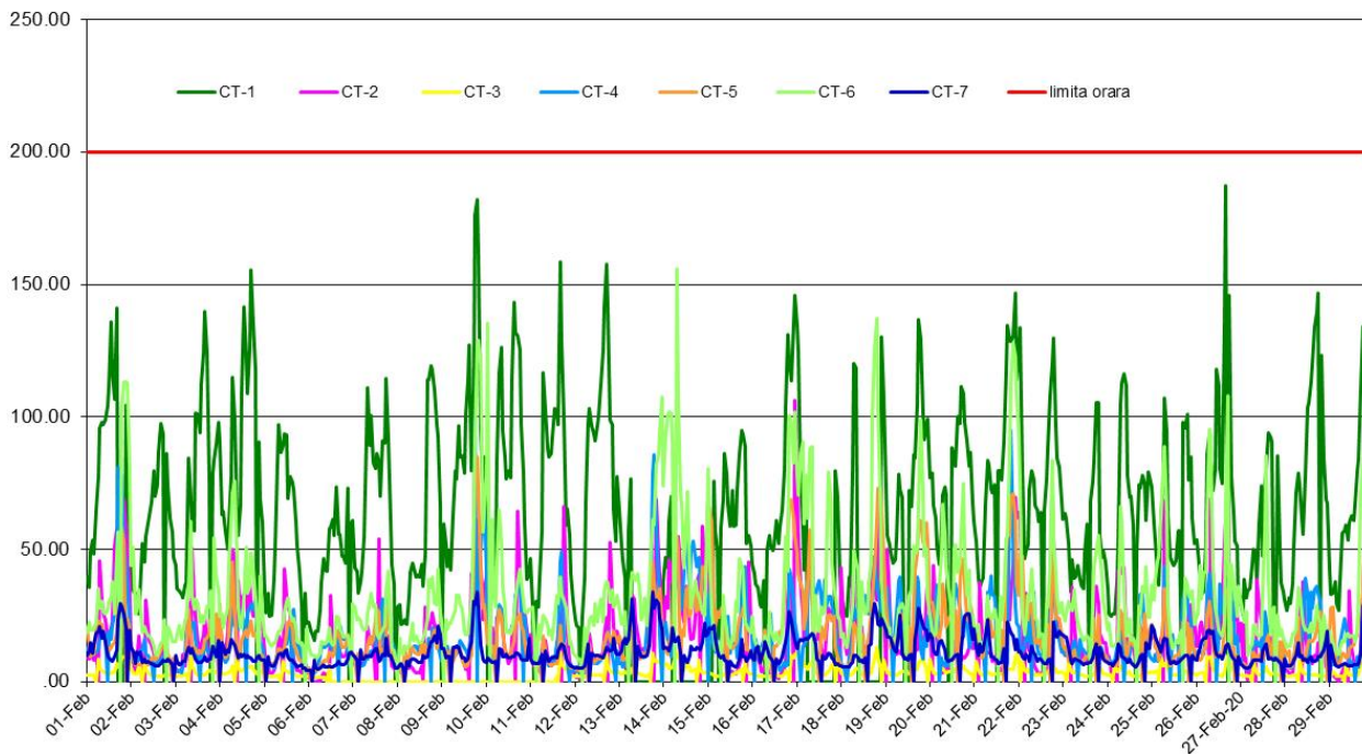
NO2 (ug/m3), perioada: 01 - 29 Februarie 2020 - Date validate
