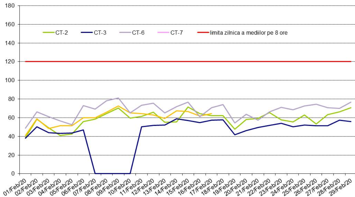
O 3 (mg/m 3 ) - maximul zilnic medie mobila perioada: 01 - 29 Februarie 2020 - date validate
