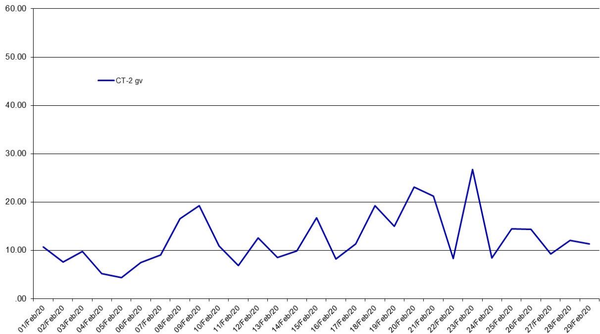
PM2.5 gv (ug/m3), perioada: 01 - 29 Februarie 2020 - Date validate
