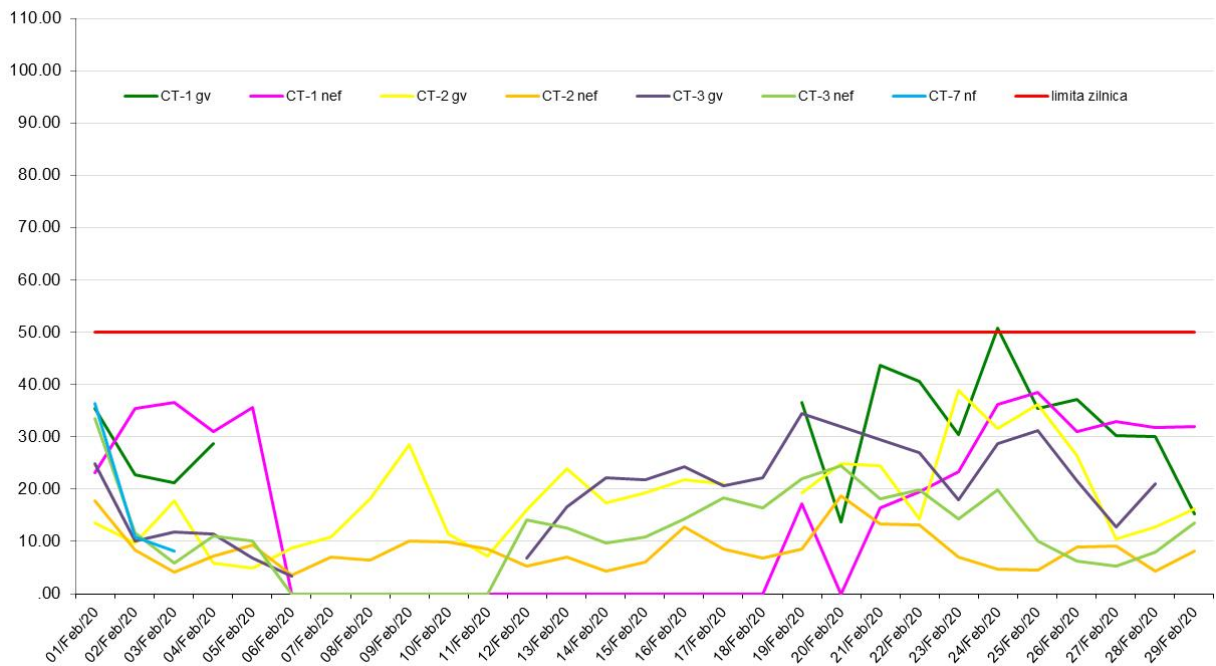
PM10 nef si PM10 gv (ug/m3), perioada: 01 - 29 Februarie 2020 - Date validate
