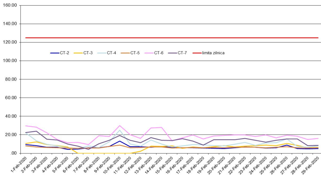
SO 2 (ug/m 3 ), perioada: 01 - 29 Februarie 2020 - Date validate
