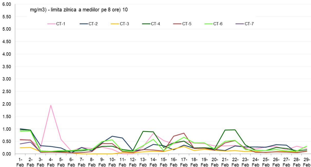
CO (mg/m3) - maximul zilnic medie mobila perioada: 01 - 29 Februarie 2020 - date validate
