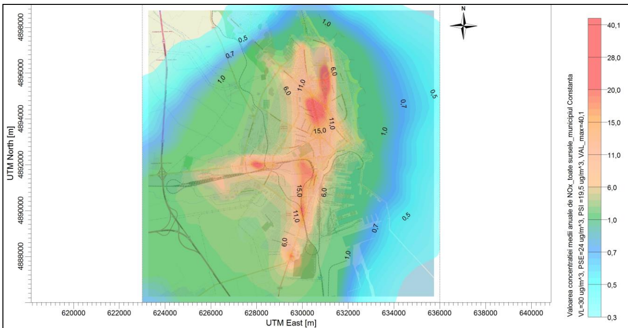
Figura nr.5.18 Concentrația anuală de NO x pentru toate sursele
