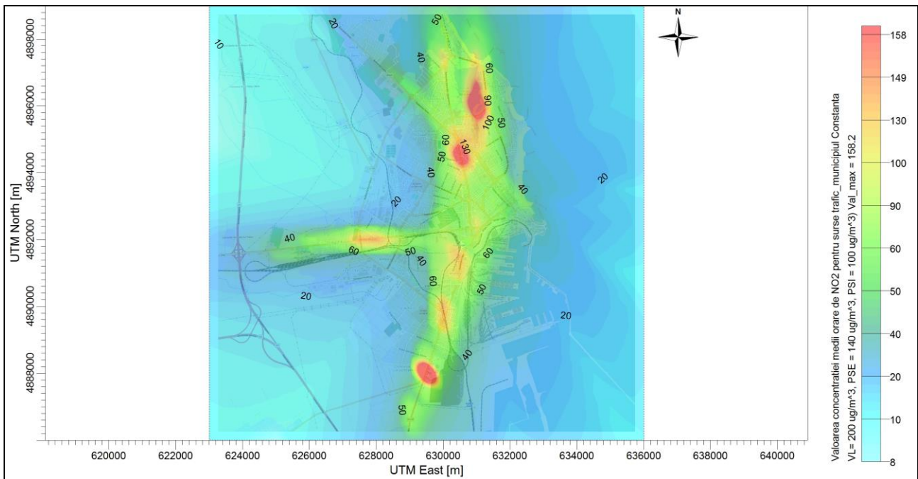
Figura nr.5.14 Concentrația orară de NO 2 pentru sursele liniare
