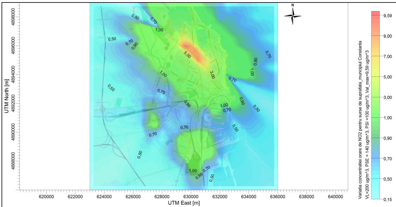
Figura nr.5.17 Concentrația medie orară de NO 2 pentru sursele de suprafață
