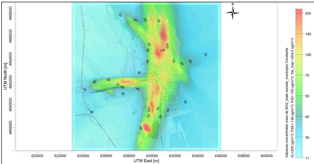
Figura nr.5.20 Concentrația medie orară de NO 2 pentru toate sursele
