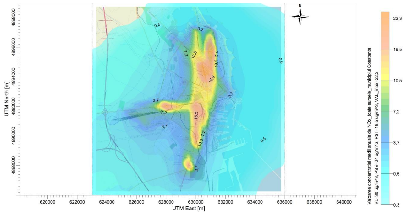
Figura nr.5.30 Concentrația anuală de NO x pentru toate sursele
