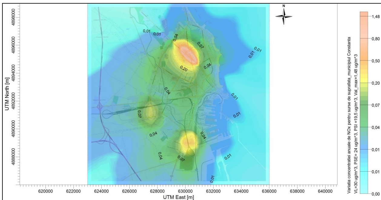
Figura nr.5.27 Concentrația anuală de NO x pentru sursele de suprafață
