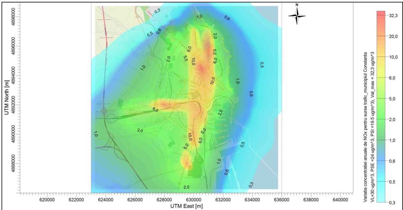
Figura nr.5.12 Concentrația anuală de NO x pentru sursele liniare
