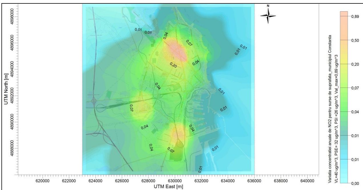
Figura nr.5.28 Concentrația anuală de NO 2 pentru sursele de suprafață
