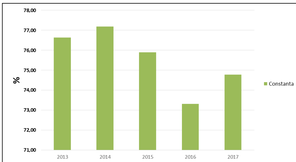
Figura nr. 2. 8 Variația umidității relative medii anuale
