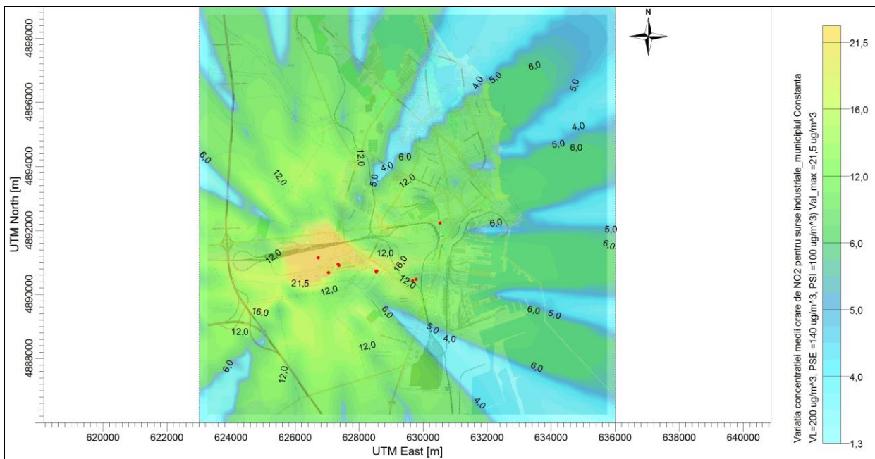
Figura nr.5.23 Concentrația orară de NO 2 pentru sursele industriale
