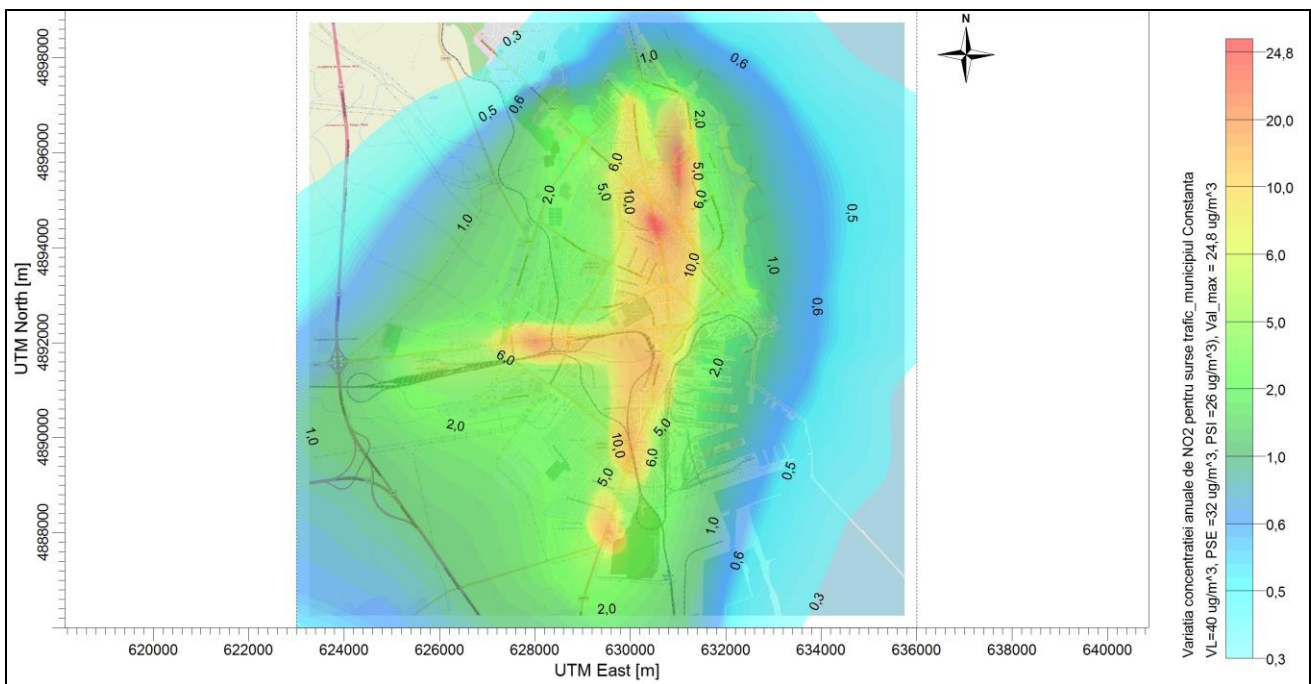
Figura nr.5.13 Concentrația anuală de NO 2 pentru sursele liniare
