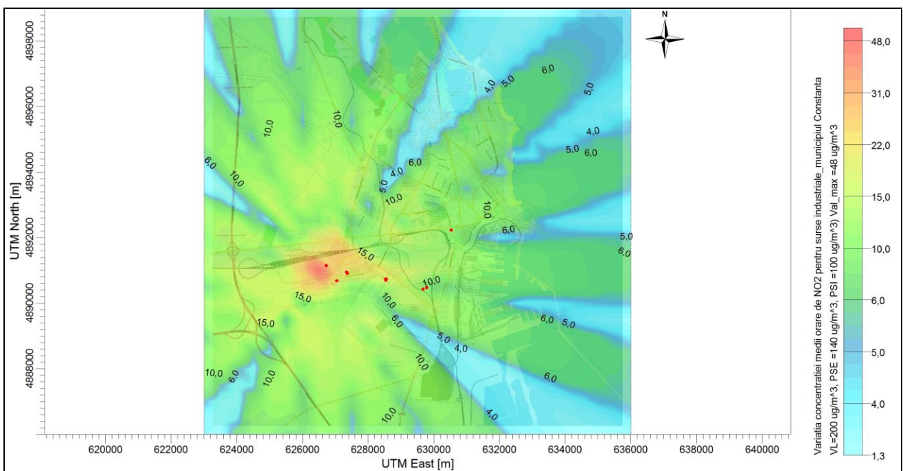
Figura nr.5.11 Concentrația orară de NO 2 pentru sursele industriale
