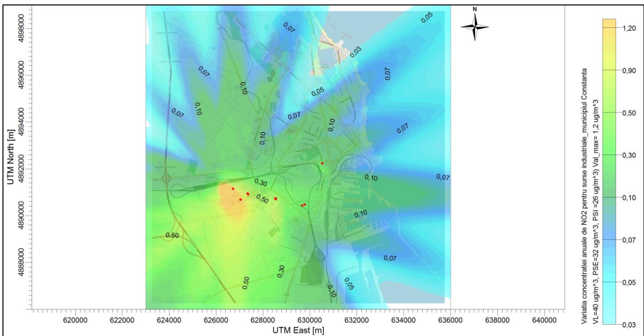
Figura nr.5.22 Concentrația anuală de NO 2 pentru sursele industriale
