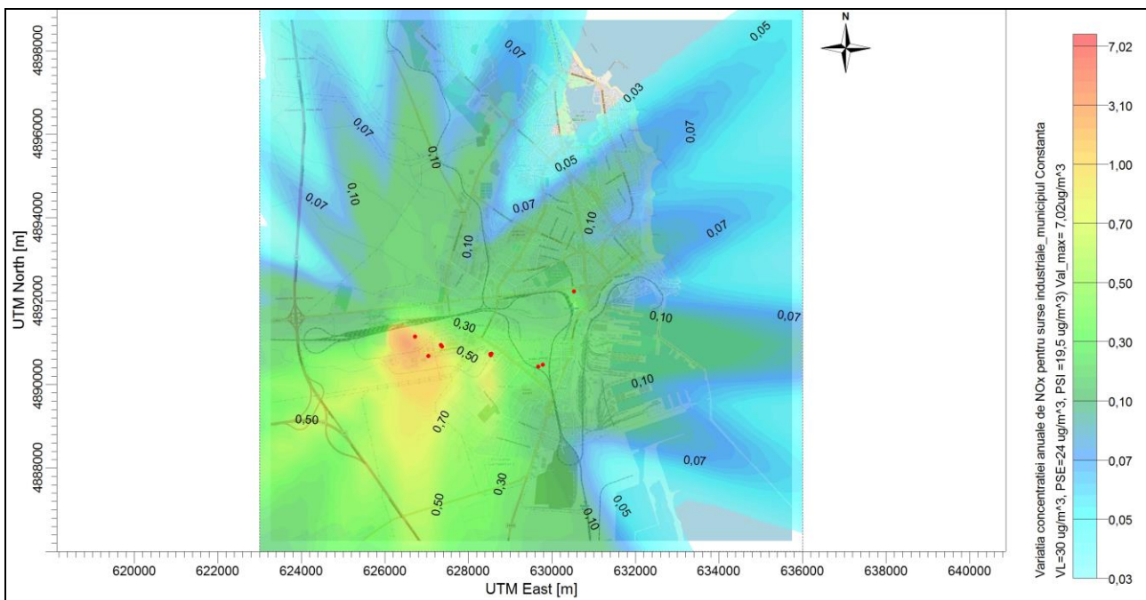
Figura nr.5.9 Concentrația anuală de NO x pentru sursele industriale
