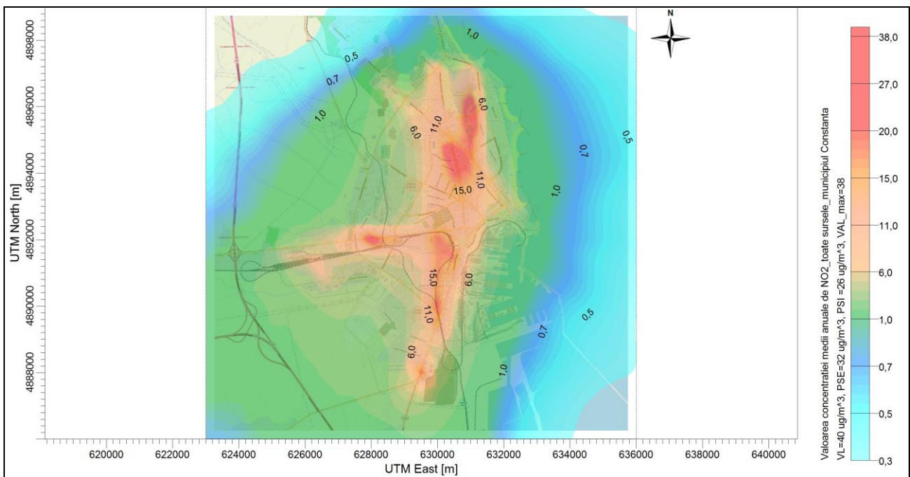
Figura nr.5.19 Concentrația anuală de NO 2 pentru toate sursele
