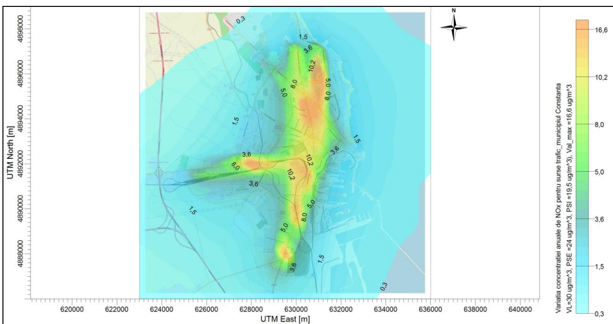
Figura nr.5.24 Concentrația anuală de NO x pentru sursele liniare
