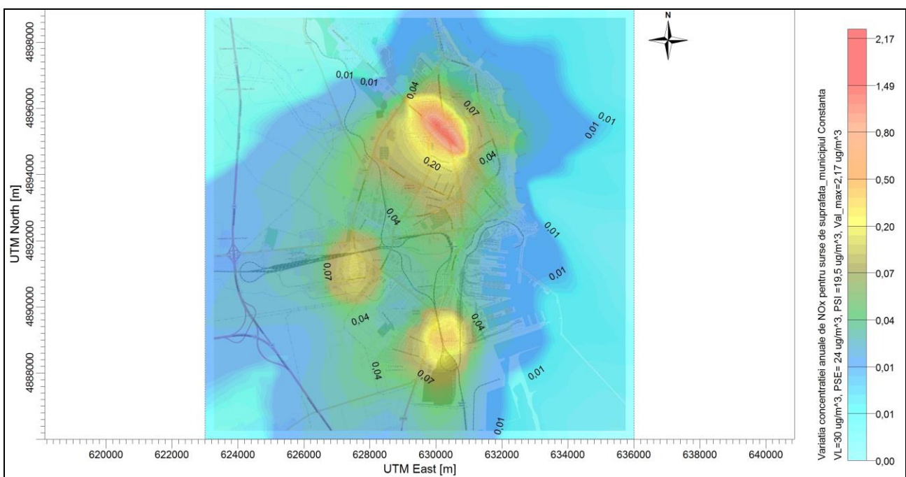
Figura nr.5.15 Concentrația anuală de NO x pentru sursele de suprafață
