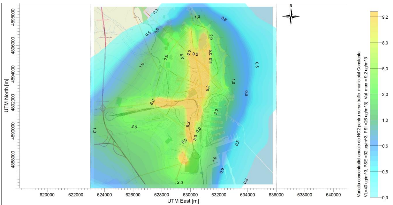
Figura nr.5.25 Concentrația anuală de NO 2 pentru sursele liniare
