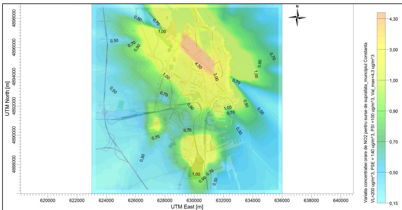
Figura nr.5.29 Concentrația medie orară de NO 2 pentru sursele de suprafață
