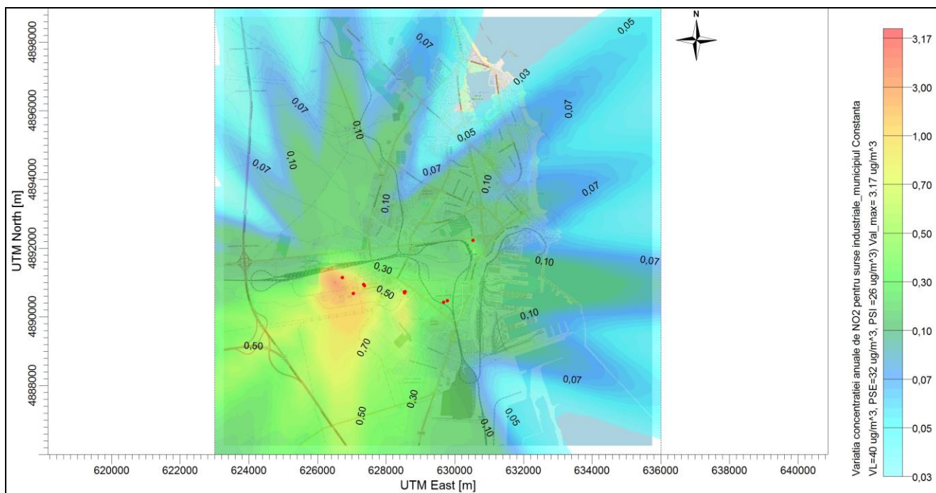
Figura nr.5.10 Concentrația anuală de NO 2 pentru sursele industriale
