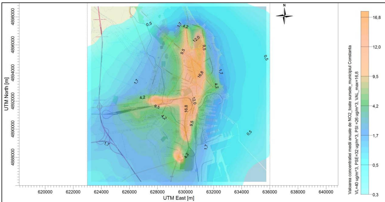
Figura nr.5.31 Concentrația anuală de NO 2 pentru toate sursele
