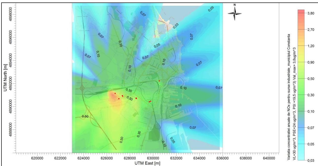
Figura nr.5.21 Concentrația anuală de NO x pentru sursele industriale
