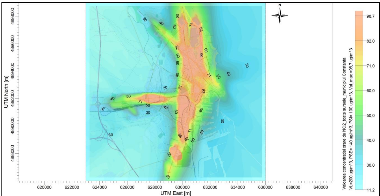
Figura nr.5.32 Concentrația medie orară de NO 2 pentru toate sursele
