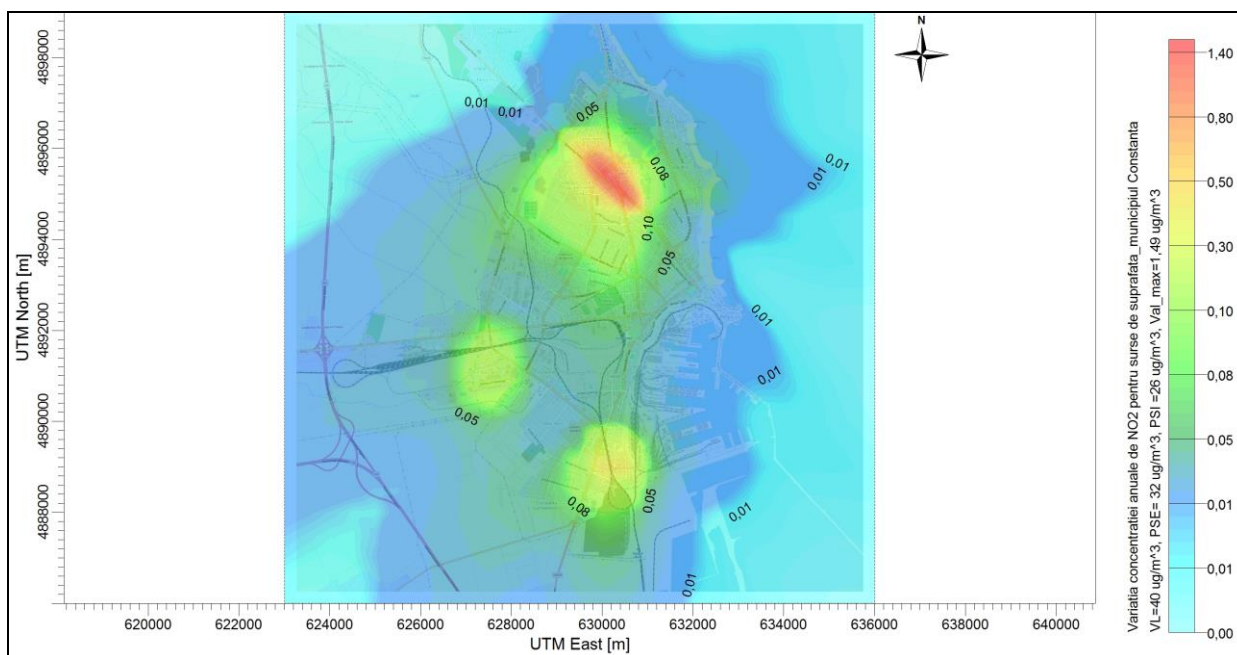
Figura nr.5.16 Concentrația anuală de NO 2 pentru sursele de suprafață
