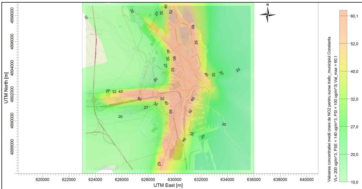
Figura nr.5.26 Concentrația orară de NO 2 pentru sursele liniare
