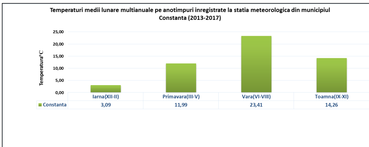
Figura nr. 2. 3 Variația temperaturii medii lunare pe anotimpuri
