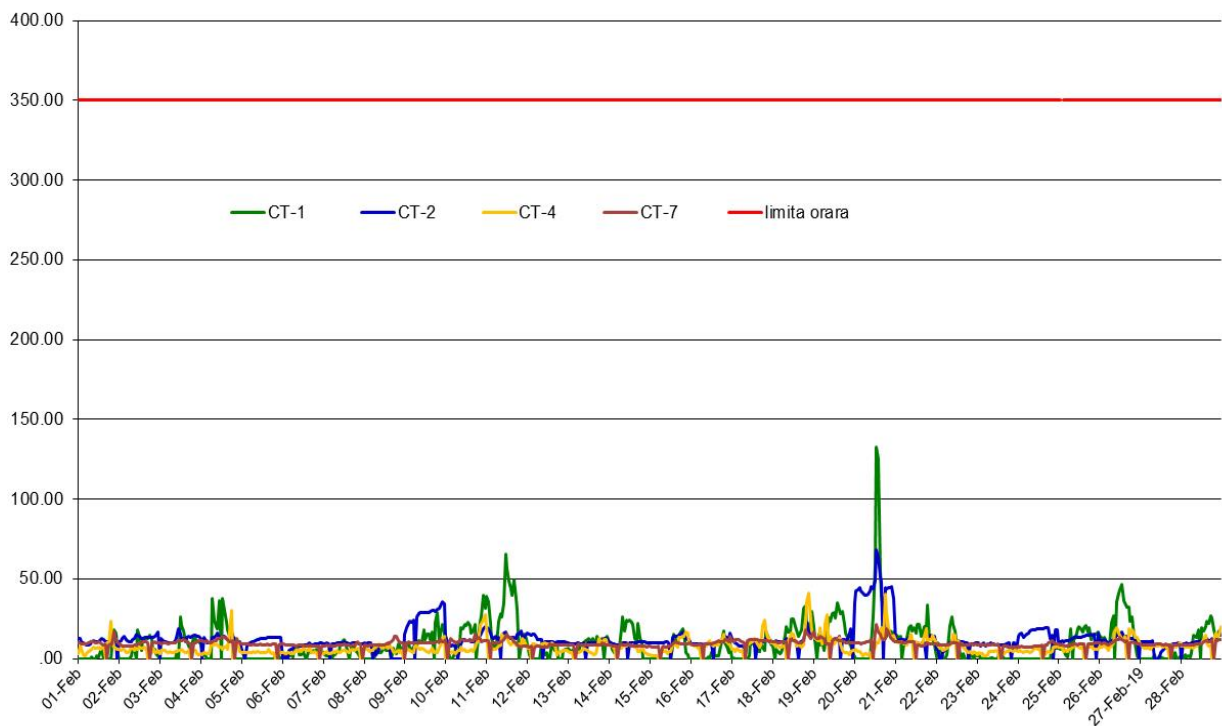
SO 2 (ug/m3), perioada: 01 Februarie 2019-28 Februarie 2019 - Date validate
