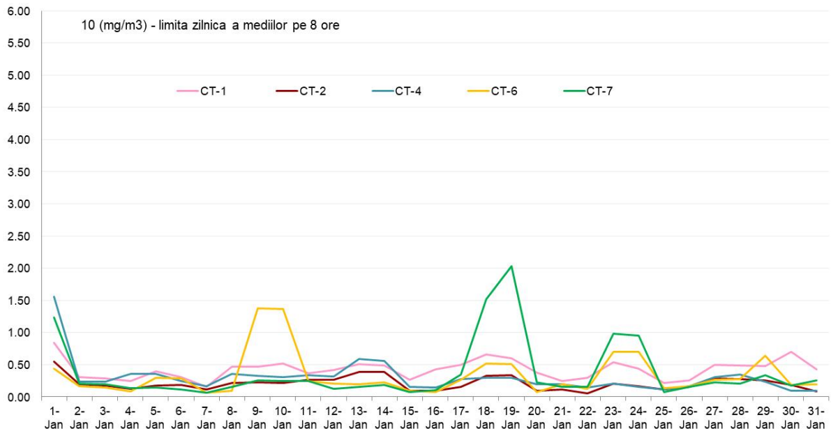
CO (mg/ m3) - maximul zilnic medie mobila perioada: 01 Ianuarie - 31 Ianuarie 2019 - date validate
