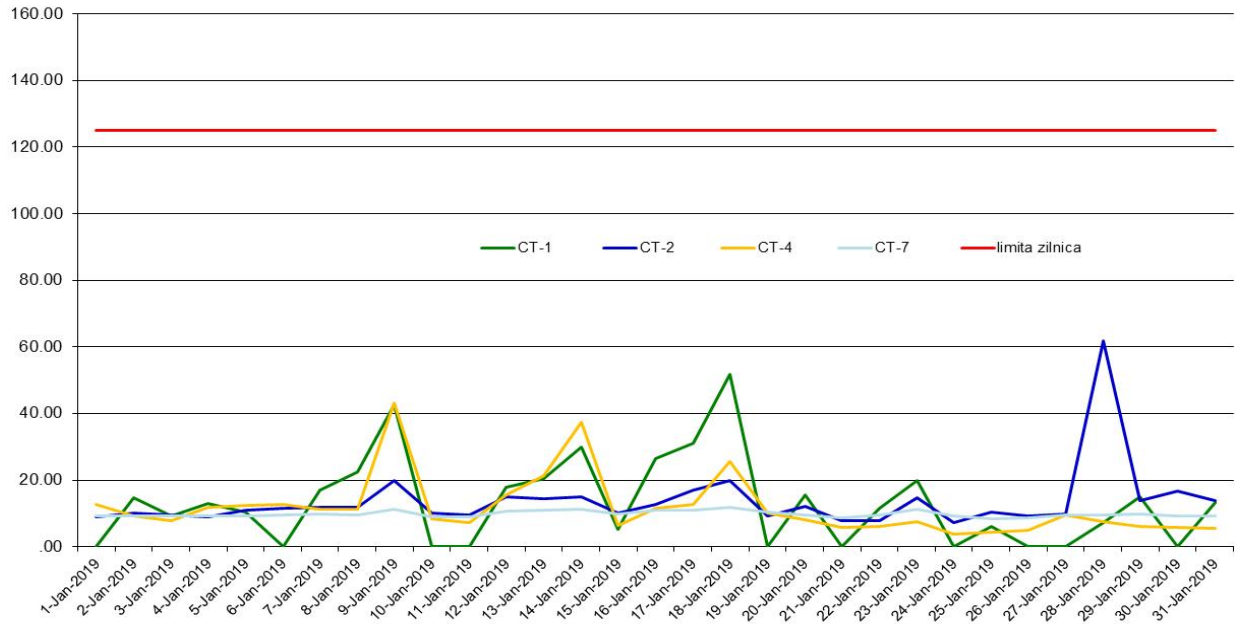
SO2 (ug/m3), perioada: 01 - 31 Ianuarie 2019 - Date validate
