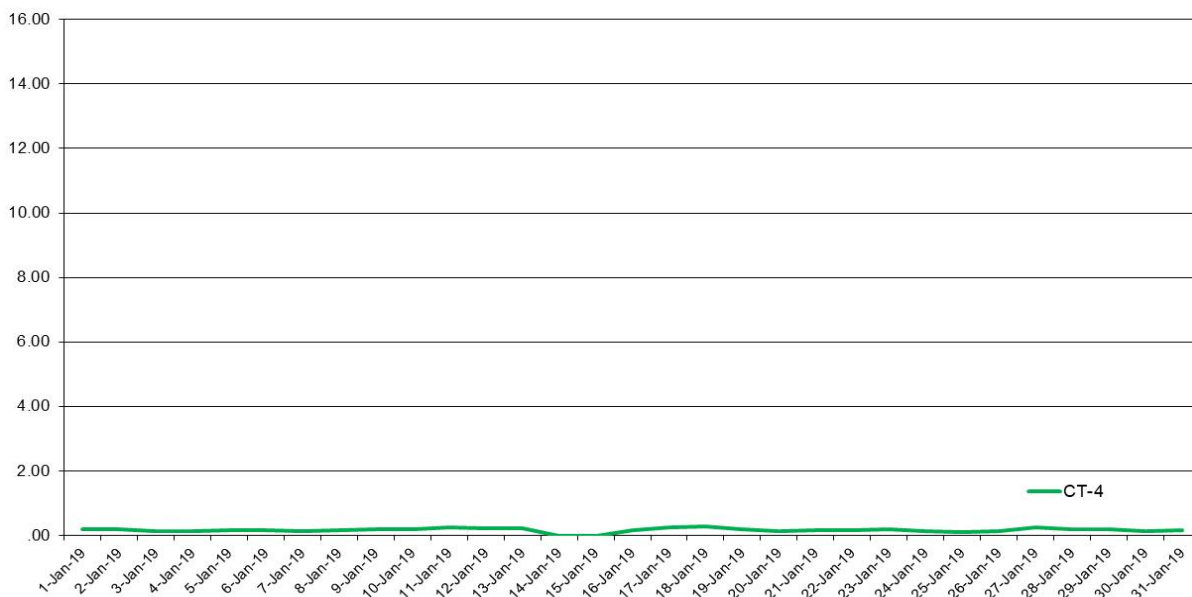
Benzen (ug/m3), perioada: 01 - 31 Ianuarie 2019 - Date validate
