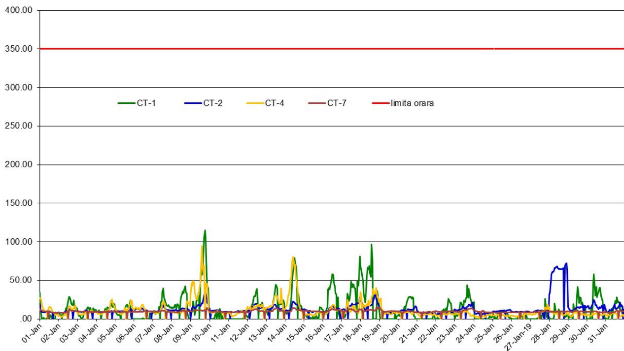
SO2 (ug/m3), perioada: 01 Ianuarie 2019-31 Ianuarie 2019 - Date validate
