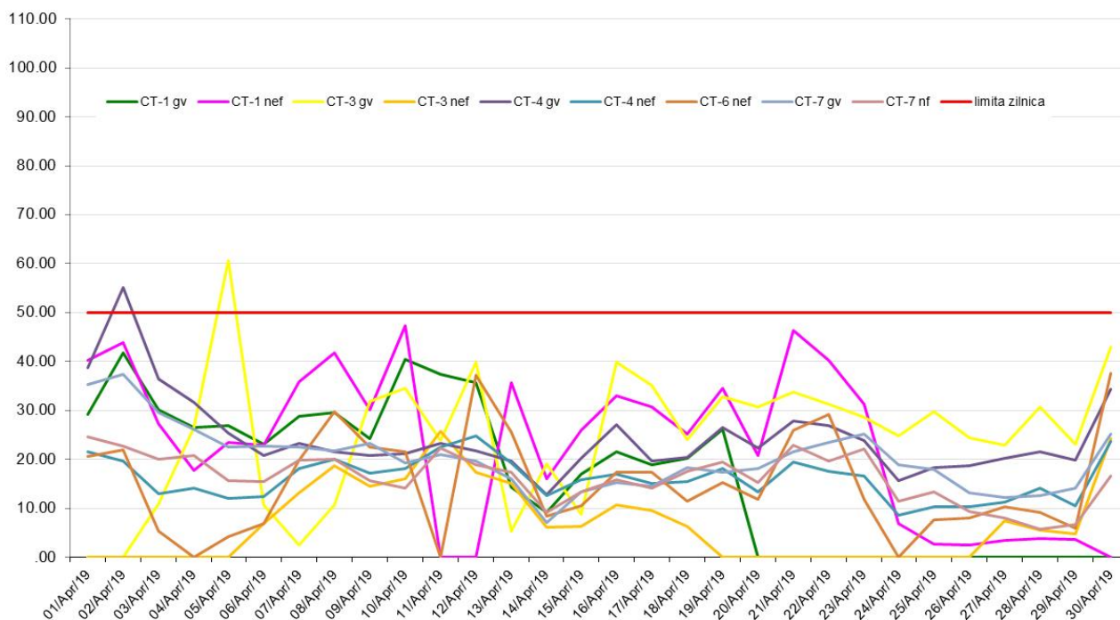
PM10 nef si PM10 gv (ug/m3), perioada: 01 -30 Aprilie 2019 - Date validate
