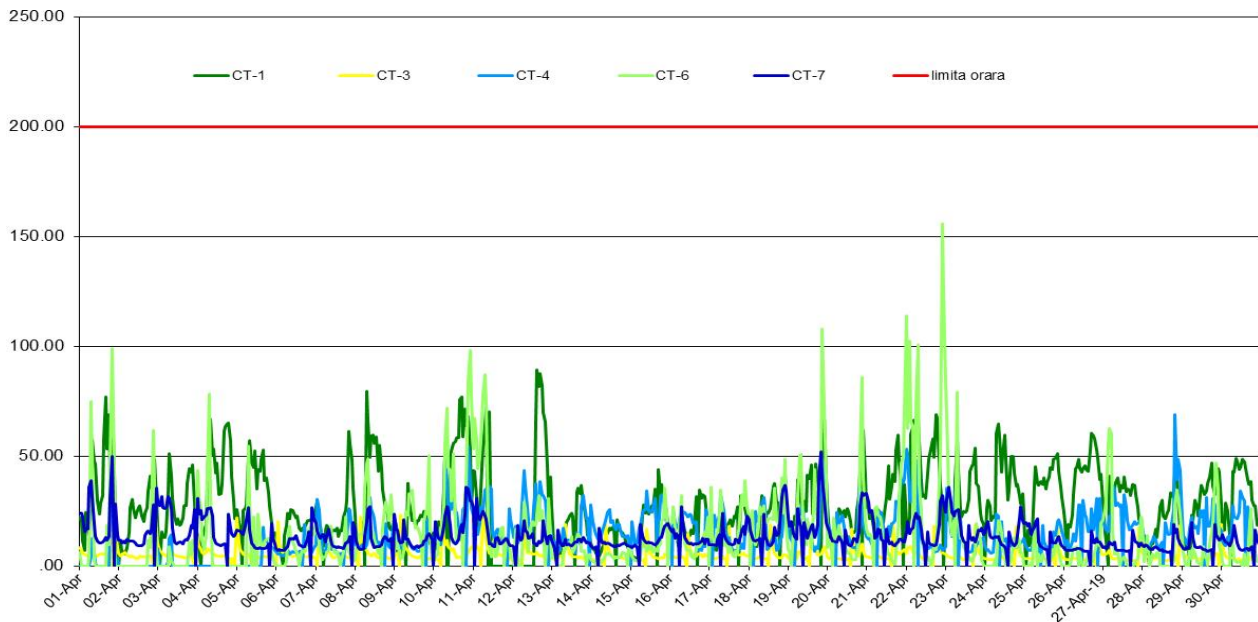
NO2 (ug/m3), perioada: 01 Aprilie 2019 - 30 Aprilie 2019 - Date validate
