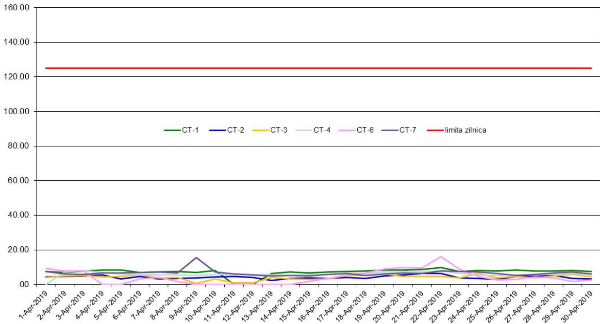
SO2 (ug/m3), perioada: 01 - 30 Aprilie 2019 - Date validate
