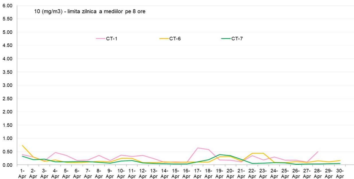
CO (mg/m 3 ) - maximul zilnic medie mobila perioada: 01 Aprilie - 30 Aprilie 2019 - date validate
