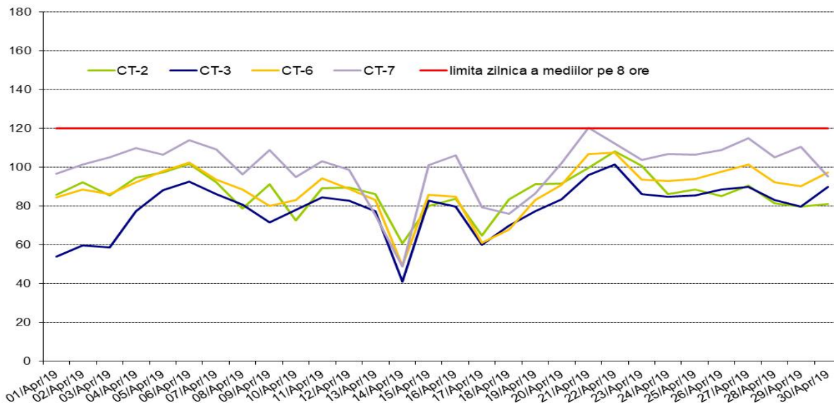
O 3 (mg/m 3 ) - maximul zilnic medie mobila perioada: 01 Aprilie - 30 Aprilie 2019 - date validate
