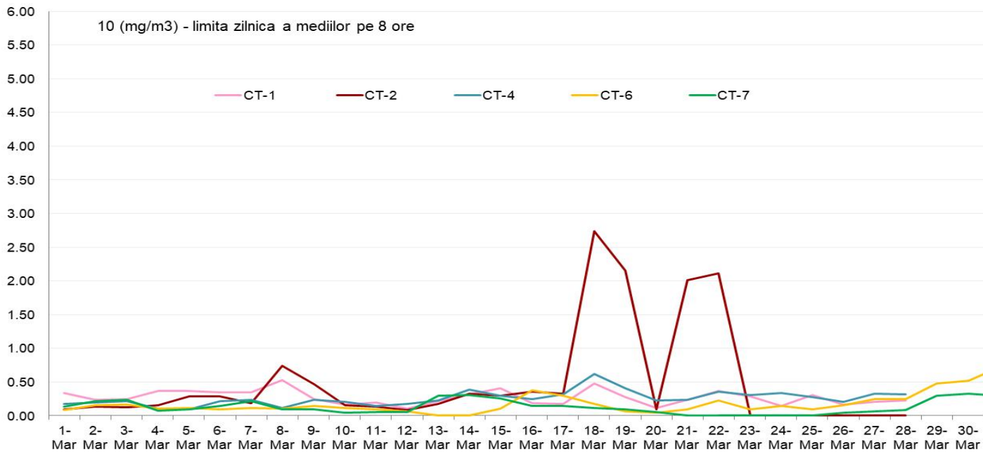
CO (mg/m3) - maximul zilnic medie mobila perioada: 01 Martie - 31 Martie 2019 - date validate
