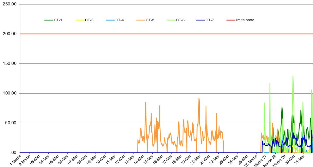
NO2 (ug/m3), perioada: 01 Martie 2019-31 Martie 2019 - Date validate
