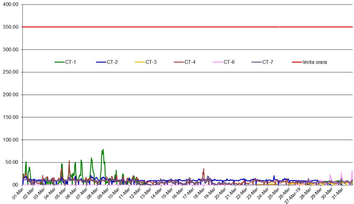
SO2 (ug/m3), perioada: 01 Martie 2019 - 31 Martie 2019 - Date validate
