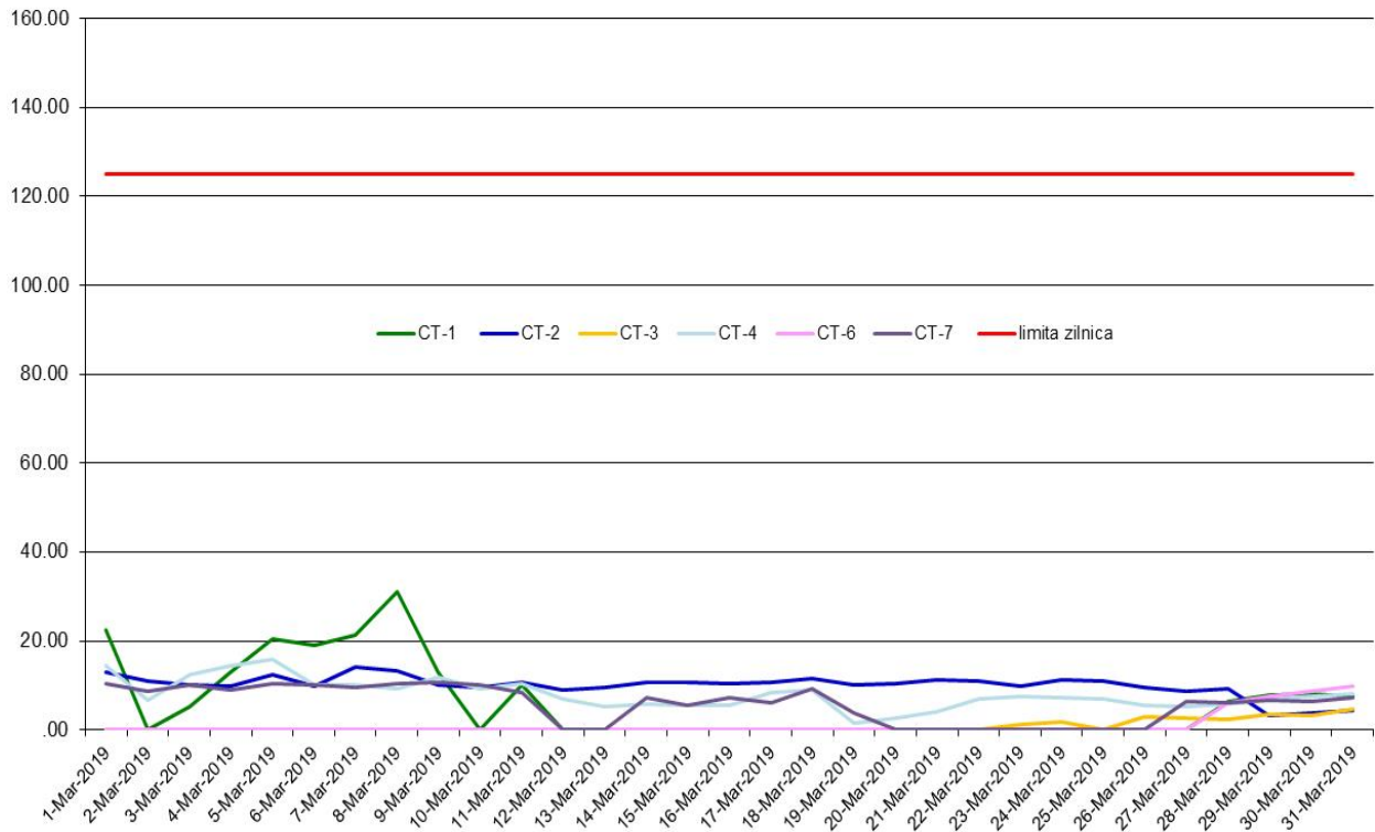
SO2 (ug/m3), perioada: 01 - 31 Martie 2019 - Date validate
