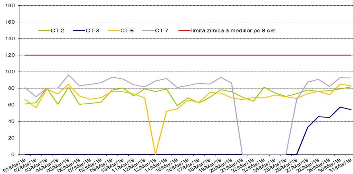
O 3 (mg/m 3 ) - maximul zilnic medie mobila perioada: 01 Martie - 31 Martie 2019 - date validate
