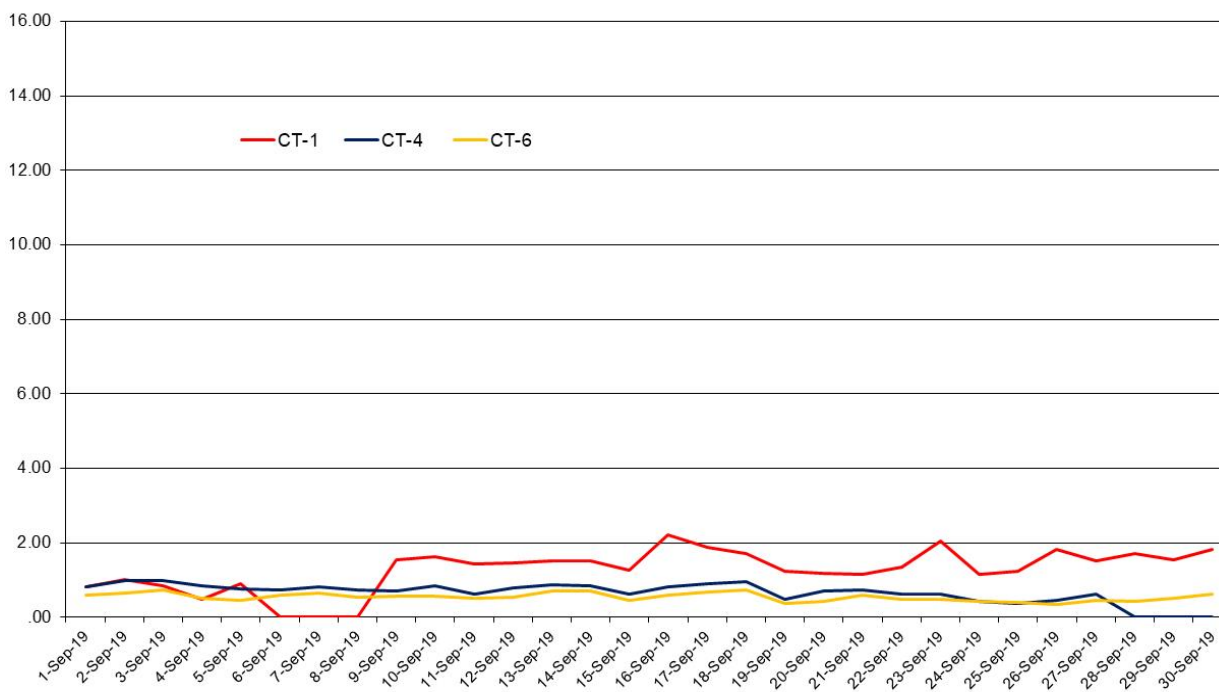
Benzen ( \mu\text{g}/\text{m}^3 ), perioada: 01 - 30 Septembrie 2019 - Date validate
