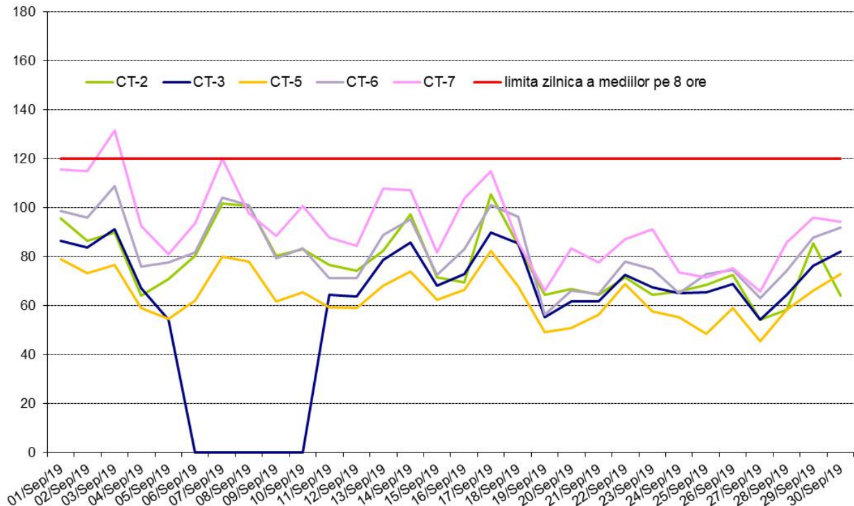
O 3 (mg/m 3 ) - maximul zilnic medie mobila perioada: 01 Septembrie - 30 Septembrie 2019 - date validate
