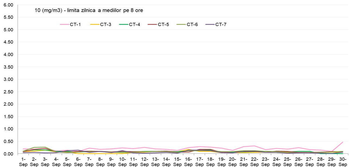
CO (mg/m3) - maximul zilnic medie mobila perioada: 01 Septembrie - 30 Septembrie 2019 - date validate
