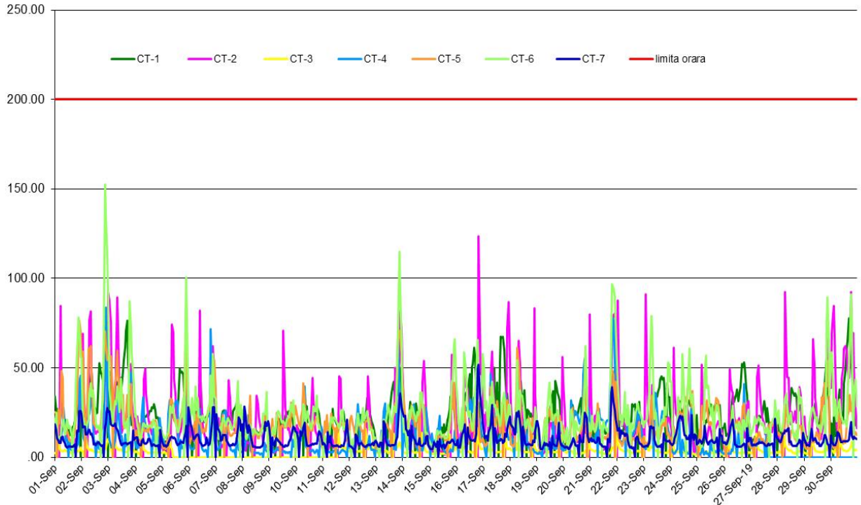
NO2 (ug/m3), perioada: 01 Septembrie 2019 - 30 Septembrie 2019 - Date validate
