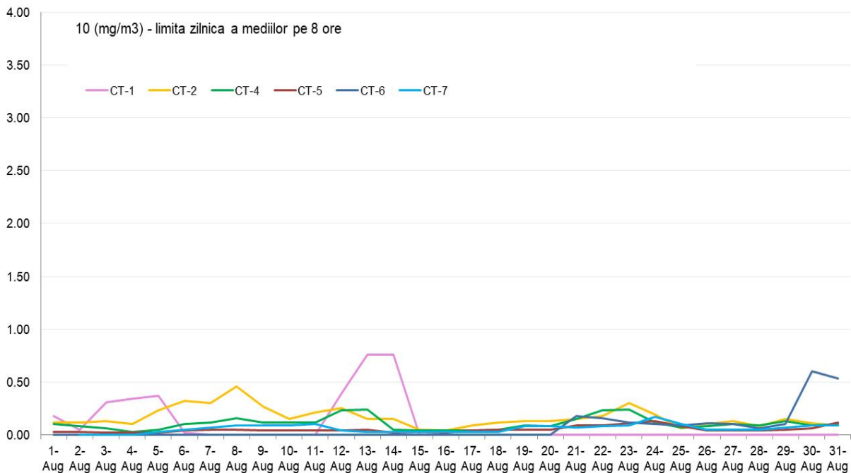
CO (mg/m3) - maximul zilnic medie mobila perioada: 01 - 31 August 2020 - date validate
