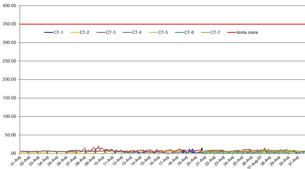
SO2 (ug/m3), perioada: 01 - 31 August 2020 - Date validate
