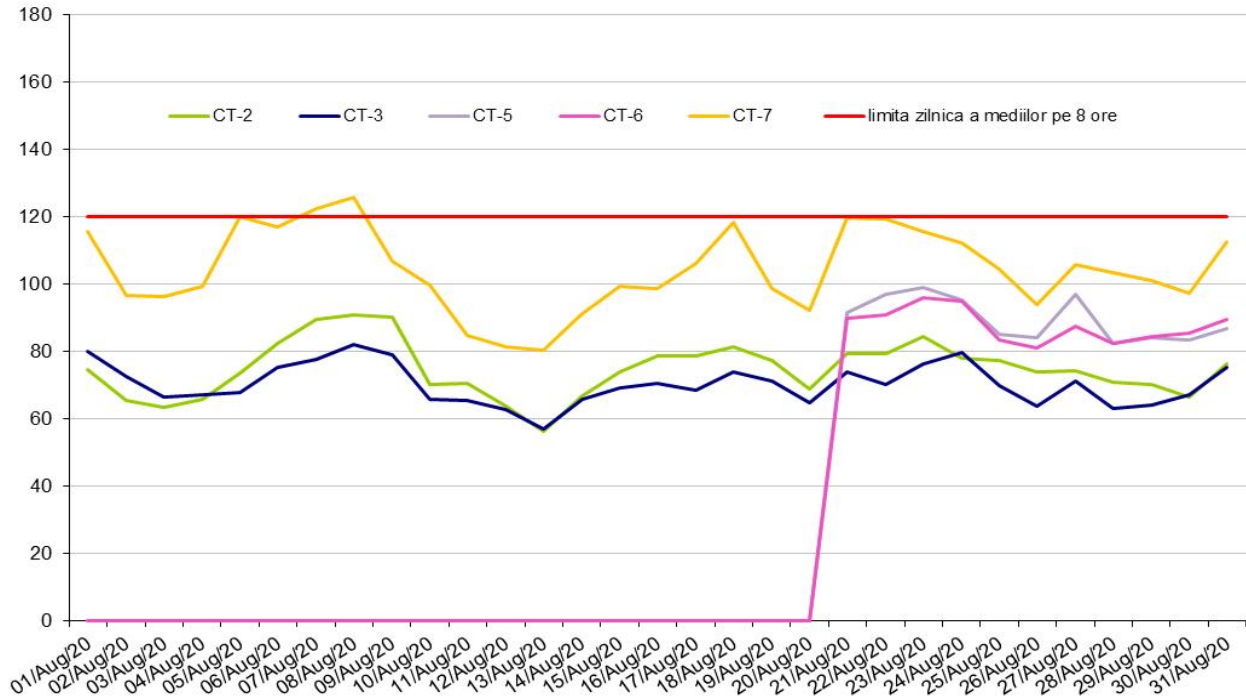
O 3 (mg/m 3 ) - maximul zilnic medie mobila perioada: 01 - 31 August 2020 - date validate
