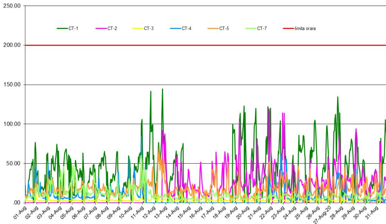
NO2 (ug/m3), perioada: 01 - 31 August 2020 - Date validate
