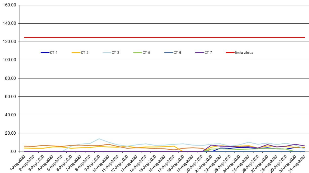
SO2 (ug/m3), perioada: 01 - 31 August 2020 - Date validate
