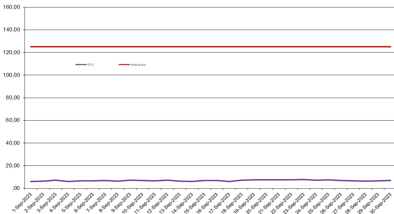
SO 2 (ug/m 3 ), perioada: 01 - 30 Septembrie 2023 - Date validate
