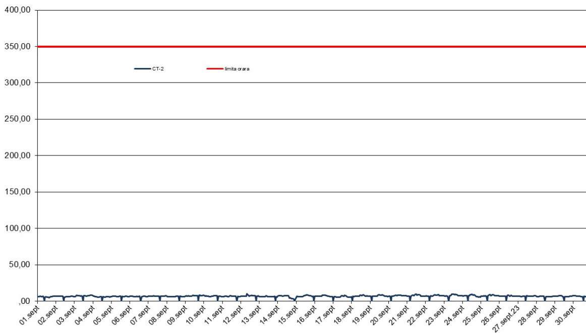
SO 2 (ug/m 3 ), perioada: 01 - 30 Septembrie 2023 - Date validate
