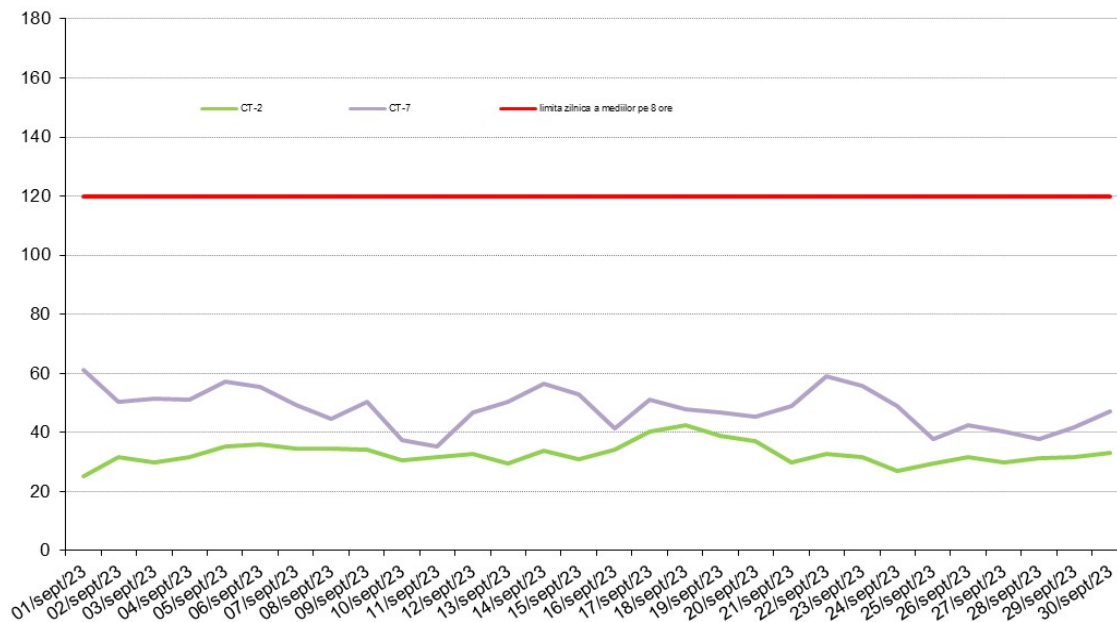
O3 (mg/m3) - maximul zilnic medie mobila perioada: 01 - 30 Septembrie 2023 - date validate
