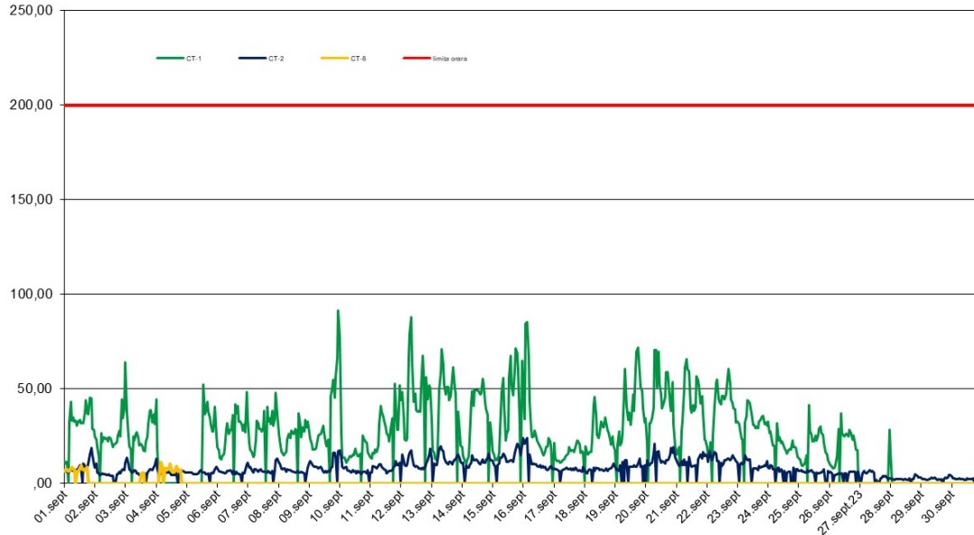
NO2 (ug/m3), perioada: 01 - 30 Septembrie 2023 - Date validate
