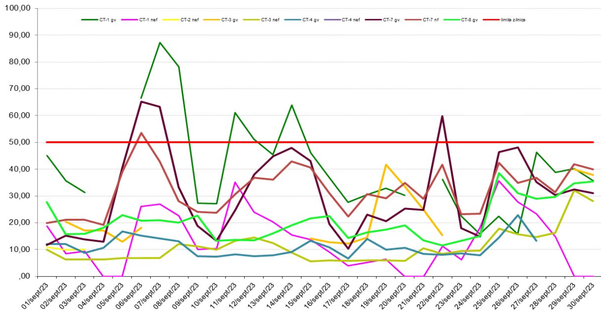
PM10 nef și PM10 gv ( \mu\text{g}/\text{m}^3 ), perioada: 01 - 30 Septembrie 2023 - Date validate
