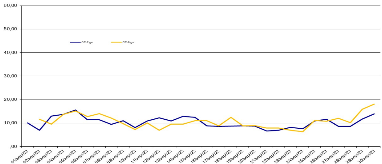
PM2.5 gv ( \mu\text{g}/\text{m}^3 ), perioada: 01 - 30 Septembrie 2023 - Date validate
