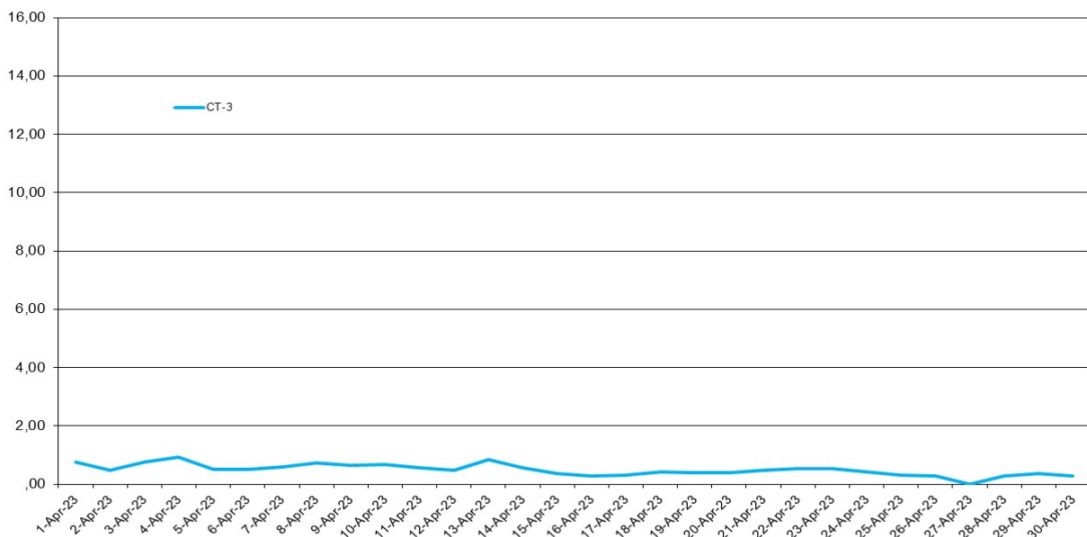
Benzen (ug/m3), perioada: 01 - 30 Aprilie 2023 - Date validate
