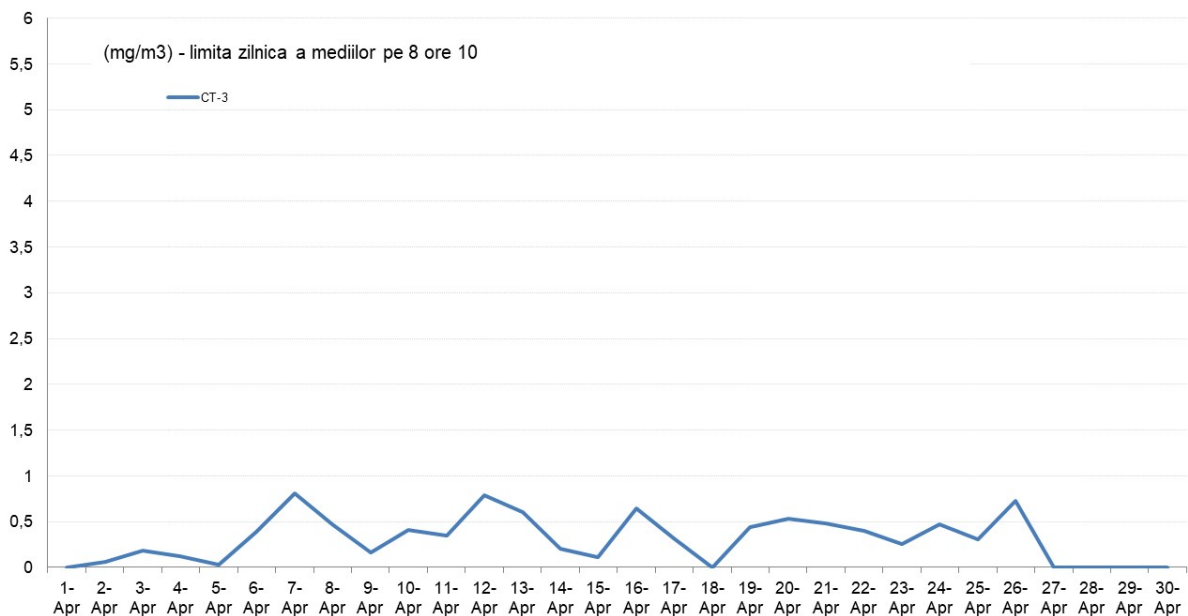
CO (mg/m3) - maximul zilnic medie mobila perioada: 01 - 30 Aprilie 2023 - date validate
