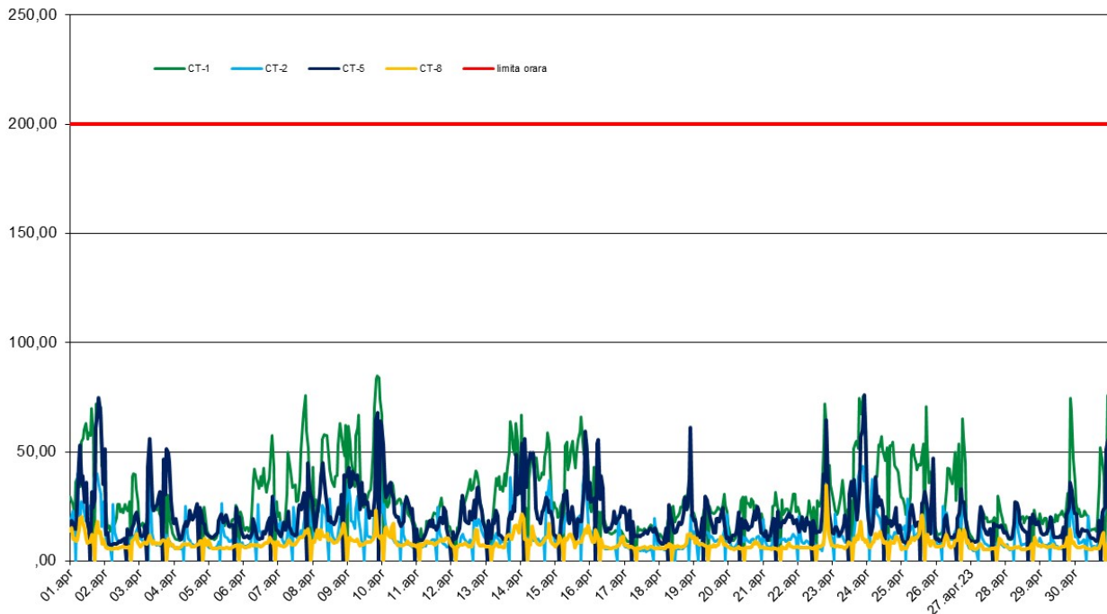
NO 2 (ug/m3), perioada: 01 - 30 Aprilie 2023 - Date validate
