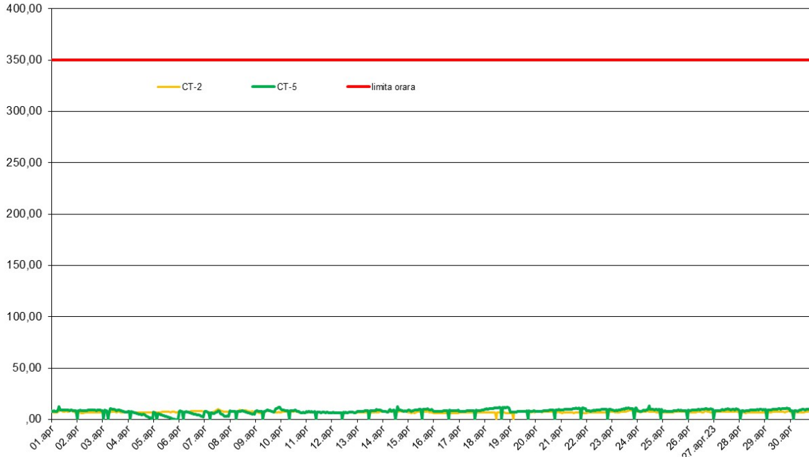
SO2 (ug/m3), perioada: 01 - 30 Aprilie 2023 - Date validate
