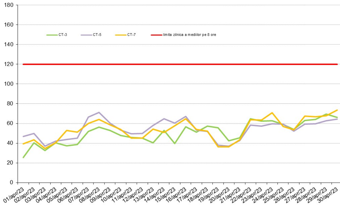
O 3 (mg/m 3 ) - maximul zilnic medie mobila perioada: 01 - 30 Aprilie 2023 - date validate
