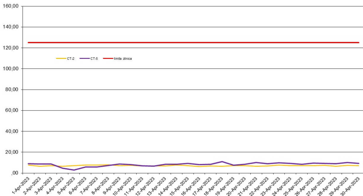
SO2 (ug/m3), perioada: 01 - 30 Aprilie 2023 - Date validate
