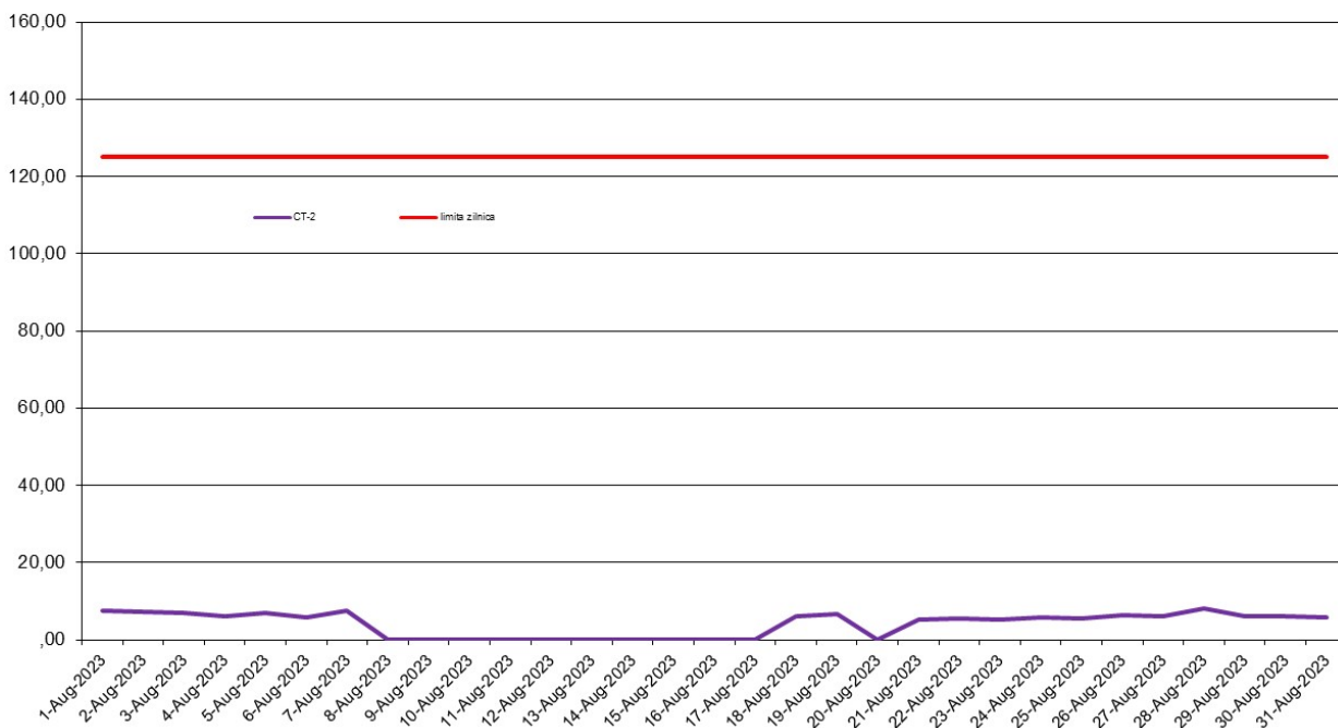
SO2 (ug/m3), perioada: 01 - 31 August 2023 - Date validate
