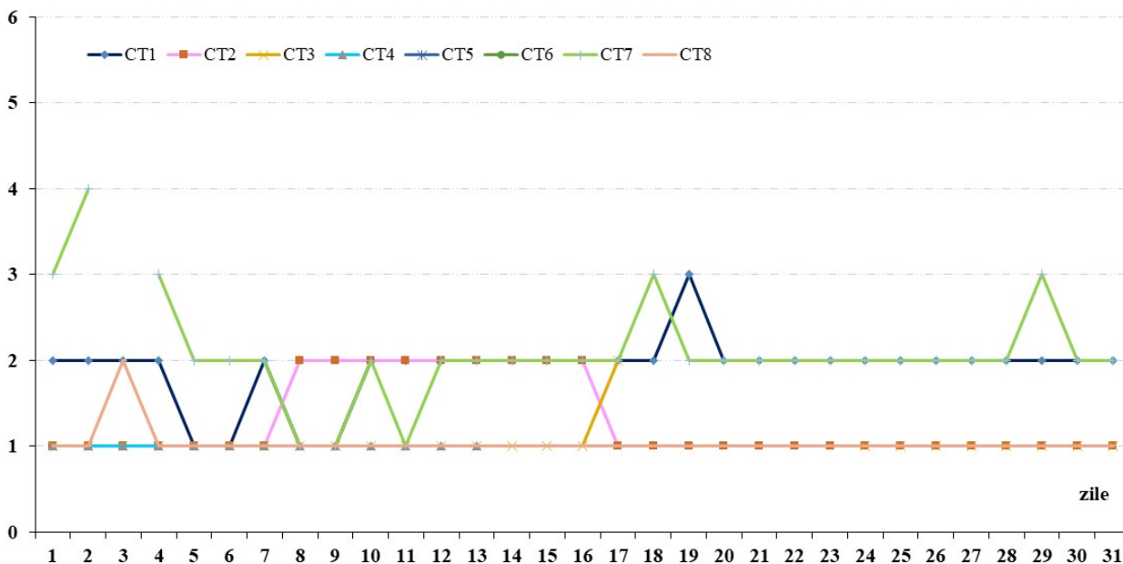
Indici generali - august 2023
