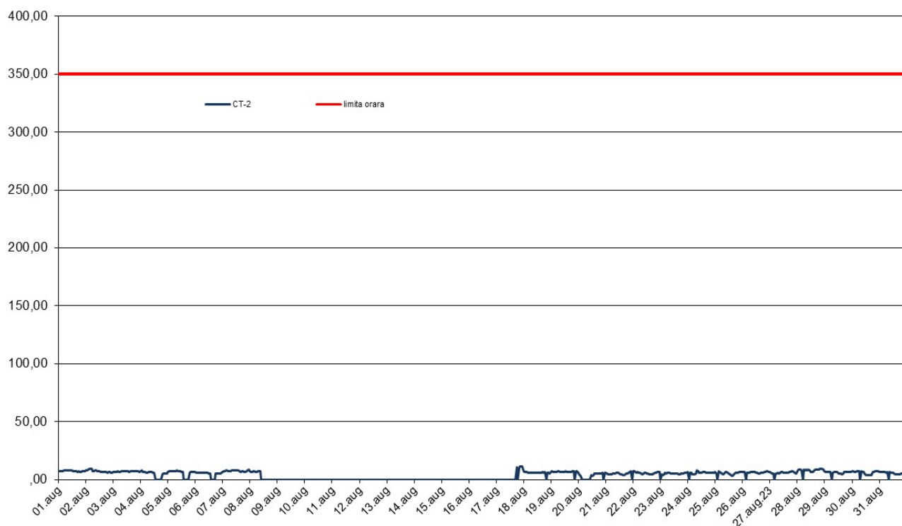
SO2 (ug/m3), perioada: 01 - 31 August 2023 - Date validate
