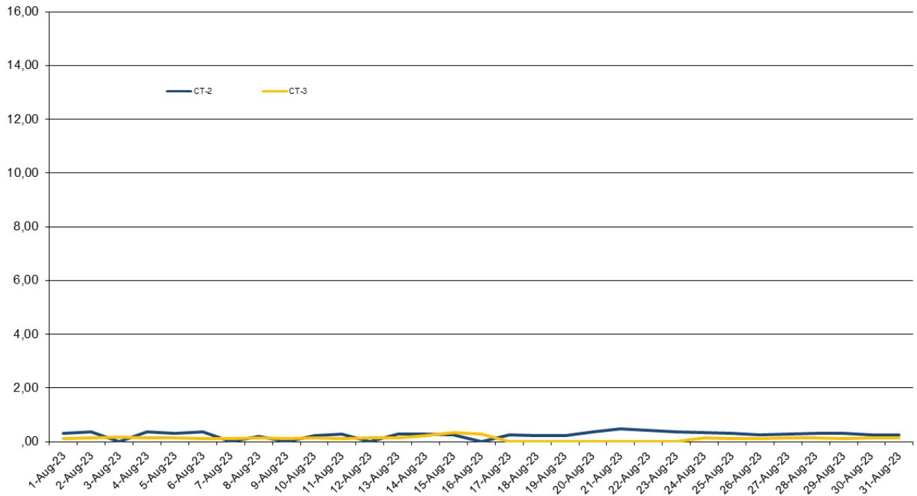
Benzen (ug/m3), perioada: 01 - 31 August 2023 - Date validate
