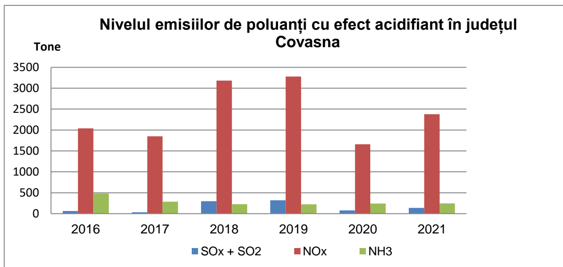
Figura 1.2.1.1.4. Nivelul emisiilor de poluanți cu efect acidifiant în județul Covasna
