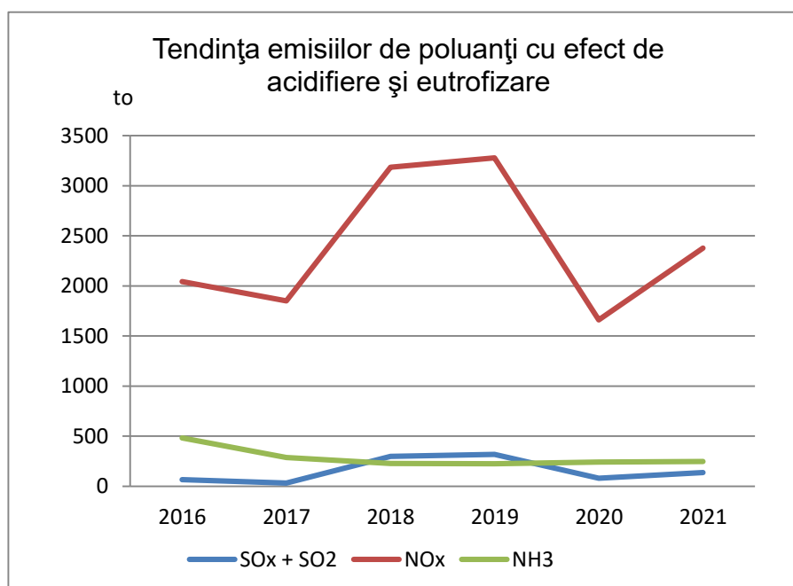
Figura nr. 1.3.1.1. Tendința emisiilor de poluanți cu efect de acidifiere
