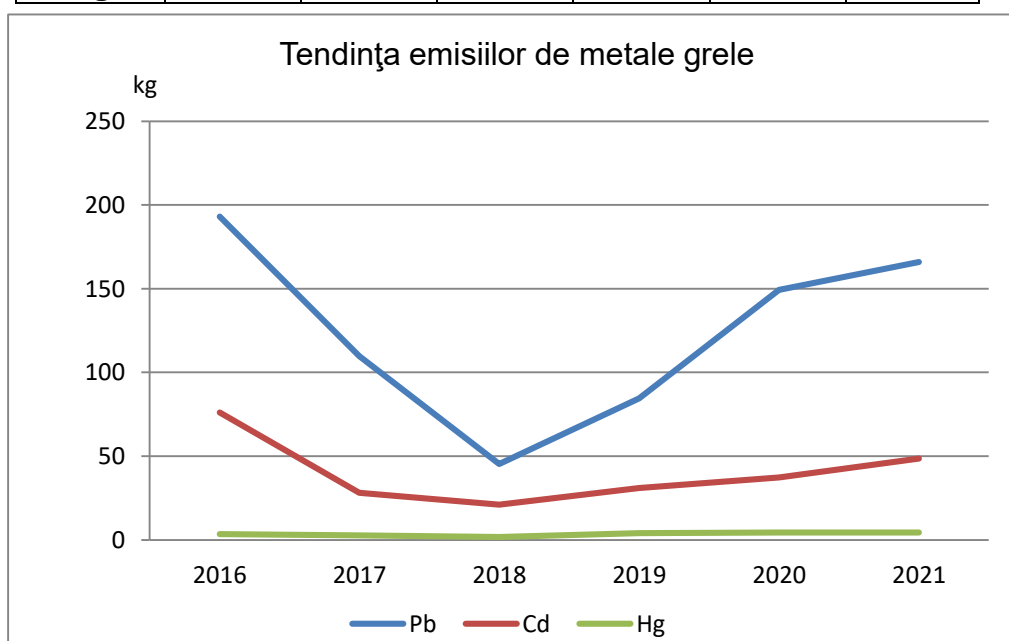
Figura 1.3.1.5. Tendența emisiilor de metale grele
