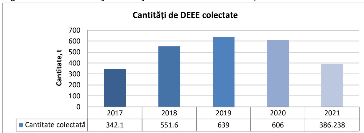
Figura VII.1.3.1.1 Evoluția cantităților de DEEE colectate în perioada 2017-2021
