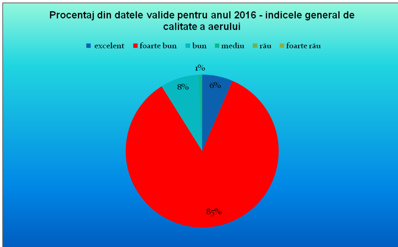
Figura 4.2 Calitatea aerului reflectată prin indici în anul 2016
