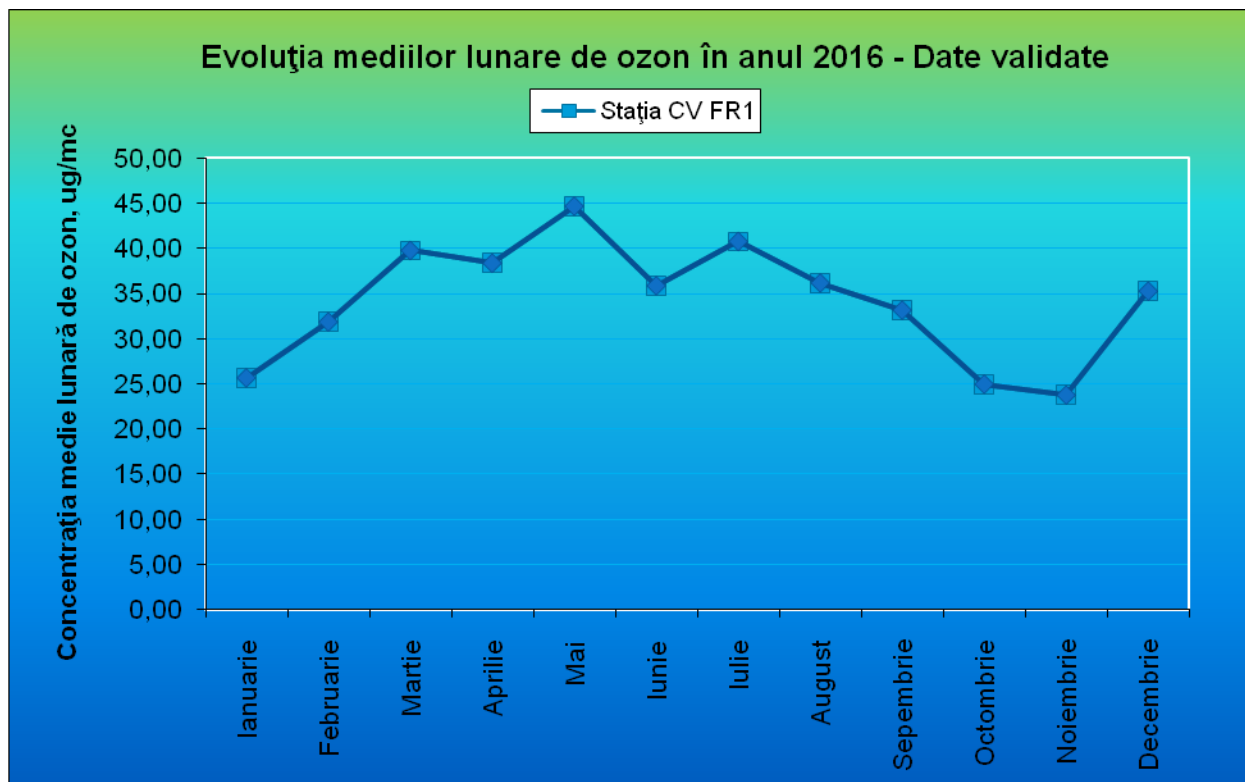
Figura 3.4.3.1 Evoluția mediilor lunare de \text{O}_3 în anul 2016
