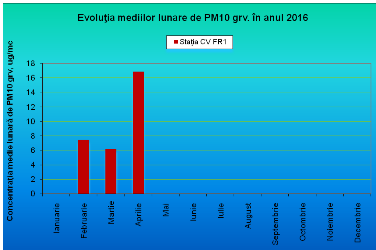
Figura 3.1.2.1 Evoluția mediilor lunare de PM 10 grv. în anul 2016
