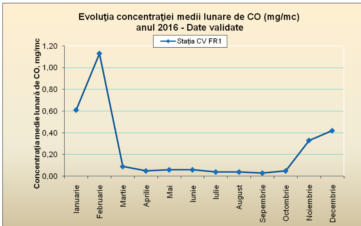
Figura 3.2.3.1 Evoluția mediilor lunare de CO, în anul 2016
