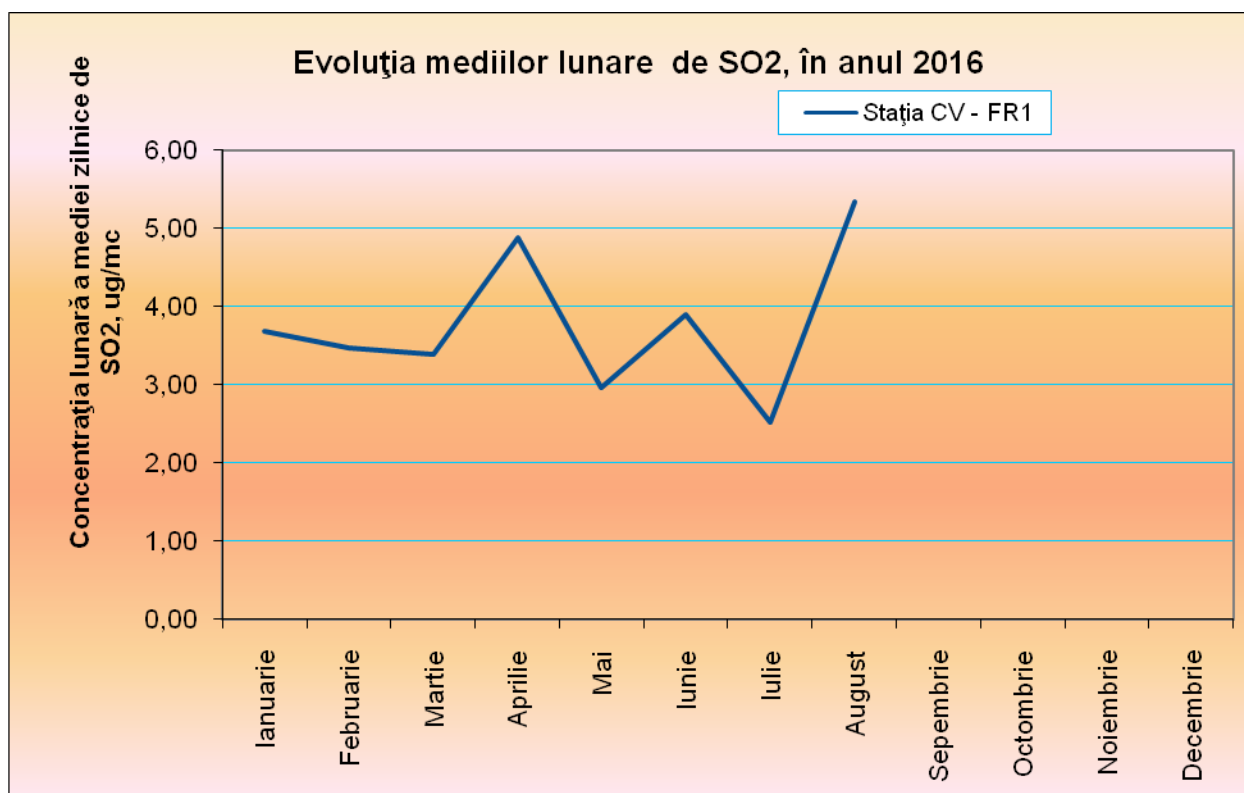
Figura 3.3.3.1 Evoluția mediilor lunare de SO 2 , în anul 2016
