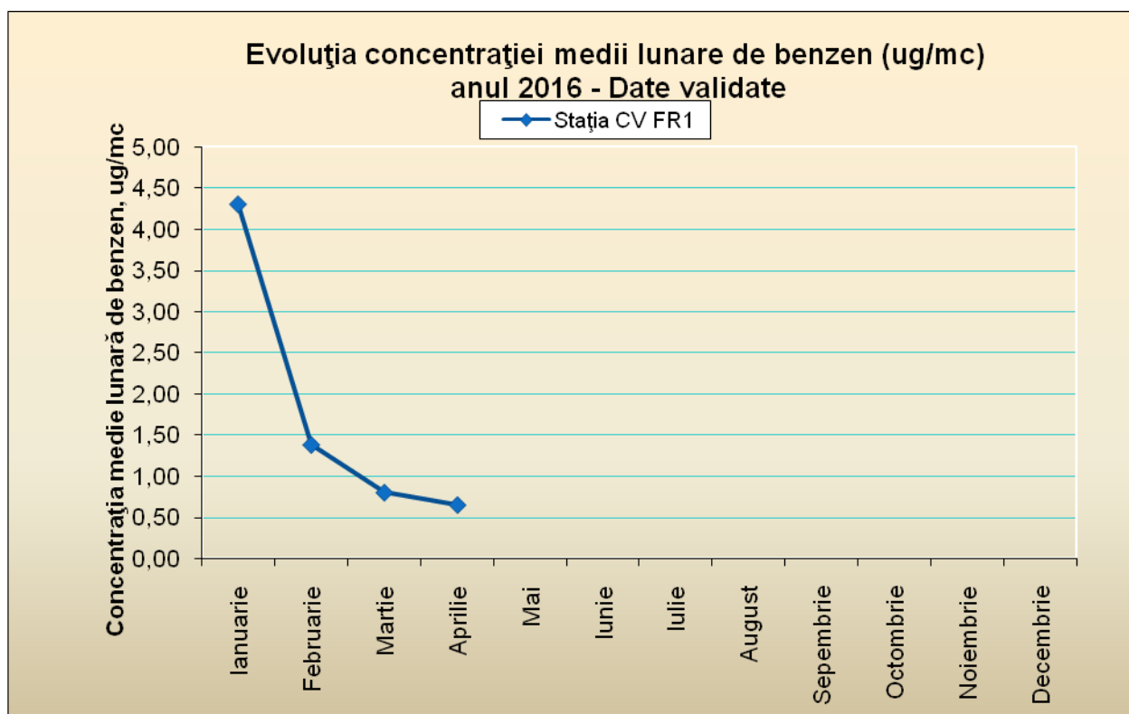
Figura 3.5.3.1 Evoluția mediilor lunare de benzen în anul 2016
