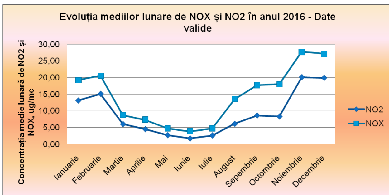
Figura 3.6.2.1 Evoluția mediilor lunare de \text{NO}_2 și \text{NOX} în anul 2016
