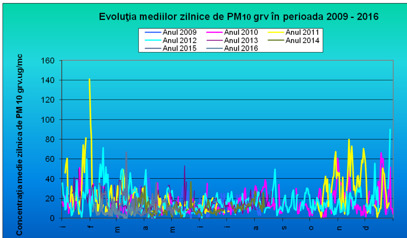
Figura 3.1.2.2 Evoluția mediilor zilnice de PM_{10} grv. în anii 2009 - 2016
