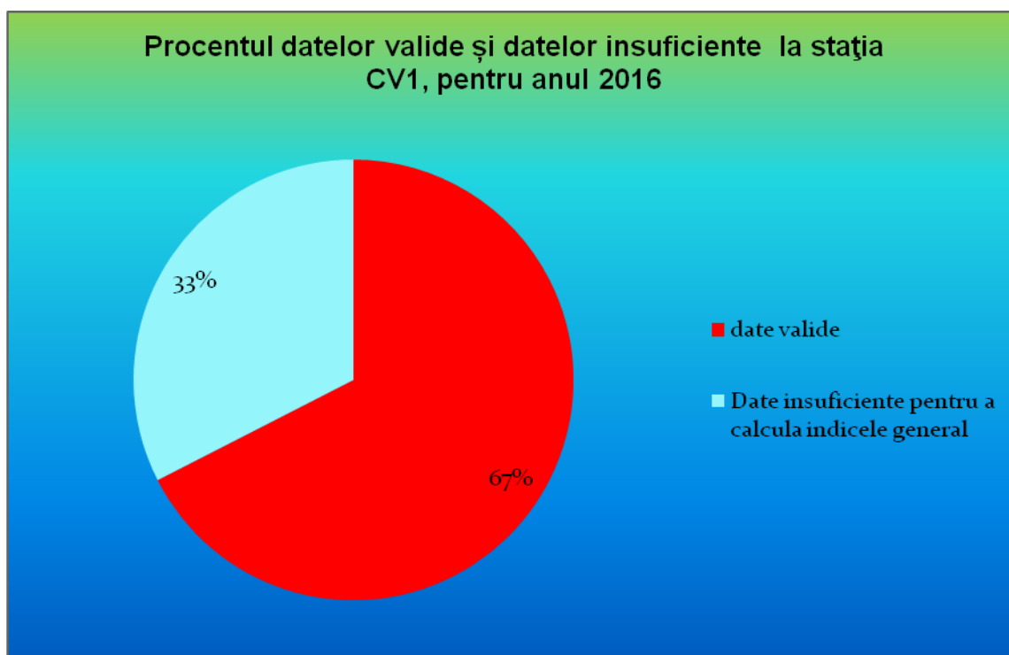
Figura 4.1 Procentul datelor valide în anul 2016
