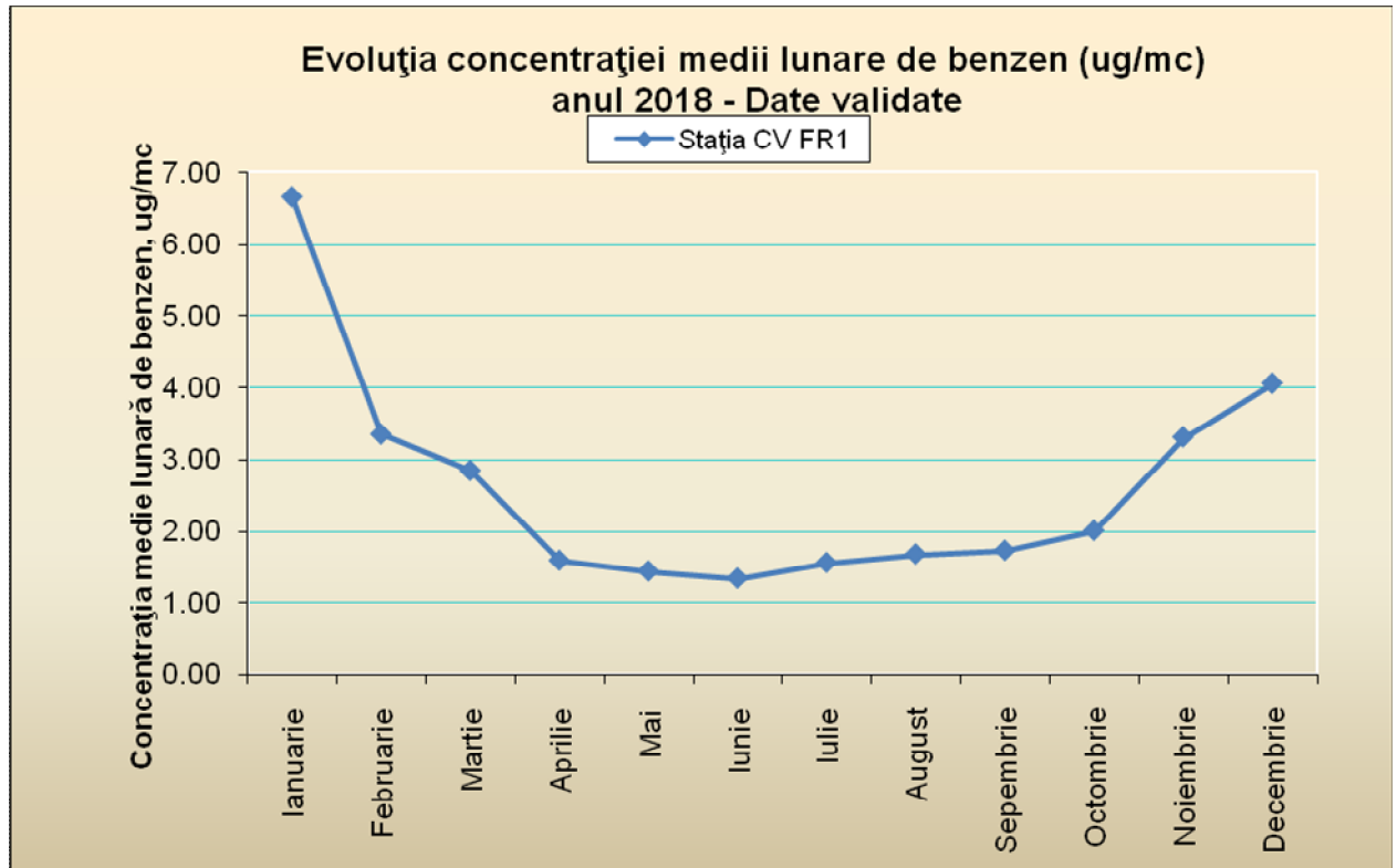
Figura 3.5.3.1 Evoluția mediilor lunare de benzen în anul 2018
