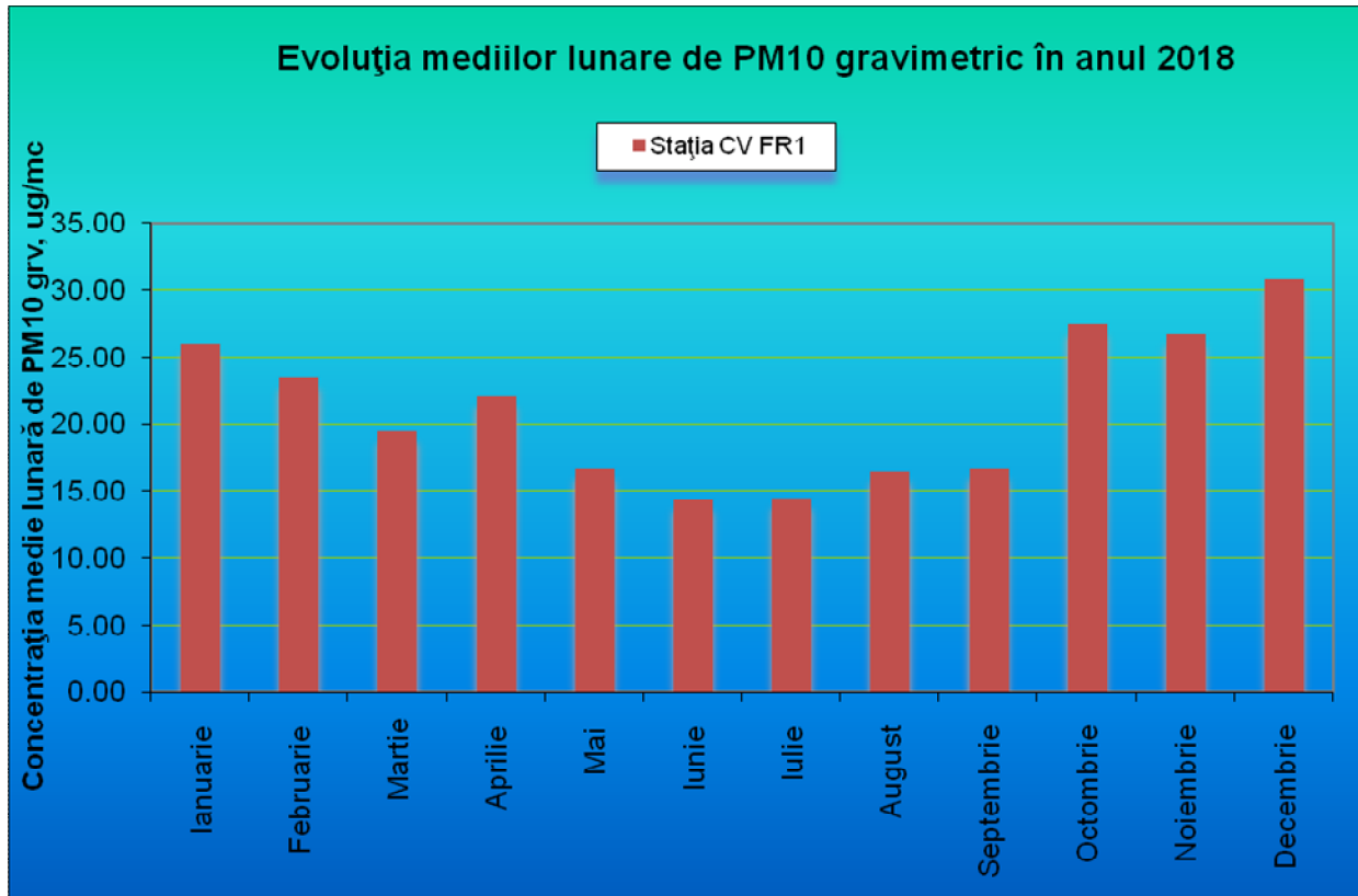
Figura 3.1.2.1 Evoluția mediilor lunare de PM 10 gravimetric în anul 2018
