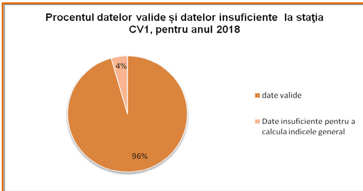
Figura 4.1 Procentul datelor valide în anul 2018
