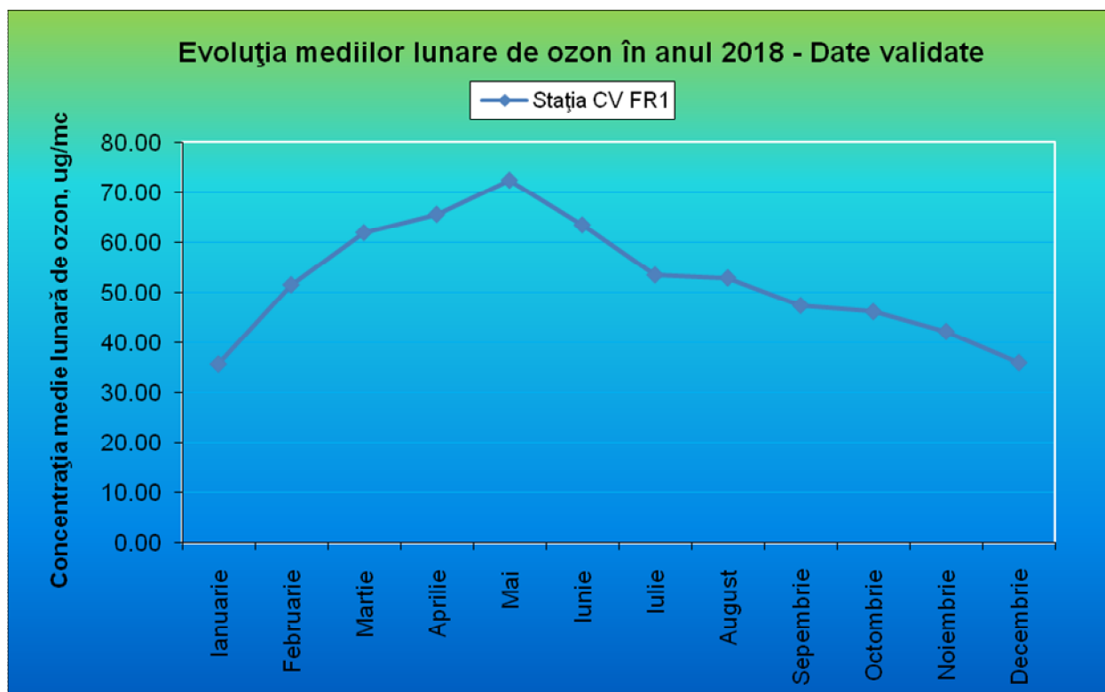
Figura 3.4.3.1 Evoluția mediilor lunare de O 3 în anul 2018
