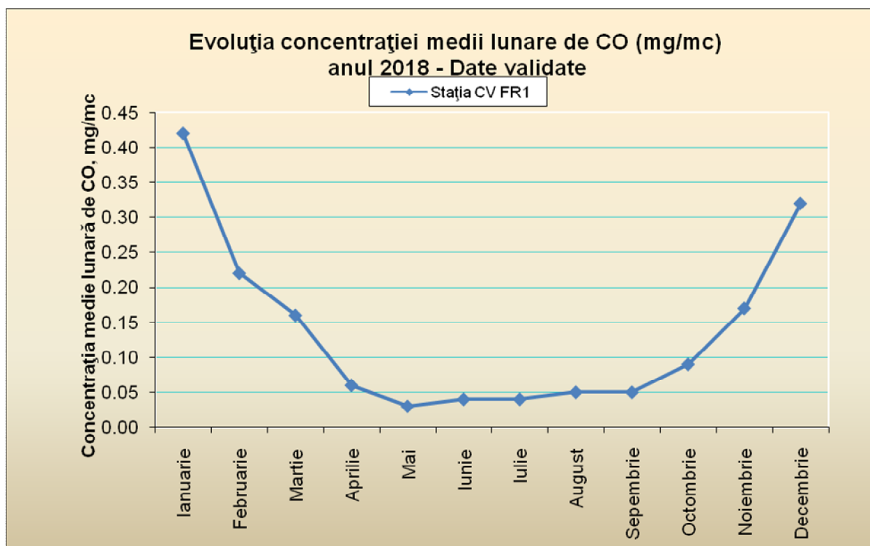
Figura 3.2.3.1 Evoluția mediilor lunare de CO, în anul 2018
