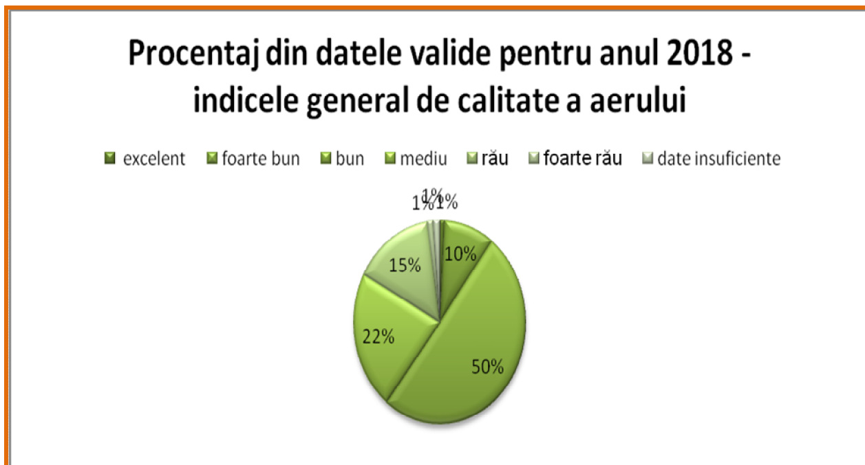
Figura 4.2 Calitatea aerului reflectată prin indici în anul 2018
