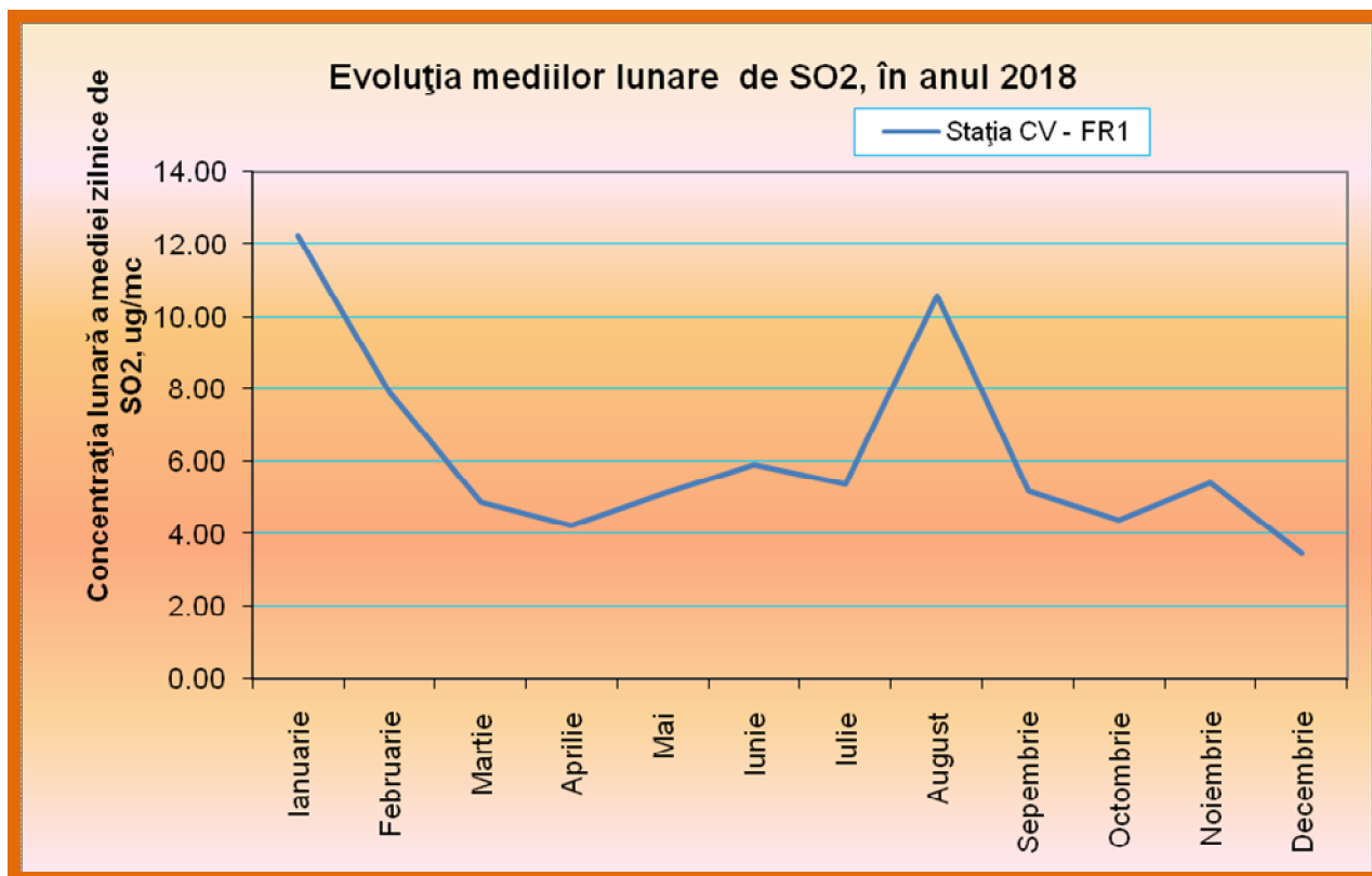
Figura 3.3.3.1 Evoluția mediilor lunare de SO 2 , în anul 2018
