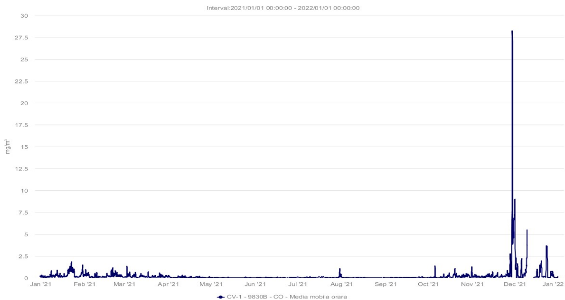
Figura 3.2.3.2 Evoluția mediei mobile de CO în anul 2021
