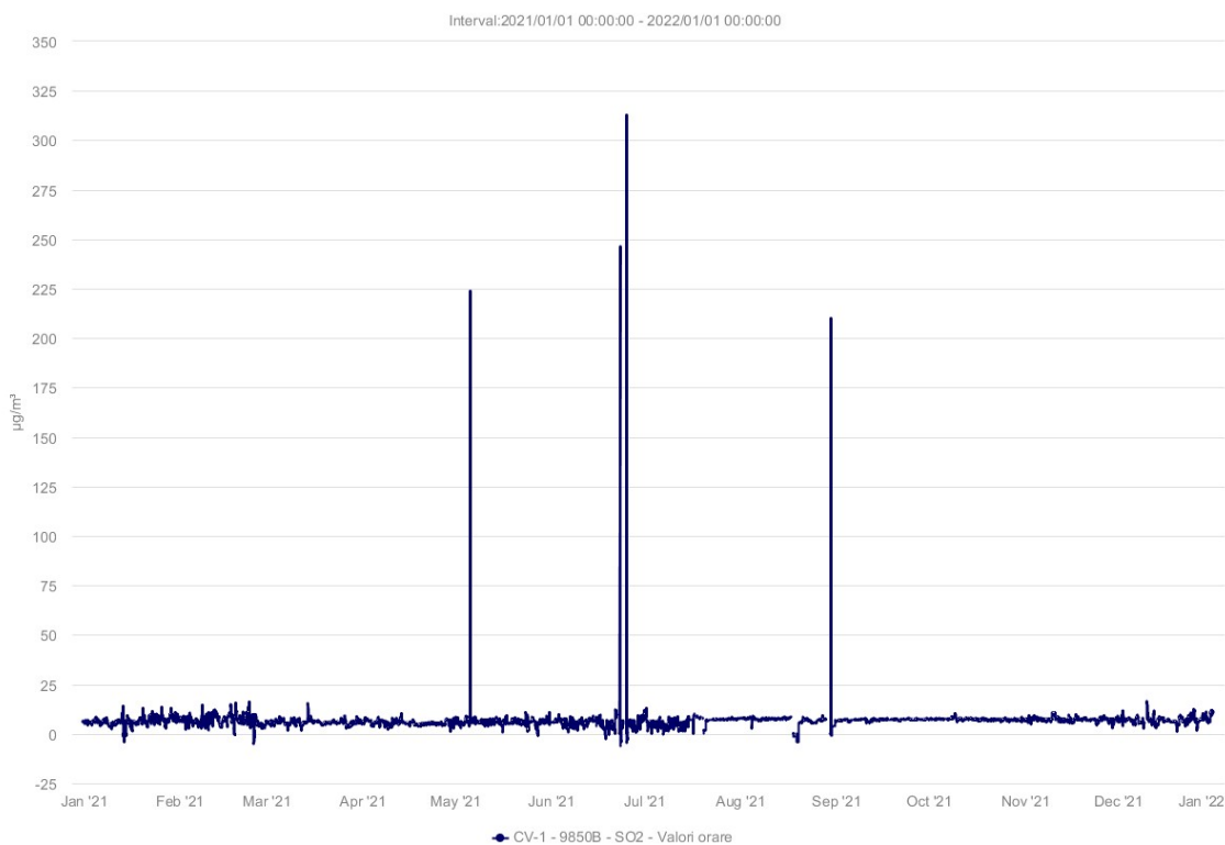
Figura 3.3.3.1 Evoluție valori orare SO 2 , în anul 2021
