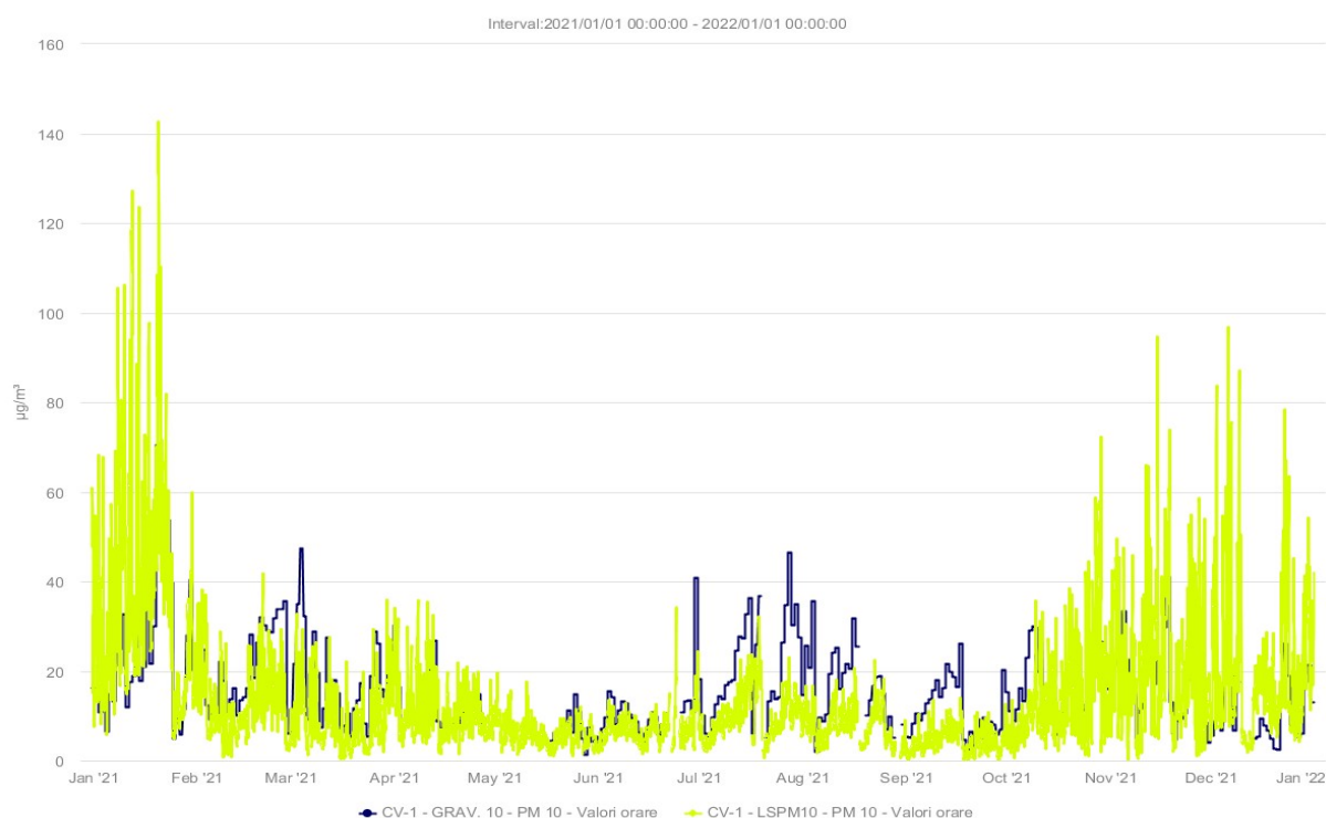
Figura 3.1.2.3 Evoluție valori PM 10 gravimetric și nefelometric în anul 2021-CV1
