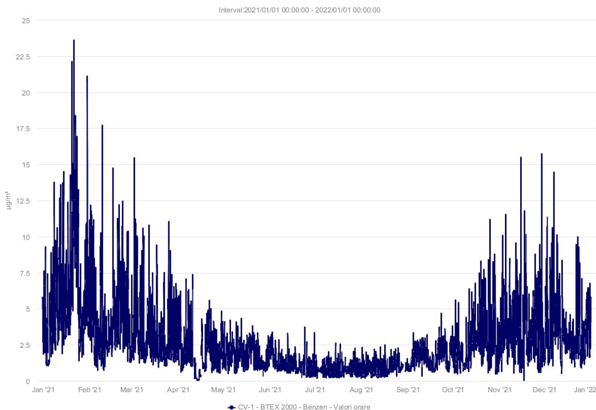
Figura 3.5.3.1 Evoluția valorilor de benzen în anul 2021
