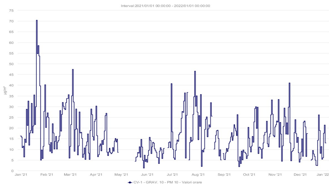
Figura 3.1.2.2 Evoluție valori PM 10 gravimetric în anul 2021-CV2
