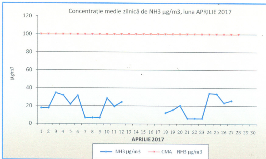
Figura 2. Evoluția concentrației medii zilnice de NH_3
