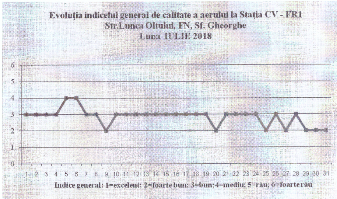
Figura 1.EVOLUTIA INDICELUI GENERAL DE CALITATE A AERULUI
