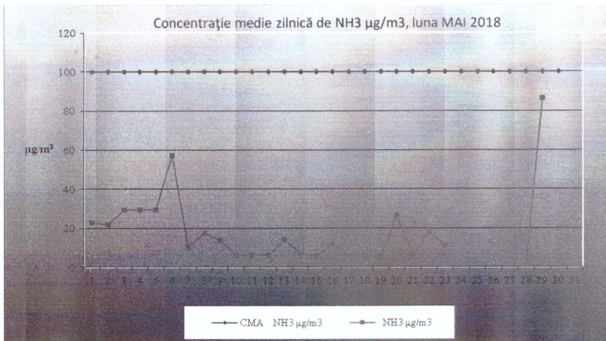
Figura 2. Evoluția concentrației medii zilnice de NH 3
