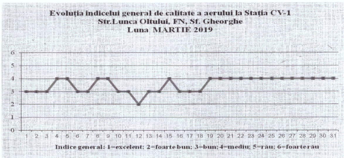
Figura 1.Evoluția indicelui general de calitate a aerului
