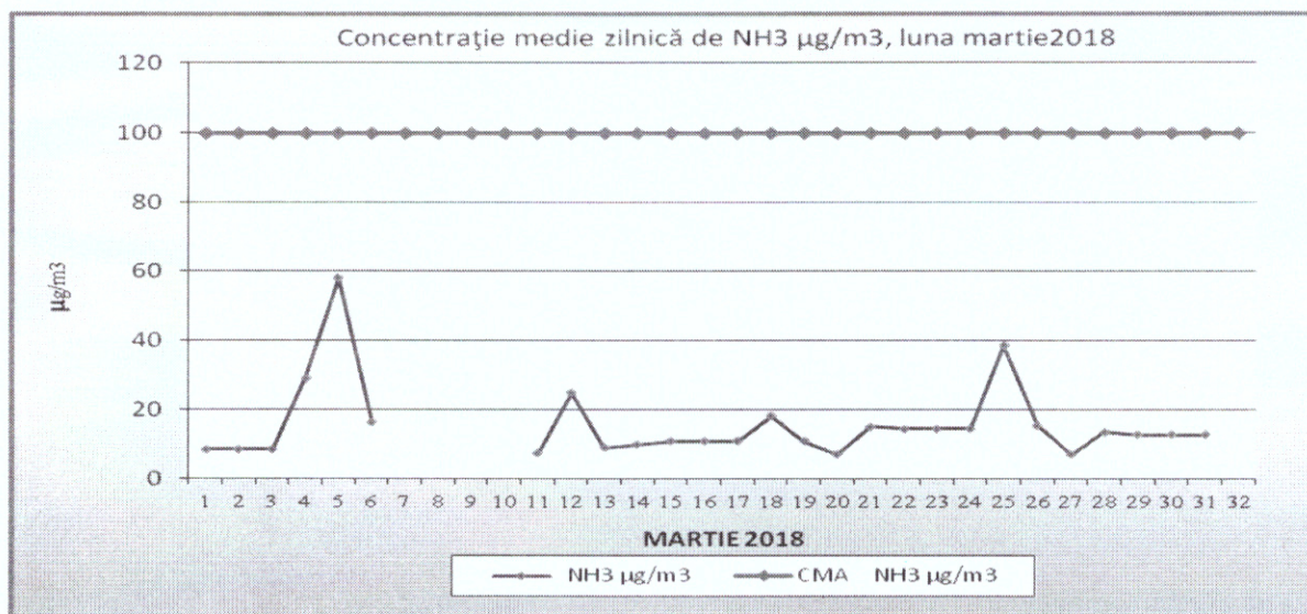
Figura 2. Evoluția concentrației medii zilnice de \text{NH}_3
