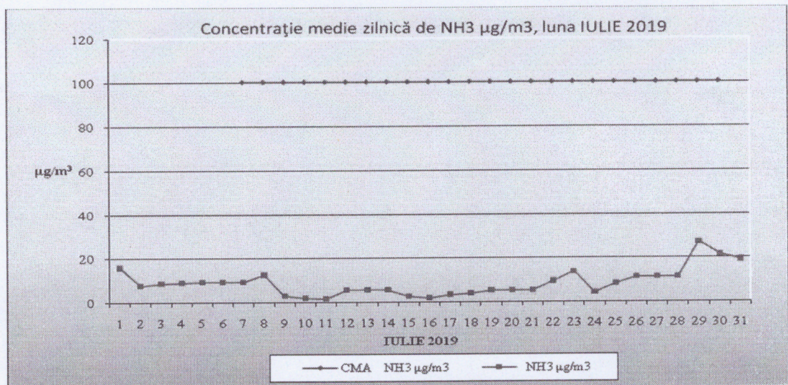
Figura 2. Evoluția concentrației medii zilnice de \text{NH}_3
