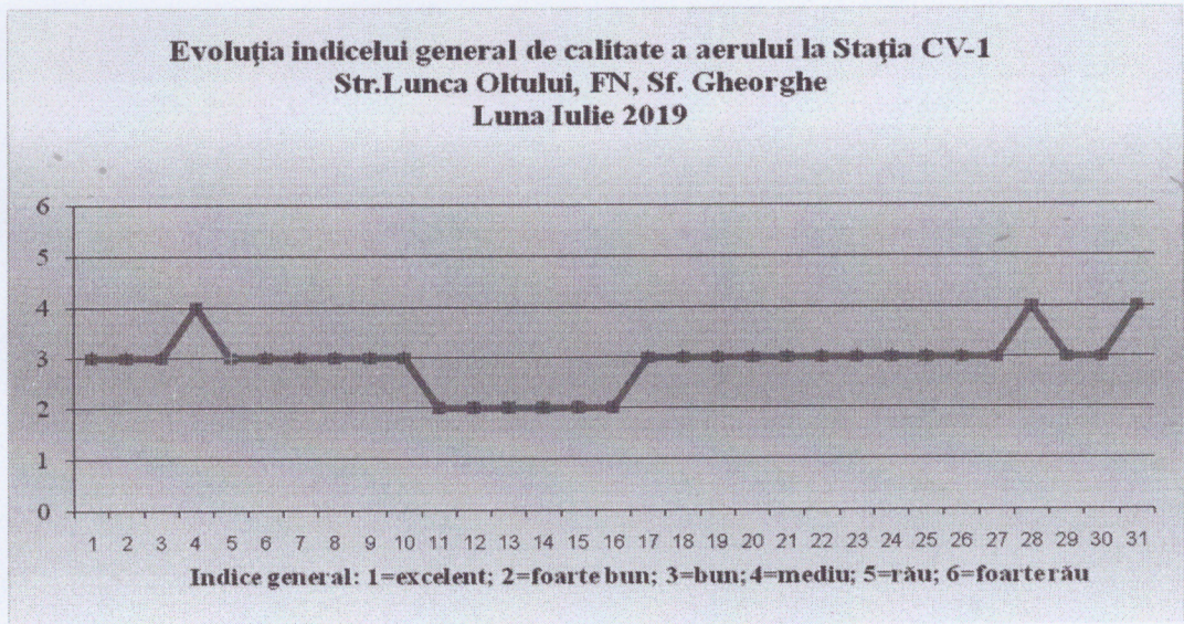
Figura 1. Evoluția indicelui general de calitate a aerului
