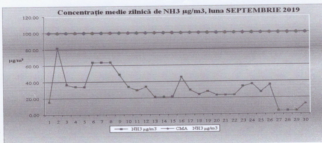
Figura 2. Evoluția concentrației medii zilnice de \text{NH}_3
